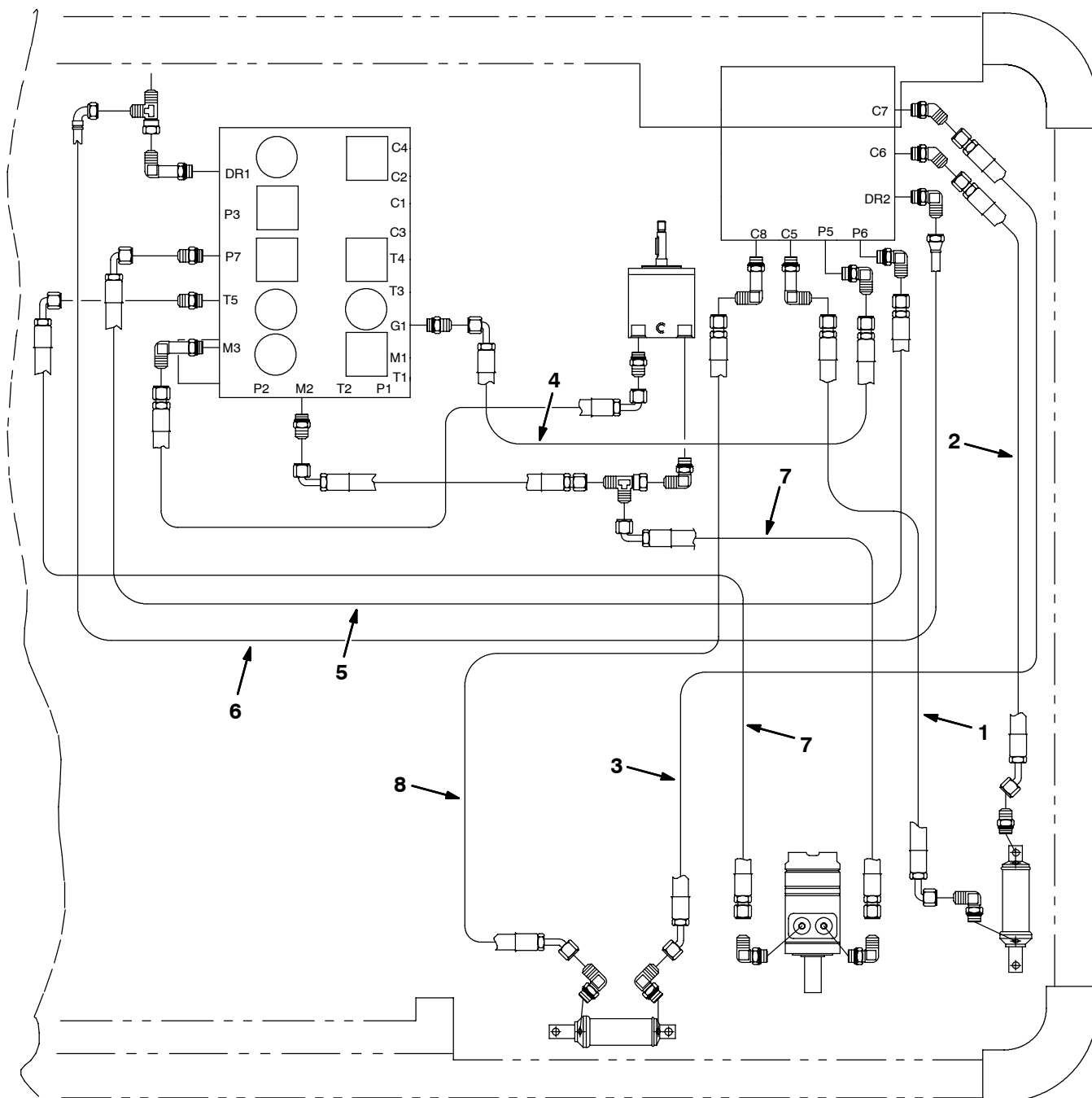
Fig. 64 - Side Brush Hydraulic Hose Group (740045 xxx- ) - Seitenbürsten-Hydraulikschlauch-Gruppe - Assemblage tuyaux hydrauliques de la brosse latérale
