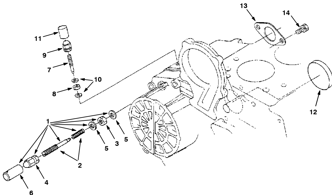
Fig. 18 - Idling Group - Leerlauf-Gruppe - Assemblage système de ralenti
