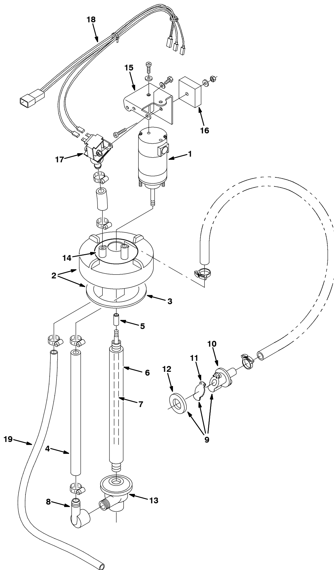
Fig. 19 - Extended Scrub Pump Breakdown, 20891 - Defekt Verlängerter Schrubbetrieb-Pumpe - Panne de pompe du système de nettoyage prolongé, 20891
