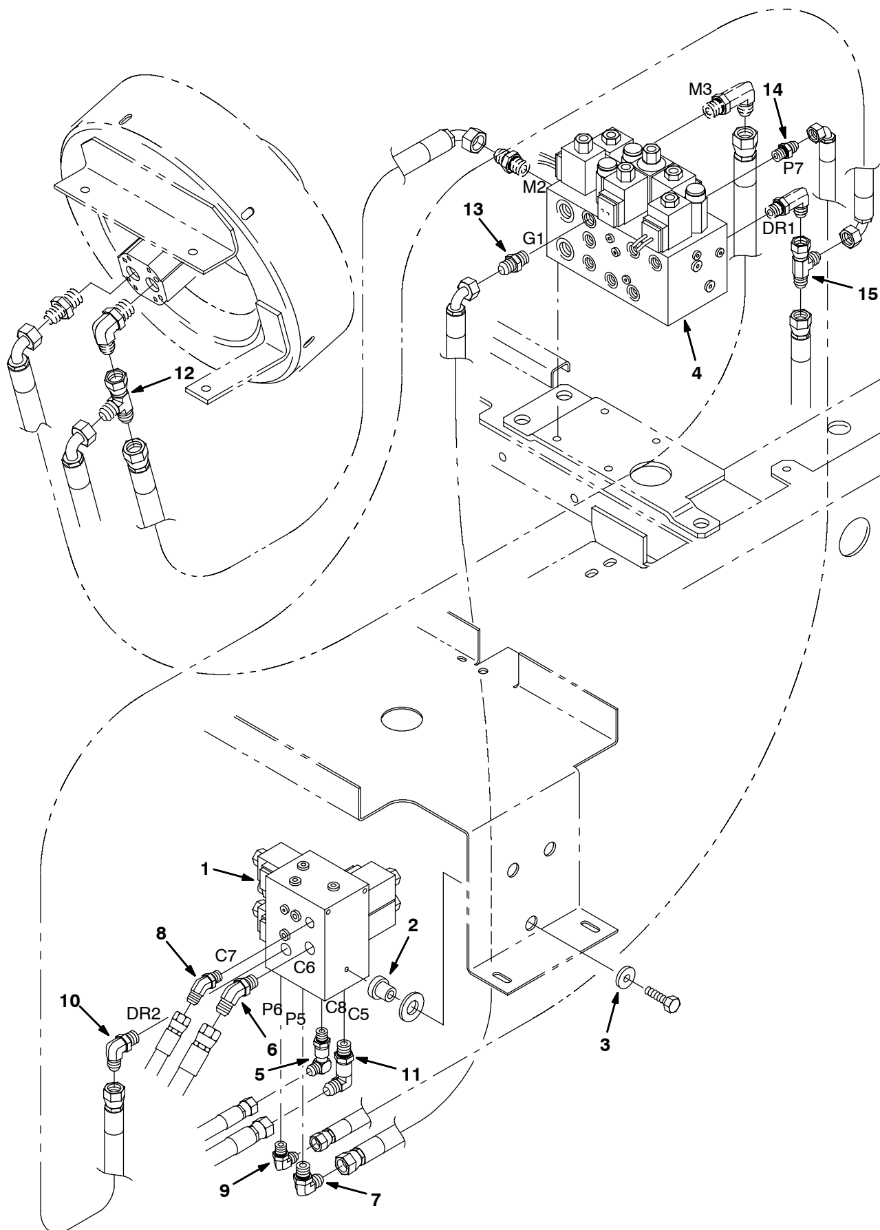
Fig. 62 - Side Brush Hydraulic Group (740045 xxx- ) - Seitenbürsten-Hydraulik-Gruppe - Assemblage système hydraulique de la brosse latérale
