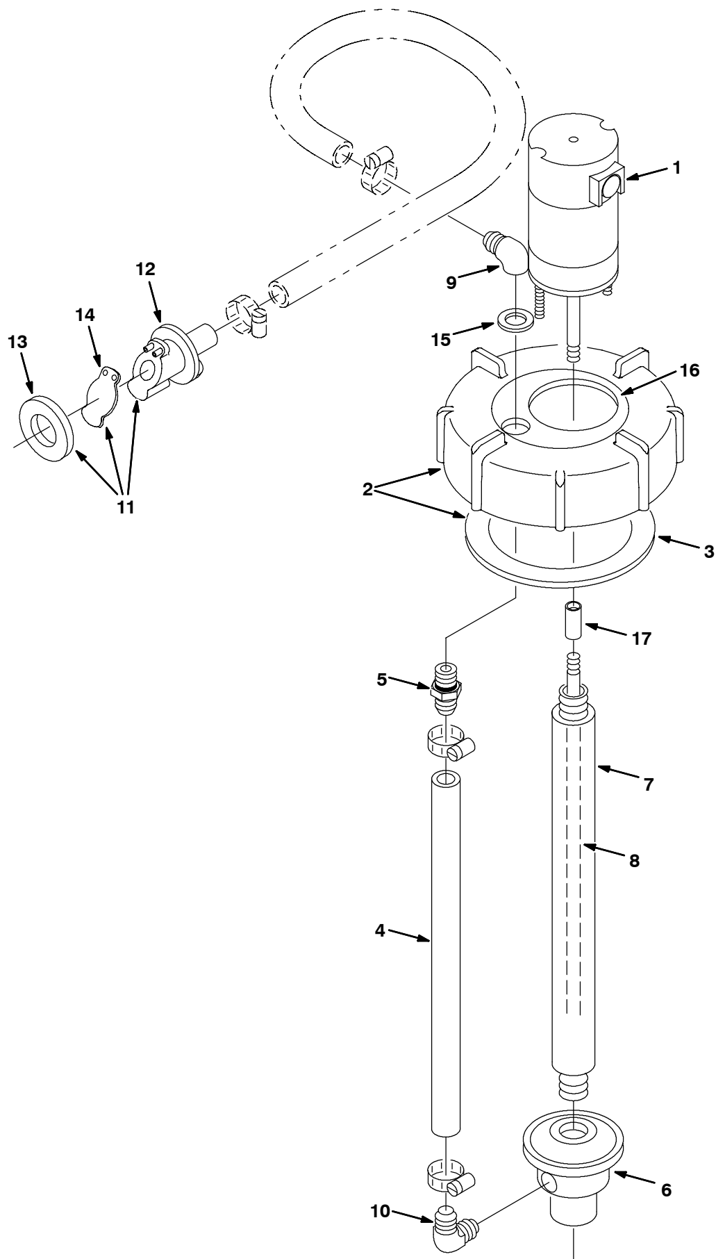
Fig. 20 - Extended Scrub Pump Breakdown, 1021210 - Defekt Verlängerter Schrubbetrieb-Pumpe - Panne de pompe du système de nettoyage prolongé, 1021210
