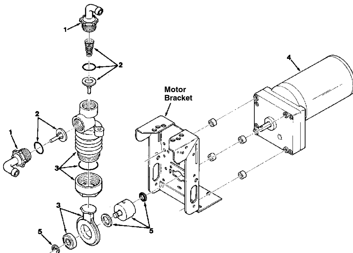
Fig. 22 - Metering Solution Pump Breakdown, 73260 - Schutzschalter für Firschwasser-Dosierungspumpe - Désamorcage de la pompe de dosage de solution
