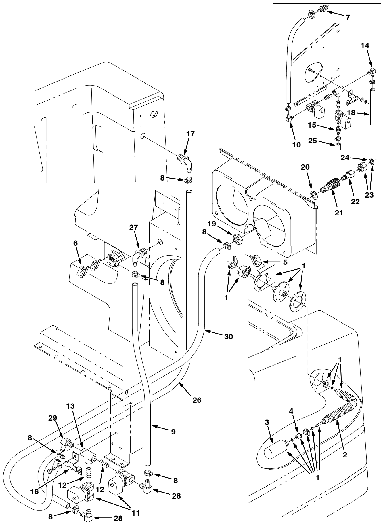
Fig. 55 - ES and Auto Fill Group - ES- und Einfüll-Automatik-Gruppe - Assemblage système ES et système de remplissage automatique
