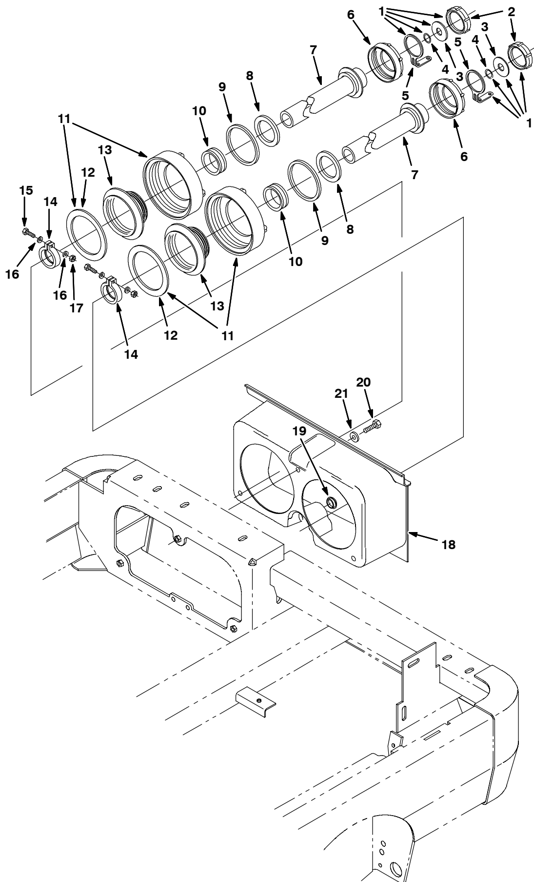
Fig. 31 - Solution and Recovery Tank Drain Group - Frischwasser-/Schmutzwasser-Tankentleerungsgruppe - Assemblage système de vidange du réservoir de solution et du réservoir de récupération
