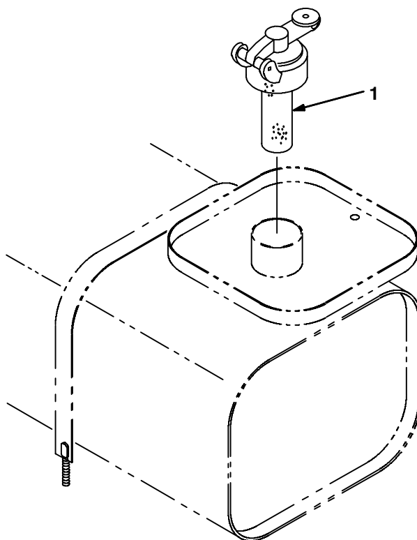
Fig. 7 - Protectoseal Fuel Tank Cap Group (7400 0001-7400 xxxx) - Protectoseal-Kraftstofftankverschluß-Gruppe - Assemblage couvercle du réservoir de carburant à joint protecto
