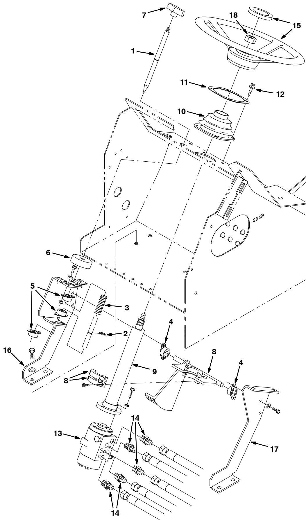
Fig. 9 - Steering Group - Lenkungsgruppe - Assemblage direction
