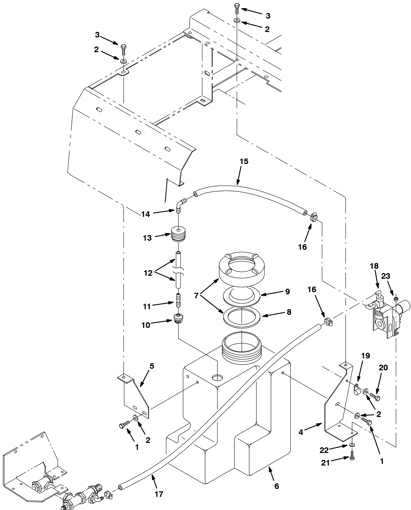
Fig. 58 - ES Detergent Tank Group - ES-Reinigungsmitteltank-Gruppe - Assemblage réservoir de détergent ES
