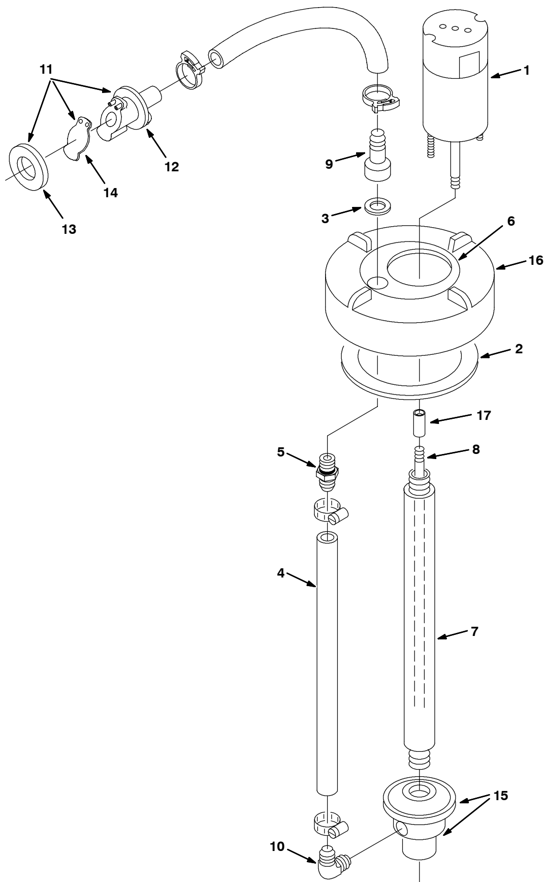
Fig. 17 - Extended Scrub Pump Breakdown, 20914 - Defekt Verlängerter Schrubbetrieb-Pumpe - Panne de pompe du système de nettoyage prolongé, 20914
