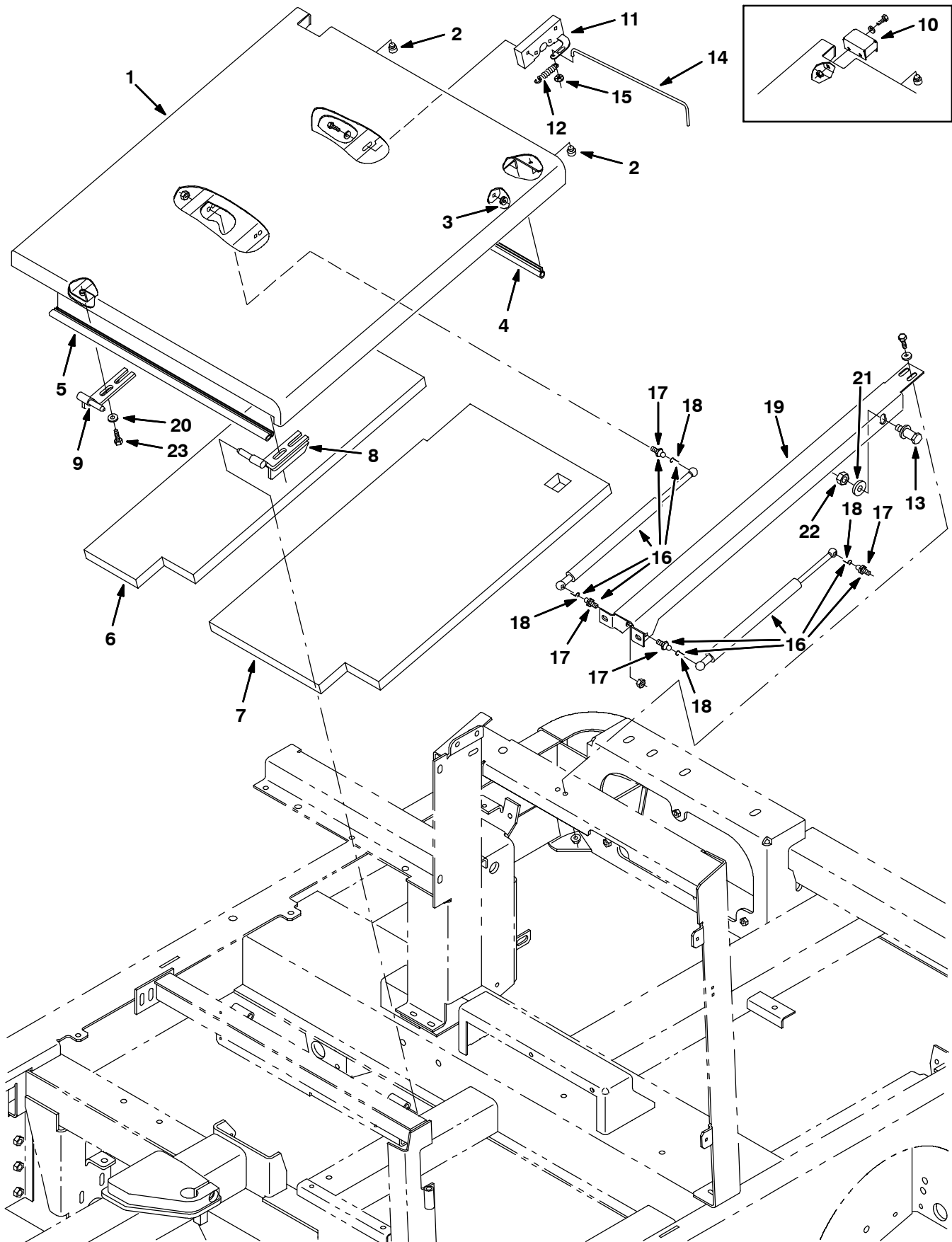
Fig. 8 - Engine Cover Group - Motorhauben-Gruppe - Assemblage couvercle du moteur
