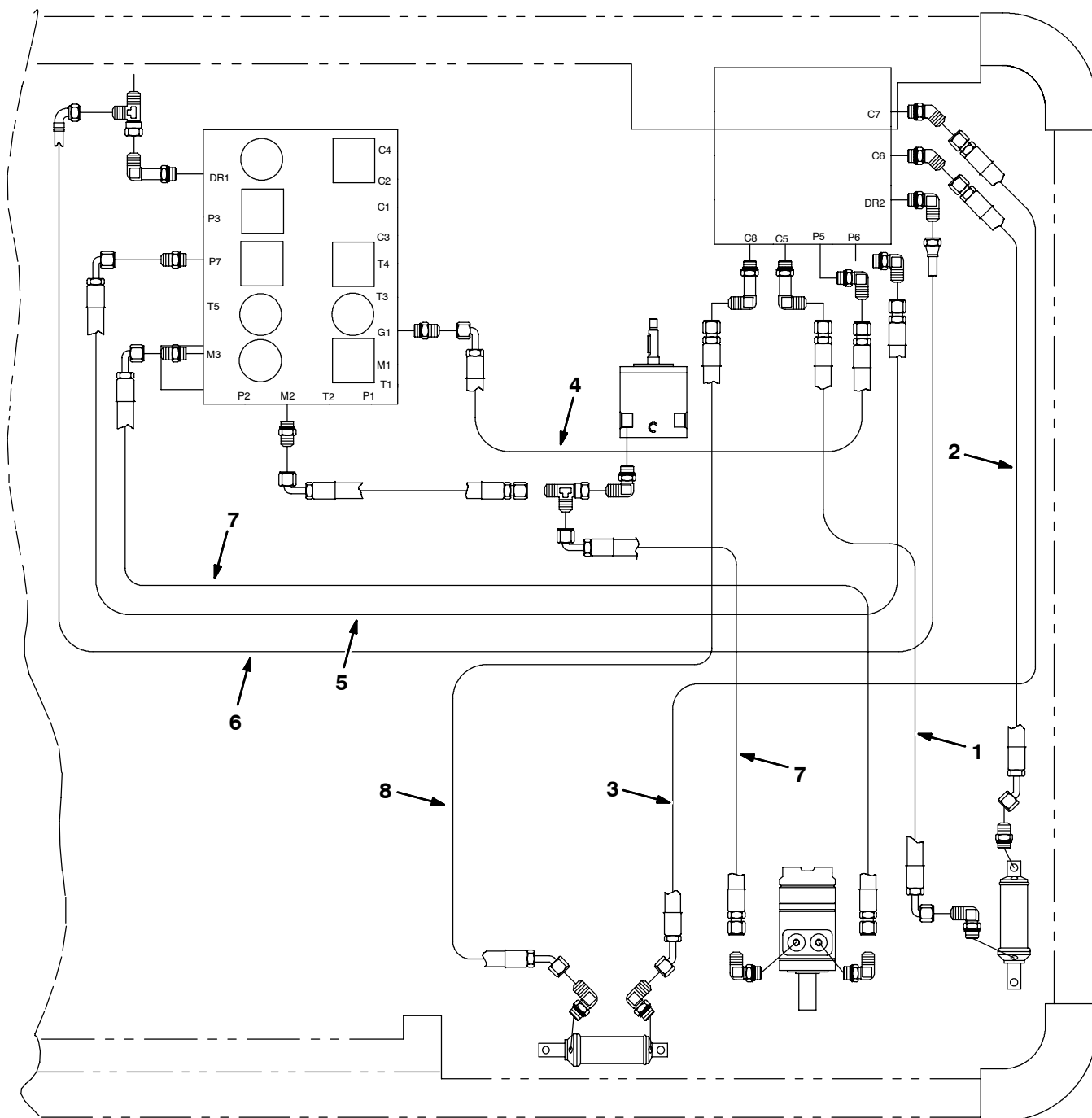
Fig. 63 - Side Brush Hydraulic Hose Group (740045 001-xxx) - Seitenbürsten-Hydraulikschlauch-Gruppe - Assemblage tuyaux hydrauliques de la brosse latérale
