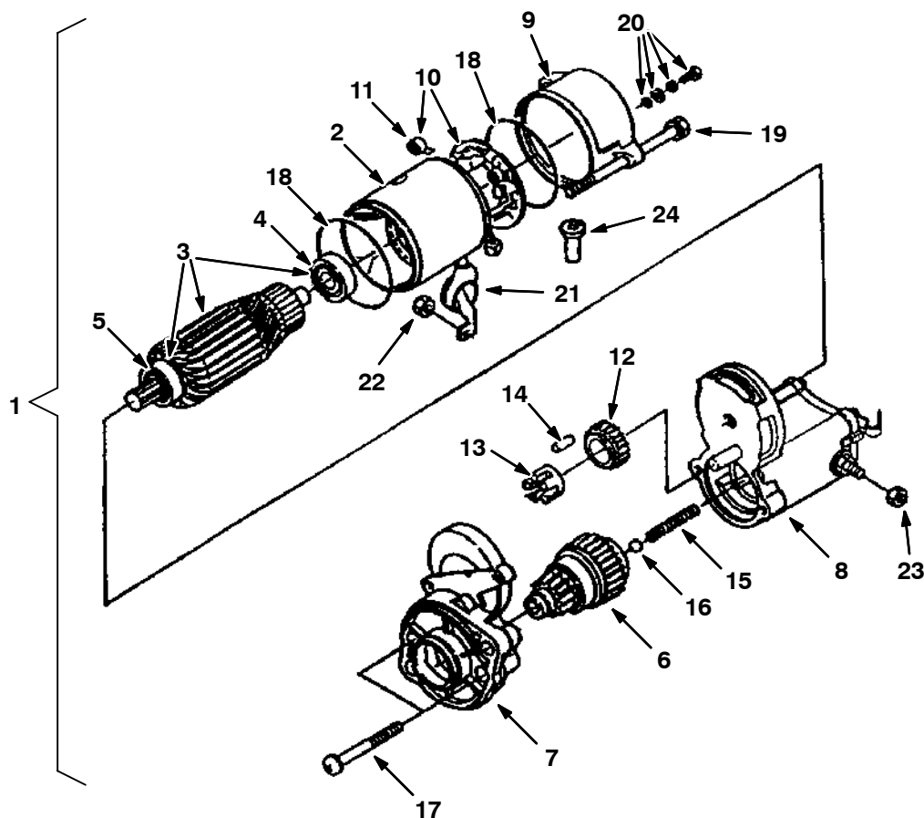
Fig. 13 - Starter Breakdown, 74405 - Anlasser-Defekt, 74405 - Panne de démarreur, 74405
