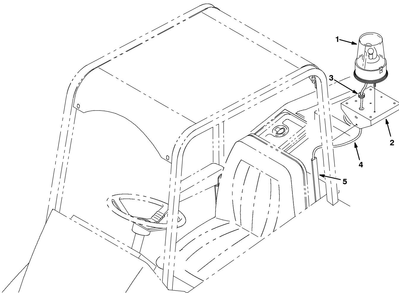
Fig. 2 - Revolving Light Kit, Overhead Guard - Warndrehlicht-Satz, Überkopf-Schutz - Jeu de pièces clignotant, protège-conducteur
