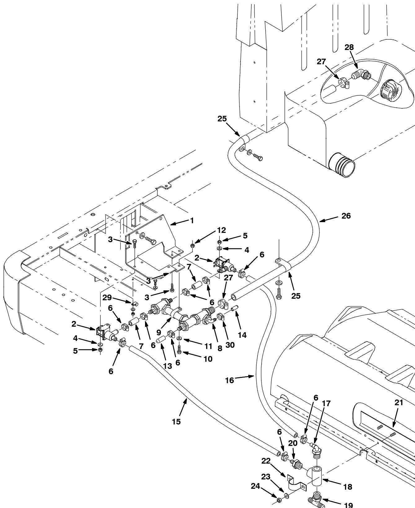
Fig. 27 - Solution Control Group - Frischwasser-Steuerungsgruppe - Assemblage système de contrôle de la solution
