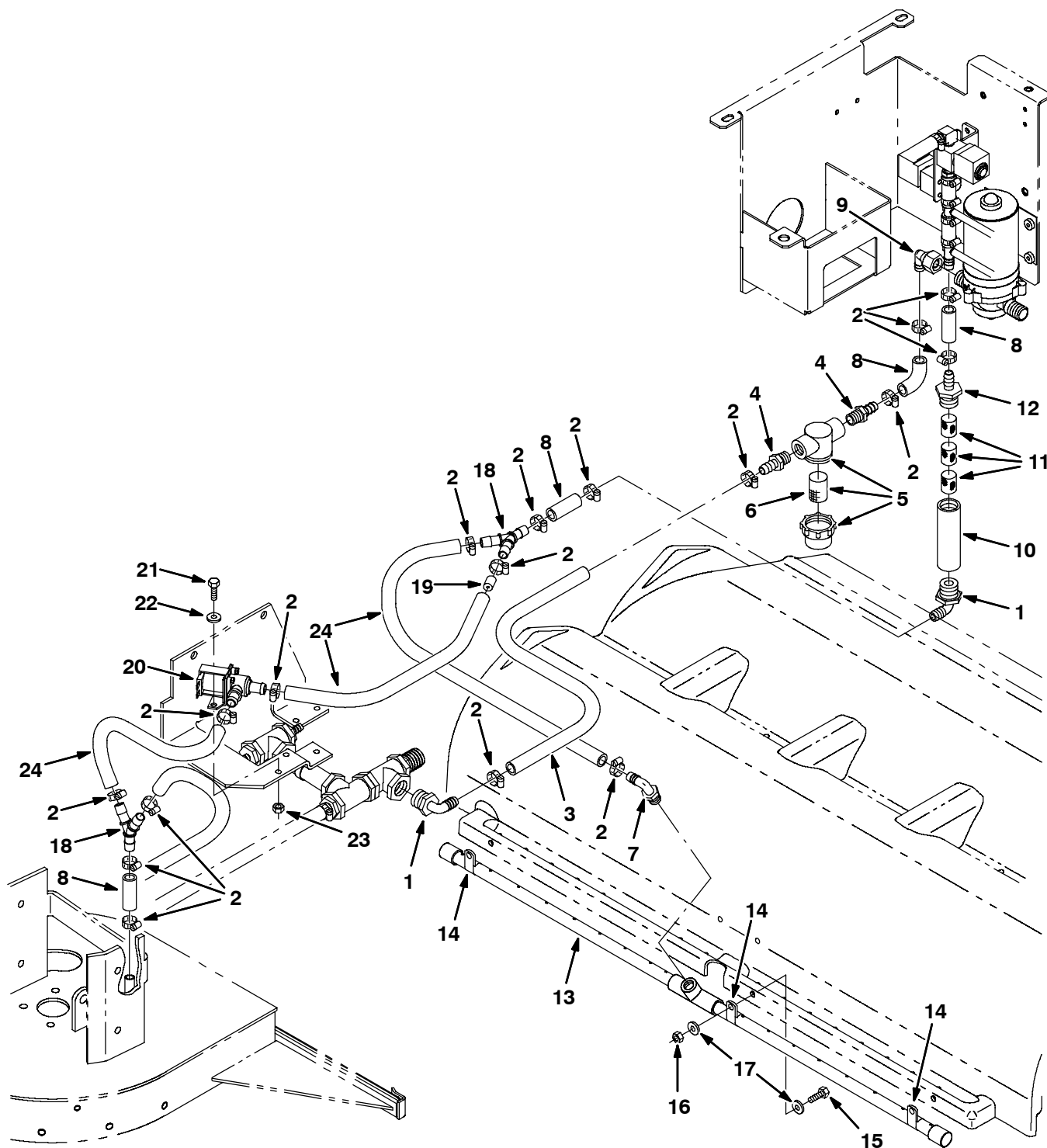
Fig. 65 - Side Brush FaST Foam Filter Group — Seitenbürsten-FaST-Schaumfilter-Einheit — Groupe filtre antimousse FaST de la brosse latérale
