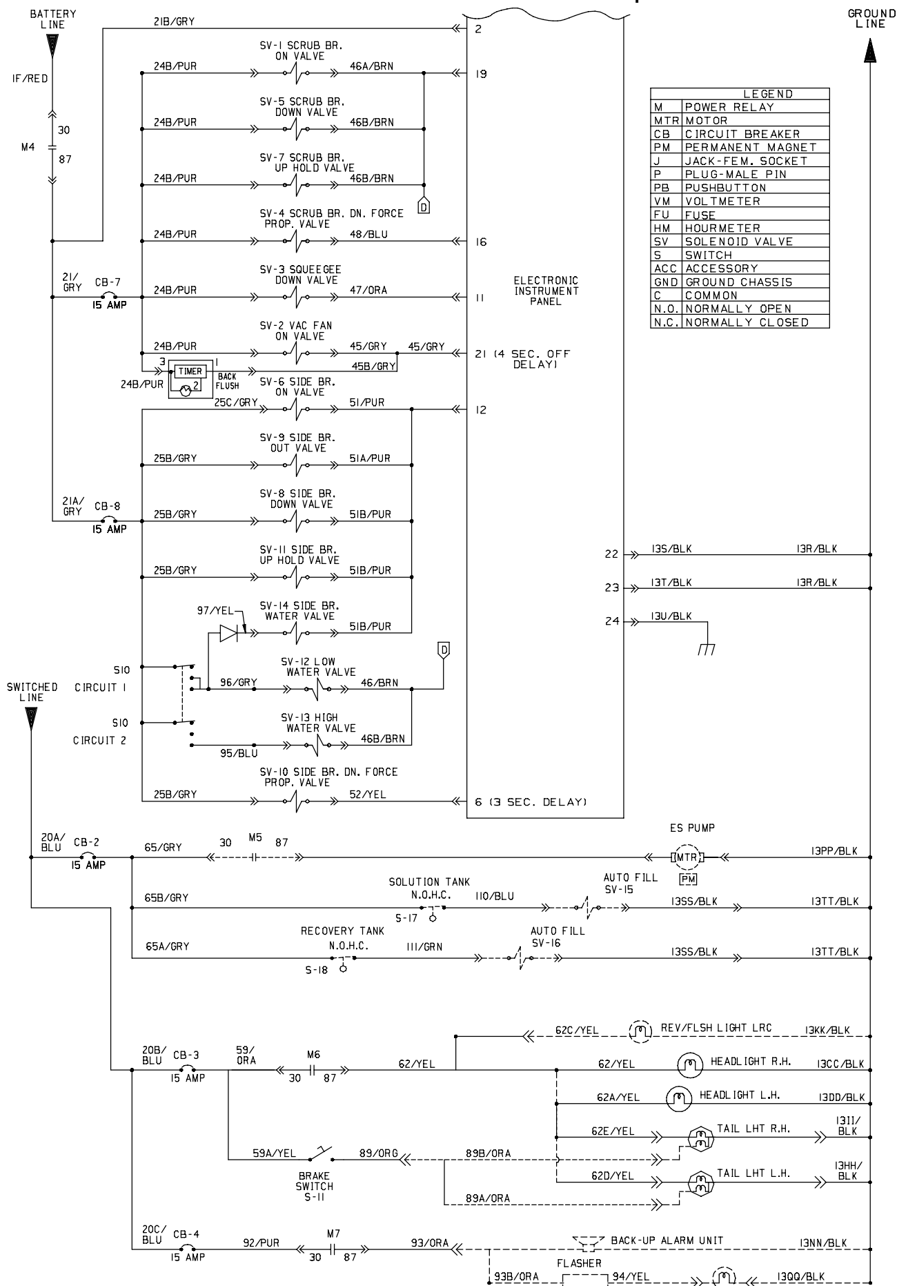
Fig. 40 - Electrical Schematic (7400 0000-7400 0542) - Schaltbild - Schéma des connexions électriques
