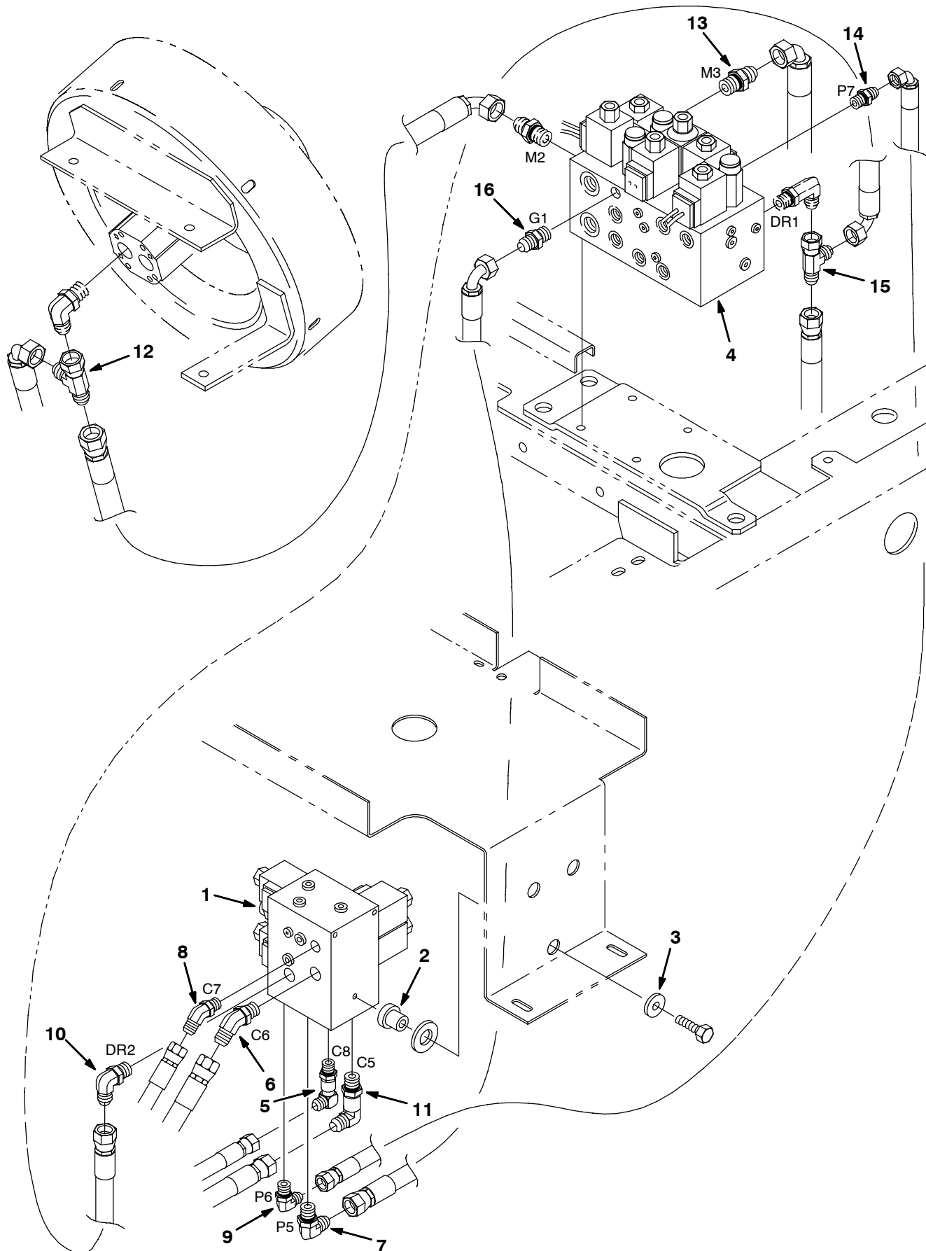
Fig. 61 - Side Brush Hydraulic Group (740045 001-xxx) - Seitenbürsten-Hydraulik-Gruppe - Assemblage système hydraulique de la brosse latérale
