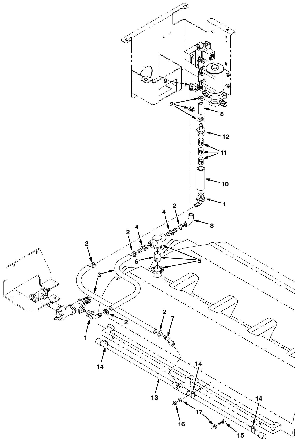
Fig. 67 - FaST Foam Filter Group — FaST-Schaumfilter-Einheit — Groupe filtre antimousse FaST
