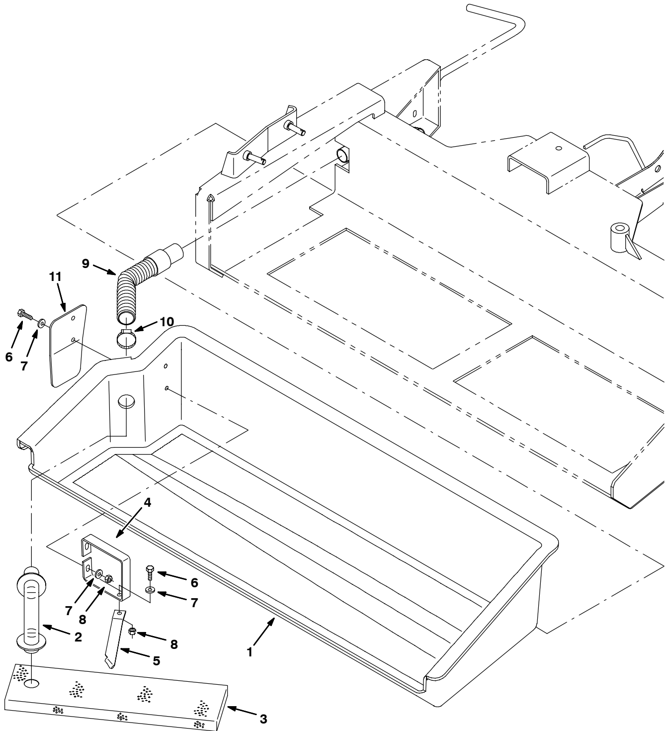
Fig. 50 - Debris Tray Trough Group - Schmutzkassette-Wannen-Gruppe - Assemblage cuvette du plateau à détrit
