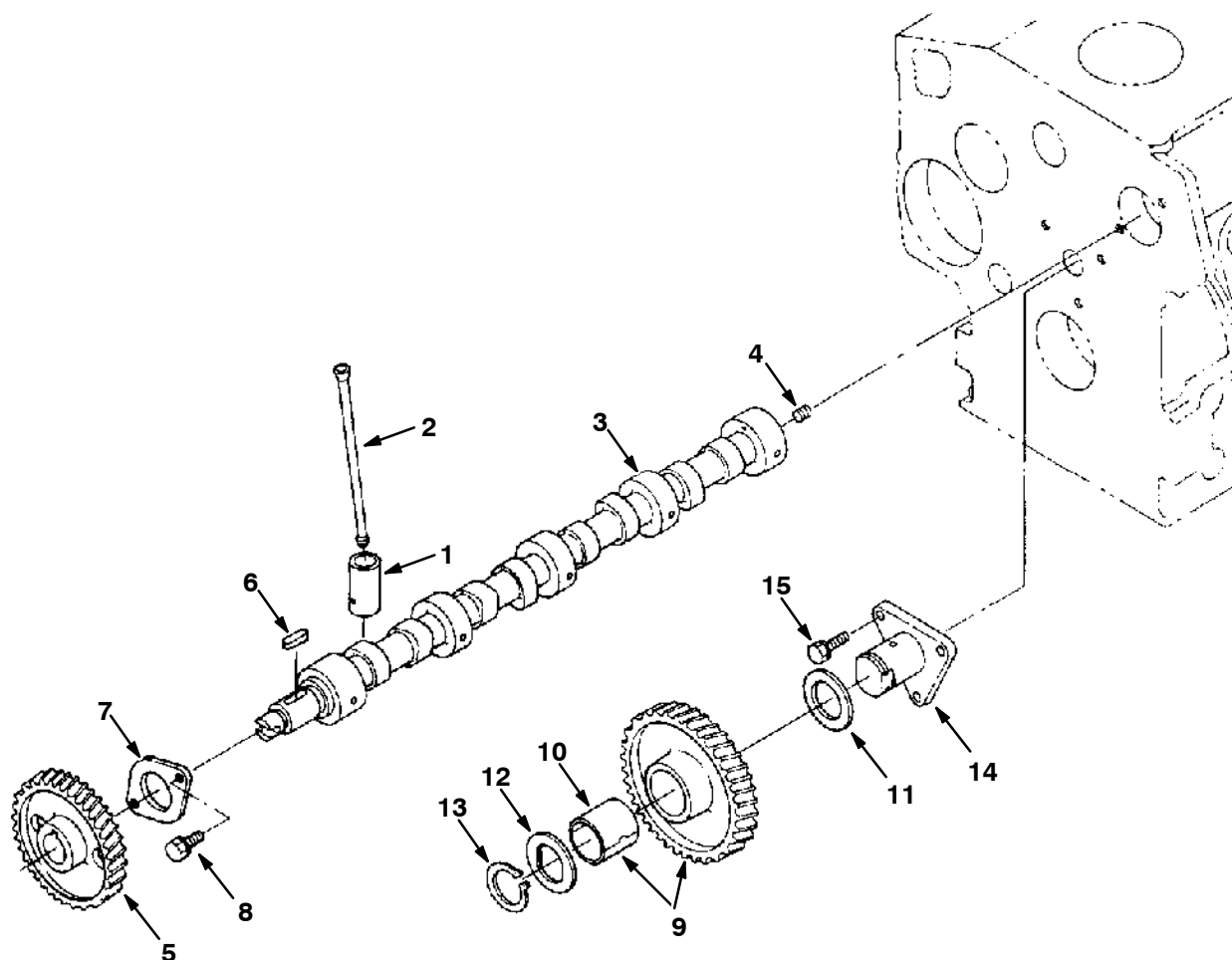
Fig. 10 - Camshaft Group - Nockenwellen-Gruppe - Assemblage arbre à cames
