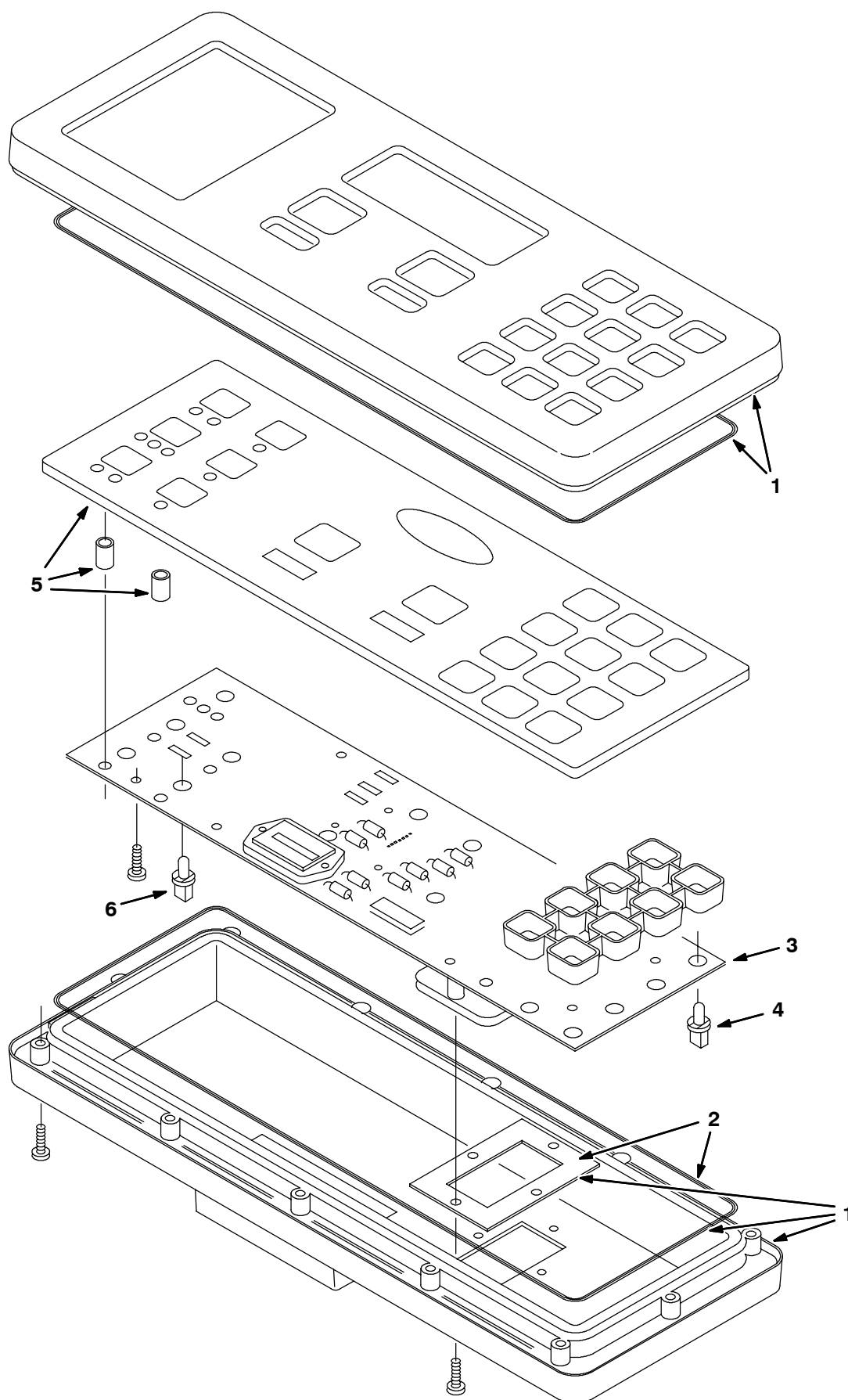
Fig. 10 - Instrument Panel Assembly - Armaturen Brett-Gruppe - Assemblage tableau de bord
