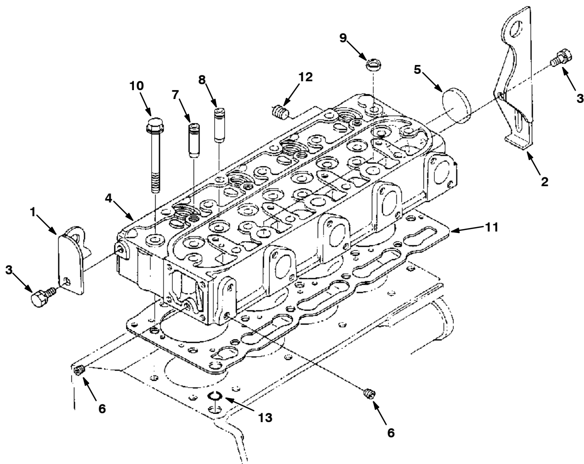
Fig. 3 - Cylinder Head Group - Zylinderkopf-Gruppe - Assemblage culasse
