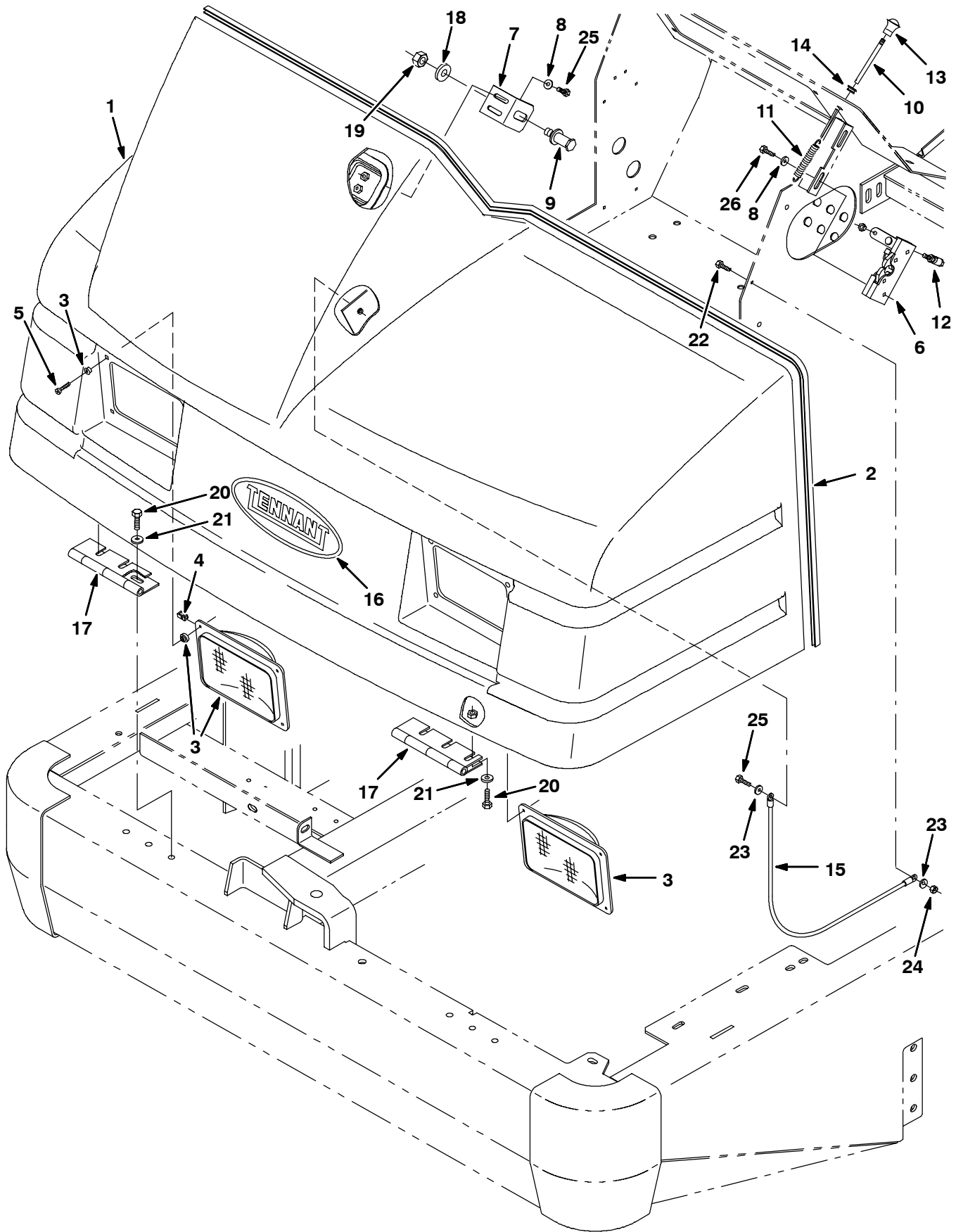
Fig. 6 - Front Hood Group - Vorderhauben-Gruppe - Assemblage capot
