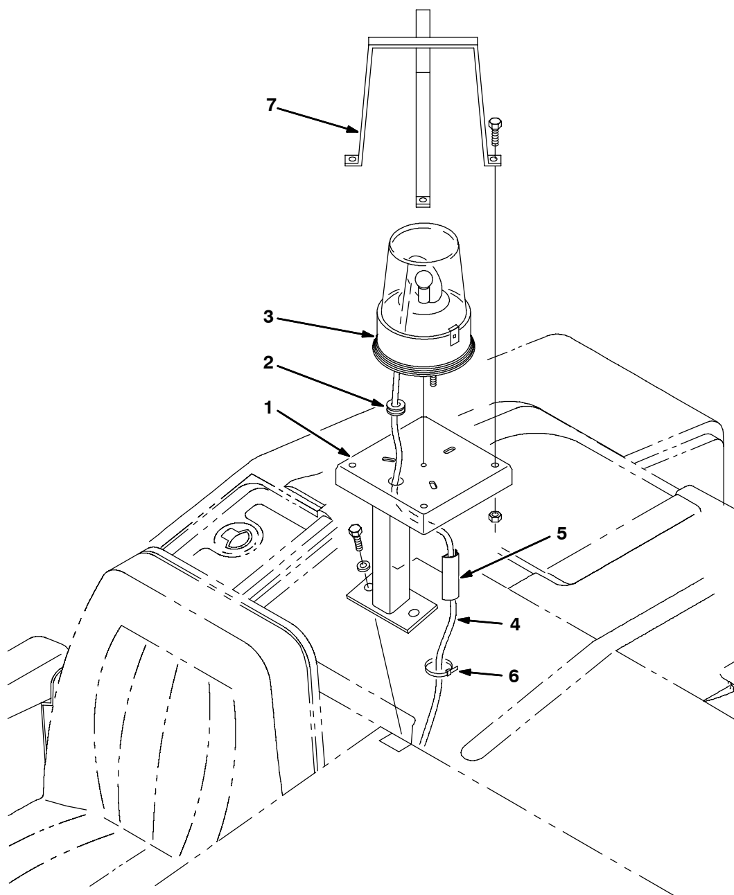
Fig. 4 - Revolving Light Kit, LRC - Blinklicht-Satz LRC - Jeu de pièces gyrophare, côtés droit et gauche
