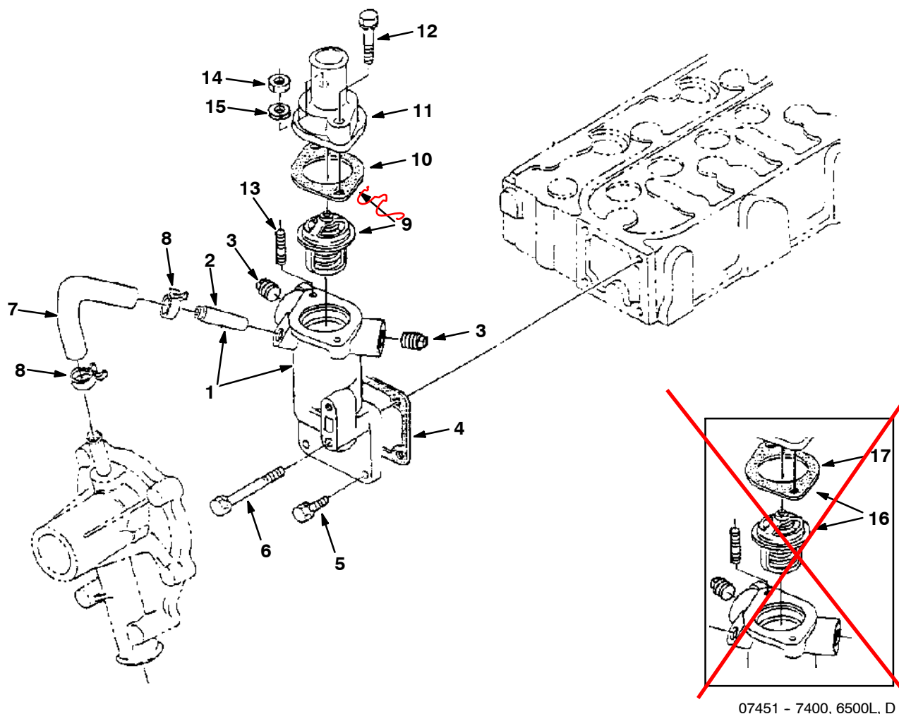
Fig. 21 - Water Flange Group - Wasserflansch-Gruppe - Assemblage flasque à eau
