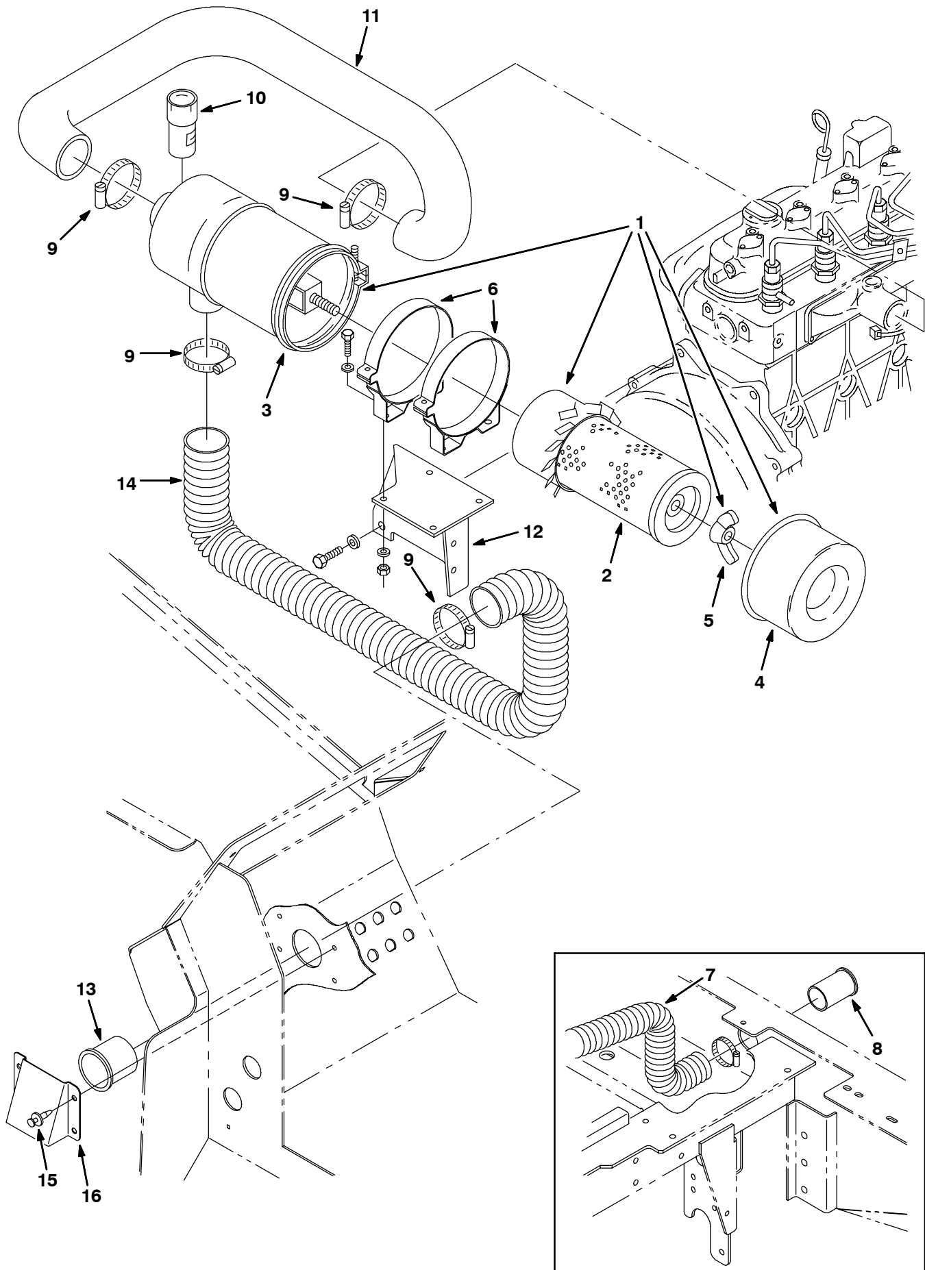
Fig. 15 - Air Cleaner Group - Luft-Reinigungsgruppe - Assemblage épurateur d'air
