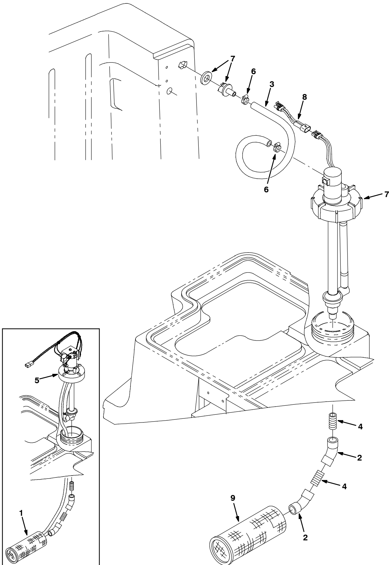
Fig. 57 - ES Pump Column Group (7400 0075- ) - ES-Pumpensäulen-Gruppe - Assemblage colonne de pompage ES
