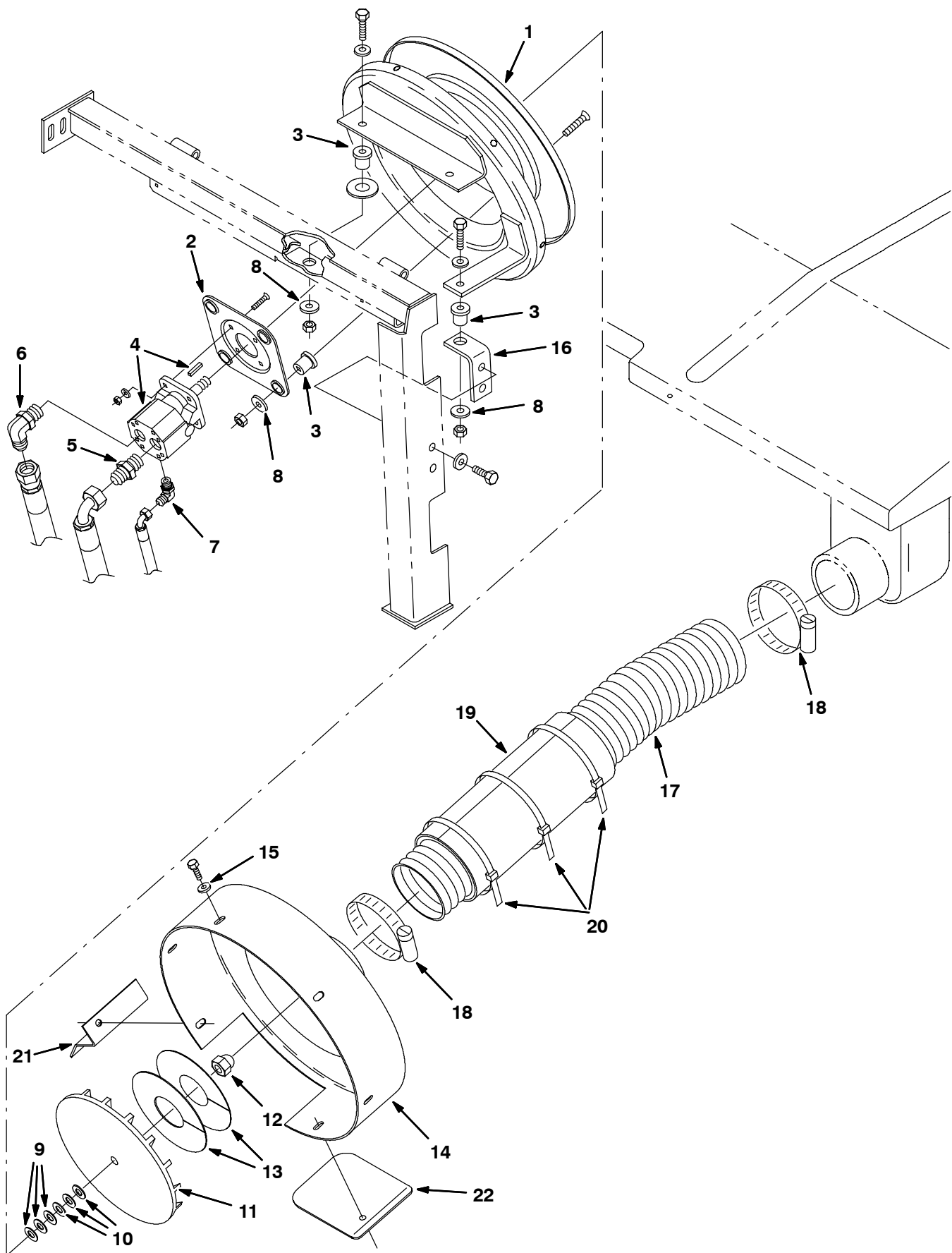
Fig. 26 - Vacuum Fan Group - Vakuumgebläse-Gruppe - Assemblage extracteur
