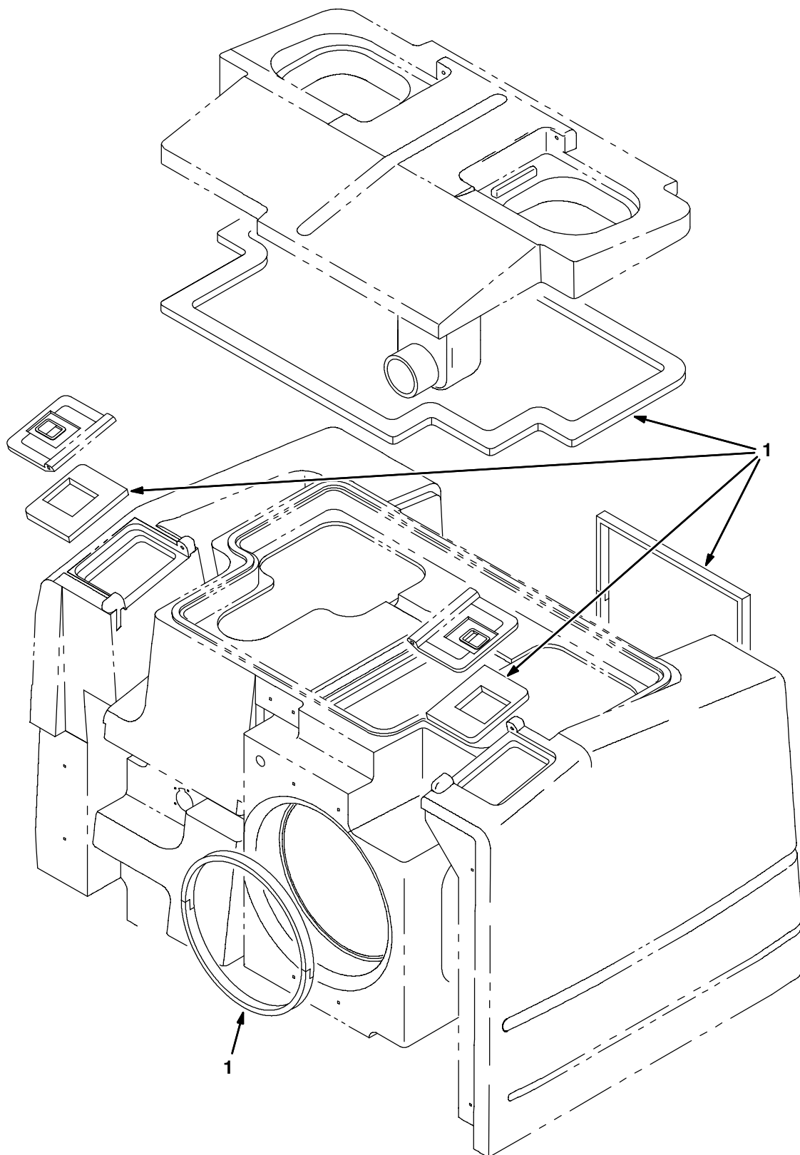
Fig. 32 - Solution and Recovery Tank Gaskets Group - Frischwasser-/Schmutzwasser-Tankdichtungsgruppe Assemblage joints du réservoir de solution et du réservoir de récupération
