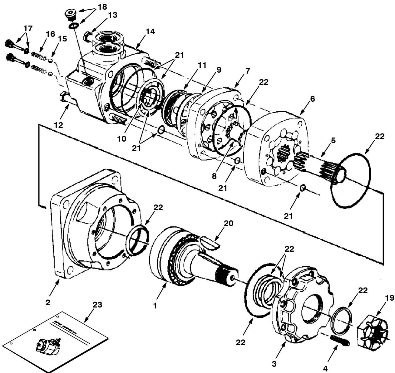
Fig. 3 - Hydraulic Motor Breakdown, 71724 - Hydraulik-Motor-Defekt - Panne de moteur hydraulique, 71724
