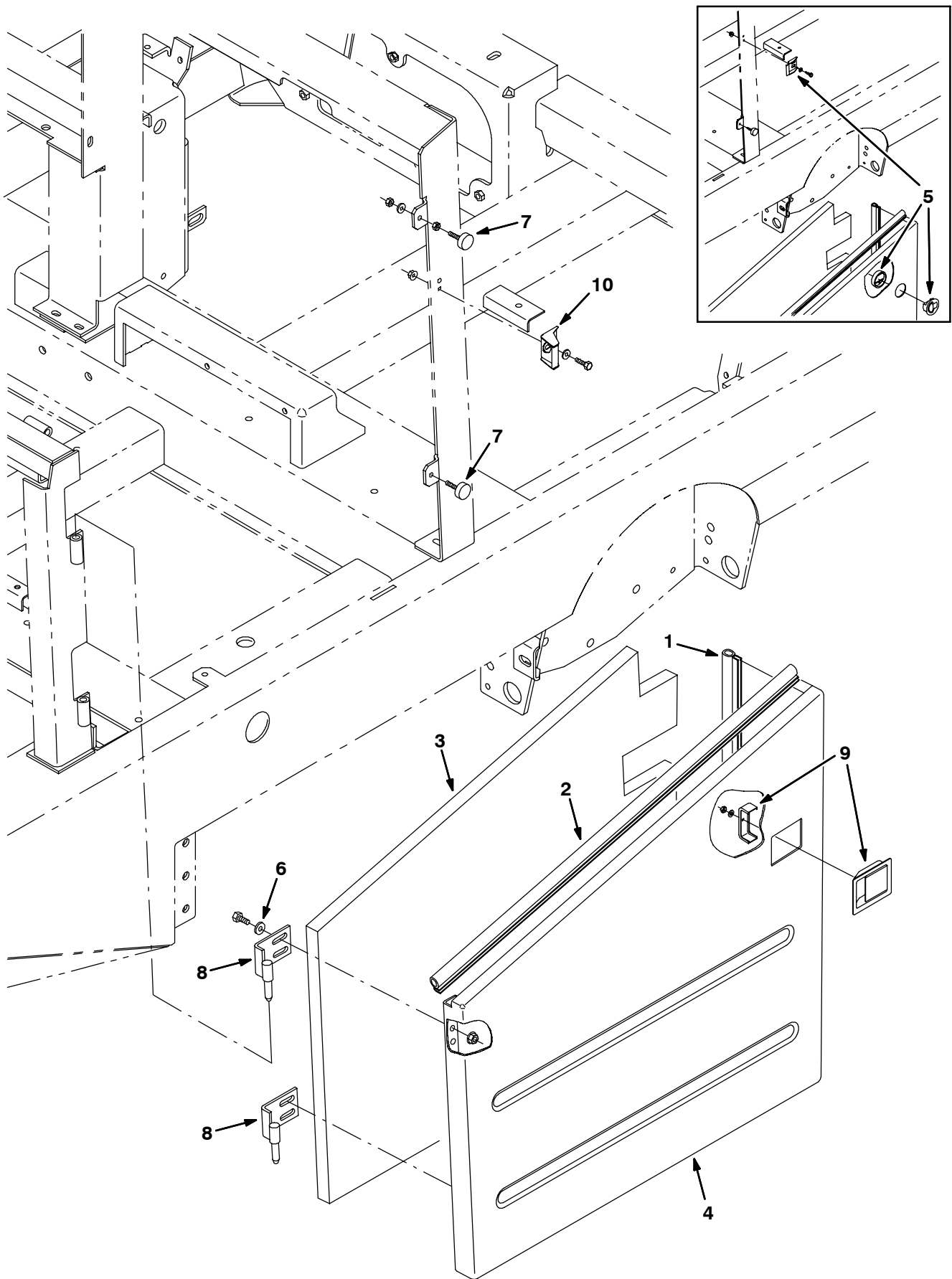
Fig. 7 - Engine Side Door Group - Motor-Seitenklappen-Gruppe - Assemblage porte latérale du moteur
