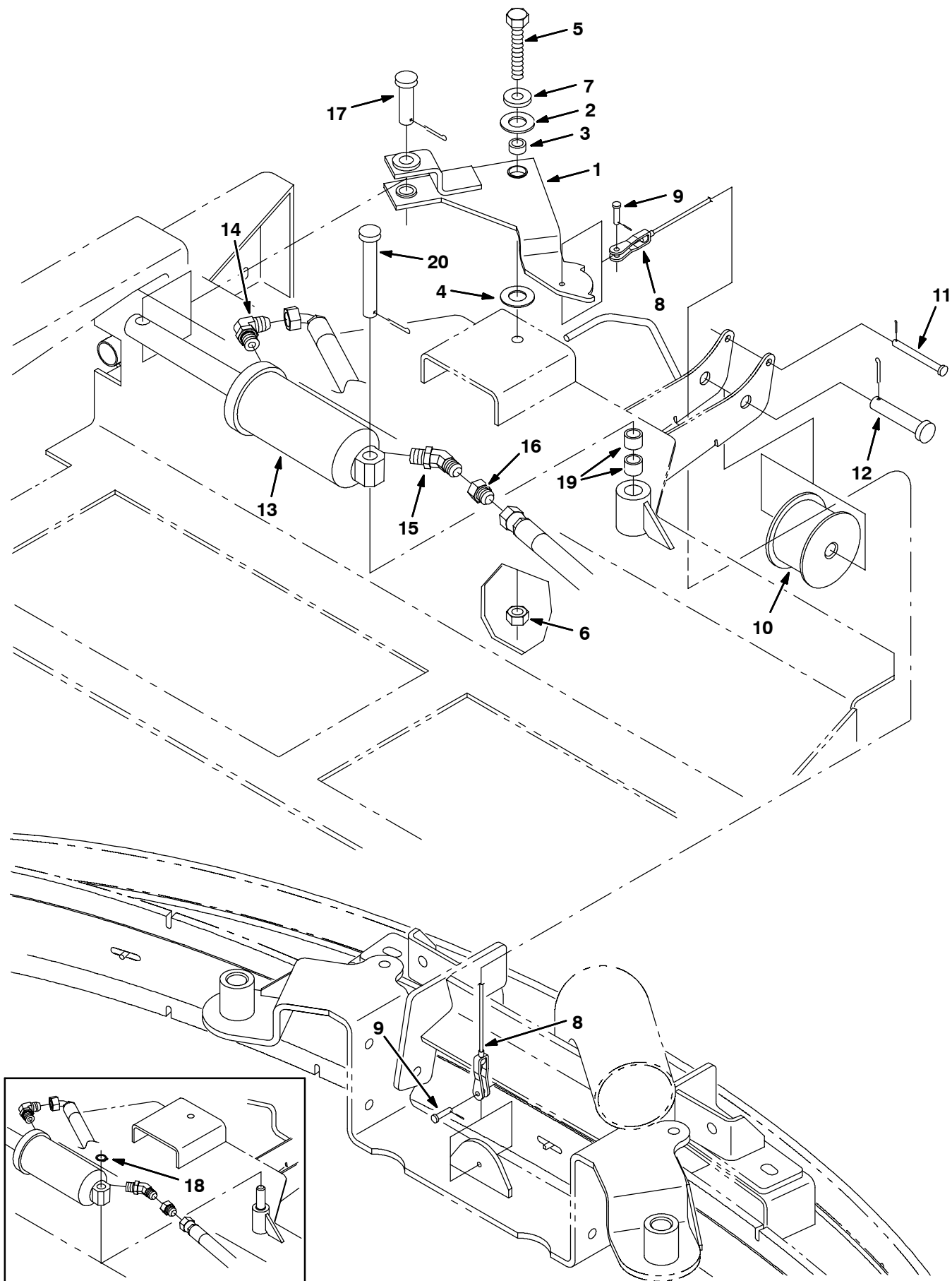
Fig. 51 - Rear Squeegee Lift Group - Heck-Abstreifleisten-Hebe-Gruppe - Assemblage système de levage du racloir arrière
