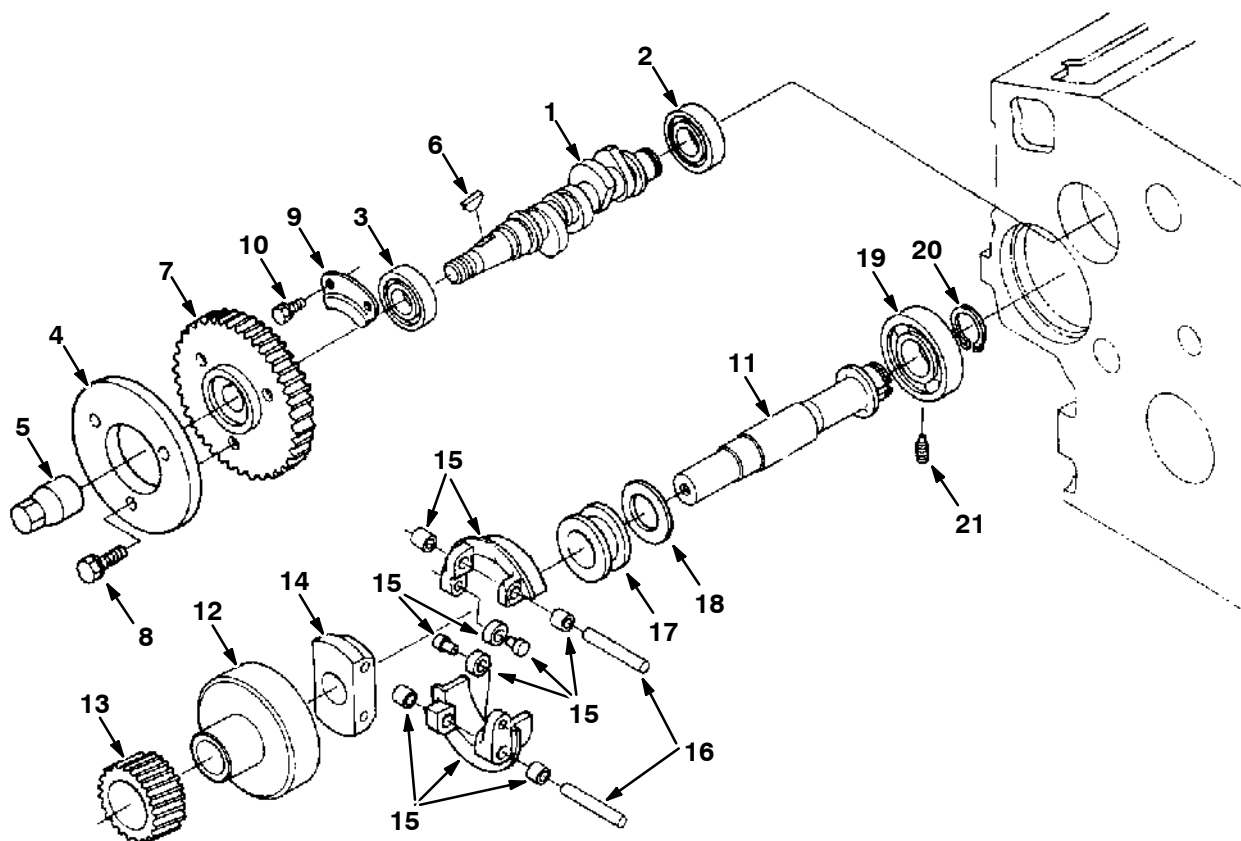
Fig. 17 - Fuel Camshaft Group - Kraftstoff-Nockenwellen-Gruppe - Assemblage arbre à cames de carburant
