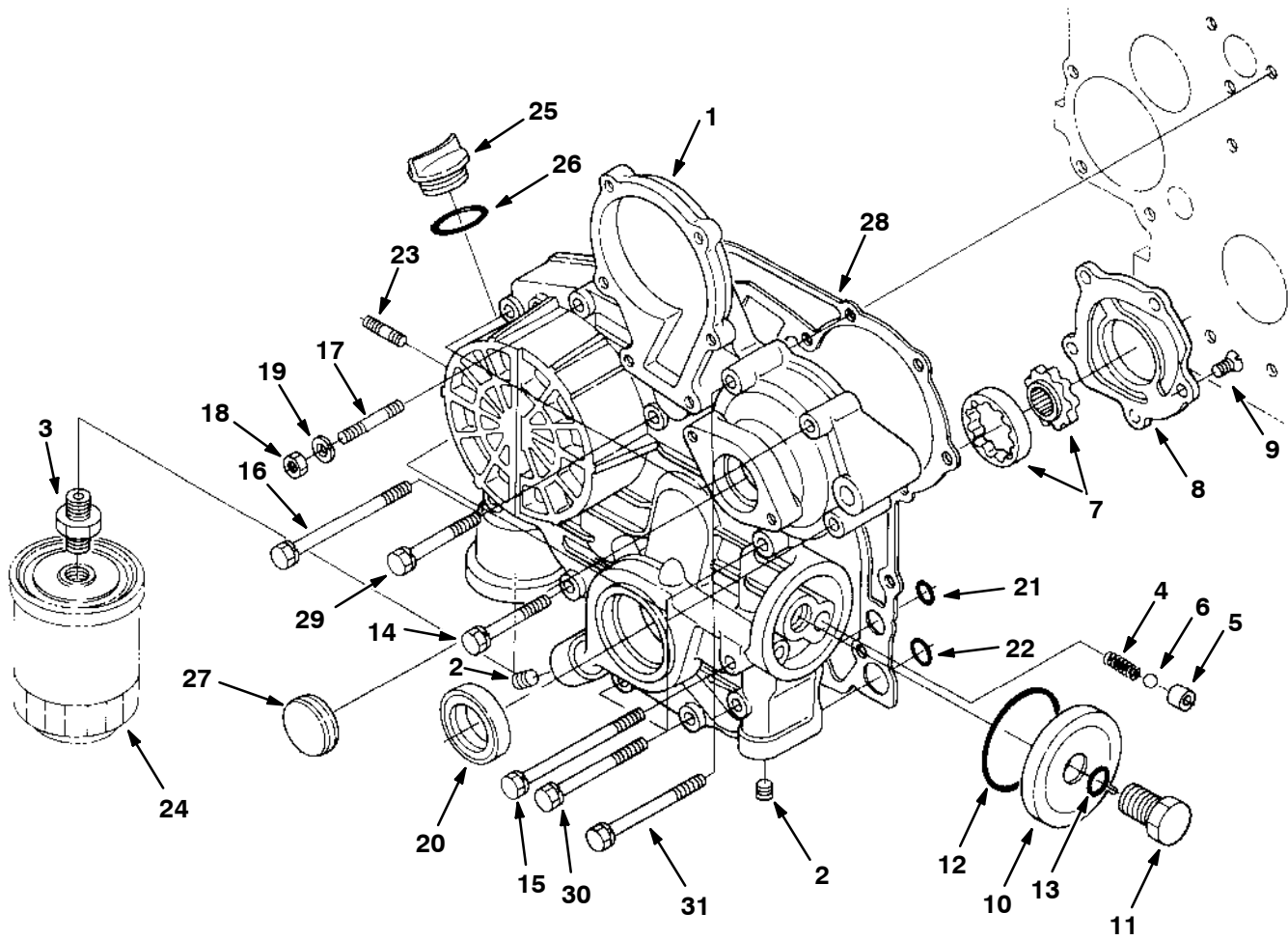
Fig. 4 - Gear Case Group - Getriebekasten-Gruppe - Assemblage boîte d'engrenages
