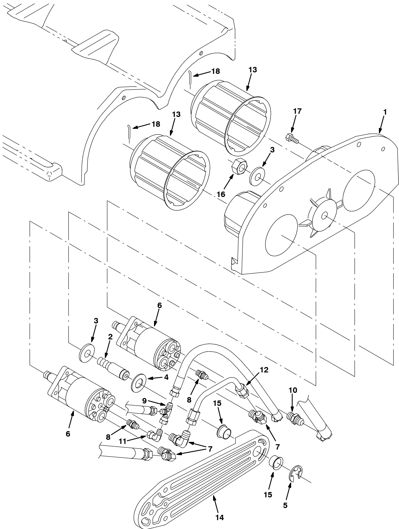
Fig. 45 - Scrub Brush Drive Motor Group - Schrubbbürsten-Antriebs-Motor-Gruppe - Groupe moteur d'entraînement de brosse dure
