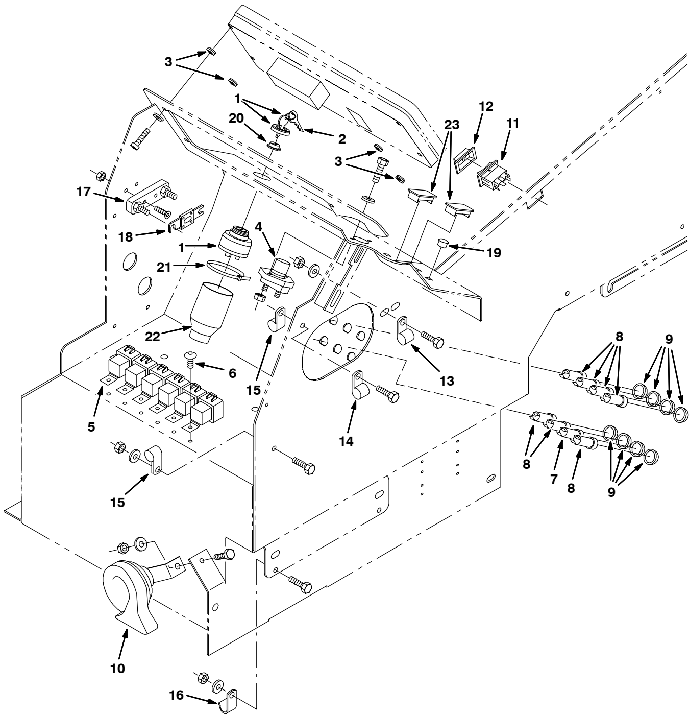
Fig. 11 - Circuit Breaker and Relay Group - Schutzschalter-/Relais-Gruppe - Assemblage coupe-circuit et relais
