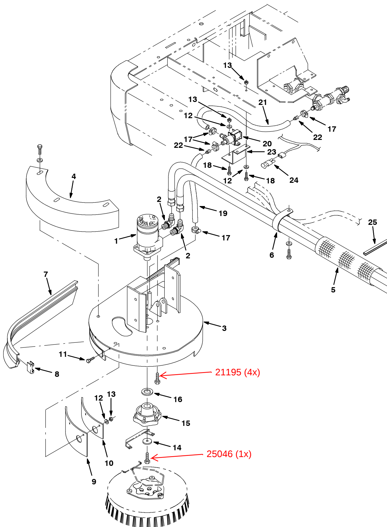
Fig. 60 - Side Brush Motor Group - Seitenbürsten-Motorgruppe - Assemblage moteur de la brosse latérale
