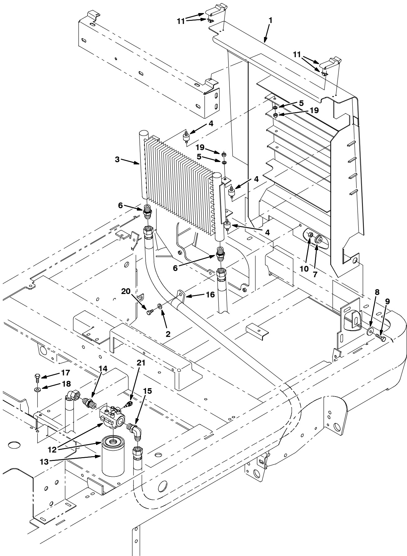
Fig. 39 - Hydraulic Filter and Cooler Group - Hydraulik-Filter-/Kühler-Gruppe - Assemblage filtre et refroidisseur du système hydraulique
