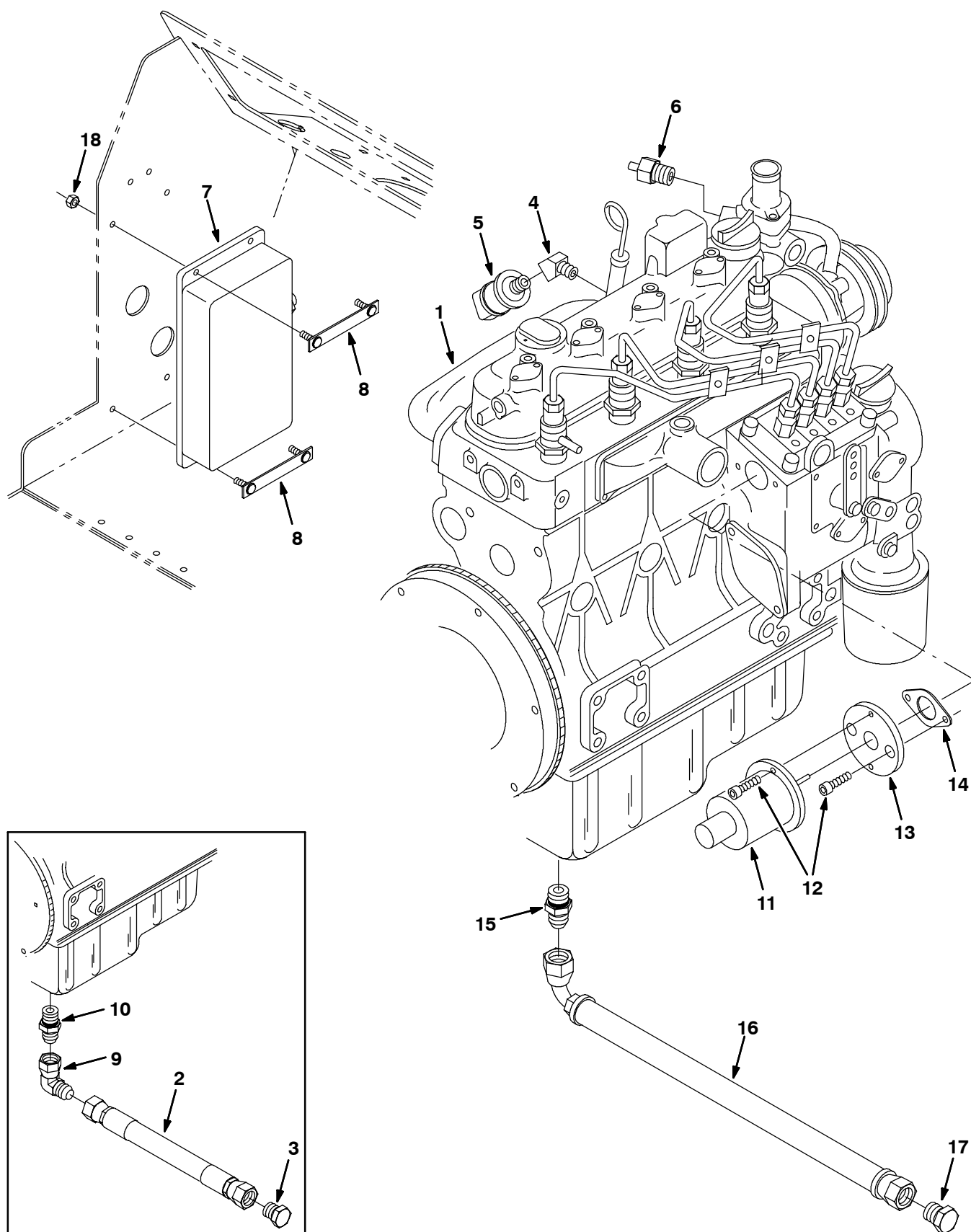
Fig. 13 - Engine and Governor Group (7400 0501- ) - DieselMotor und Regler Gruppe - Groupe du moteur et régulateur
