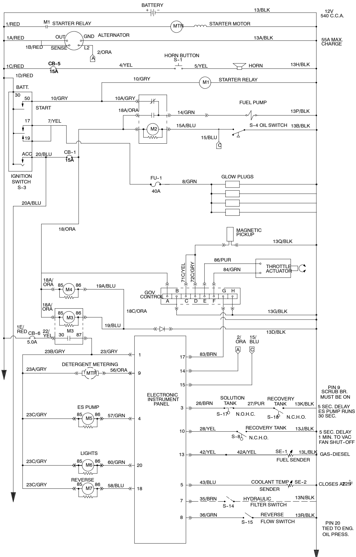
Fig. 40 - Electrical Schematic (7400 0000-7400 0542) - Schaltbild - Schéma des connexions électriques
