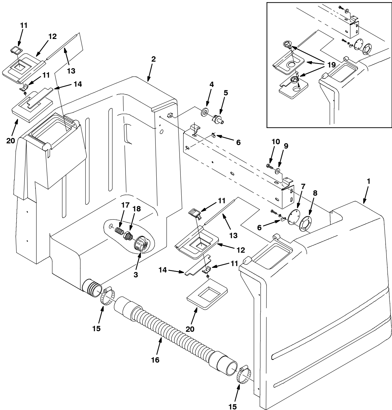
Fig. 28 - ES Solution Tank Group - ES-Frischwasser-Tankgruppe - Assemblage réservoir de solution ES
