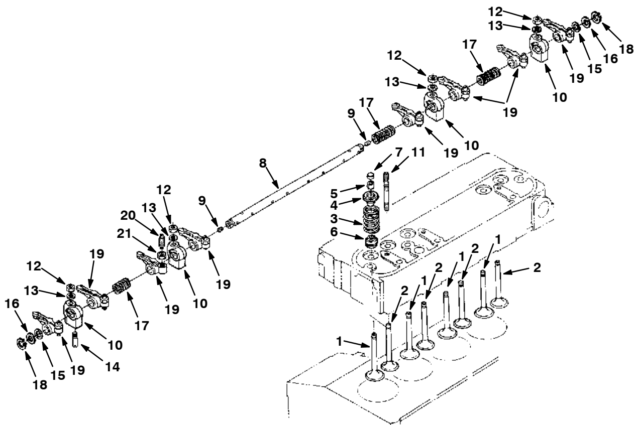
Fig. 9 - Valve, Rocker Arm Group - Ventil-/Kipphebel-Gruppe - Assemblage soupape, culbuteur
