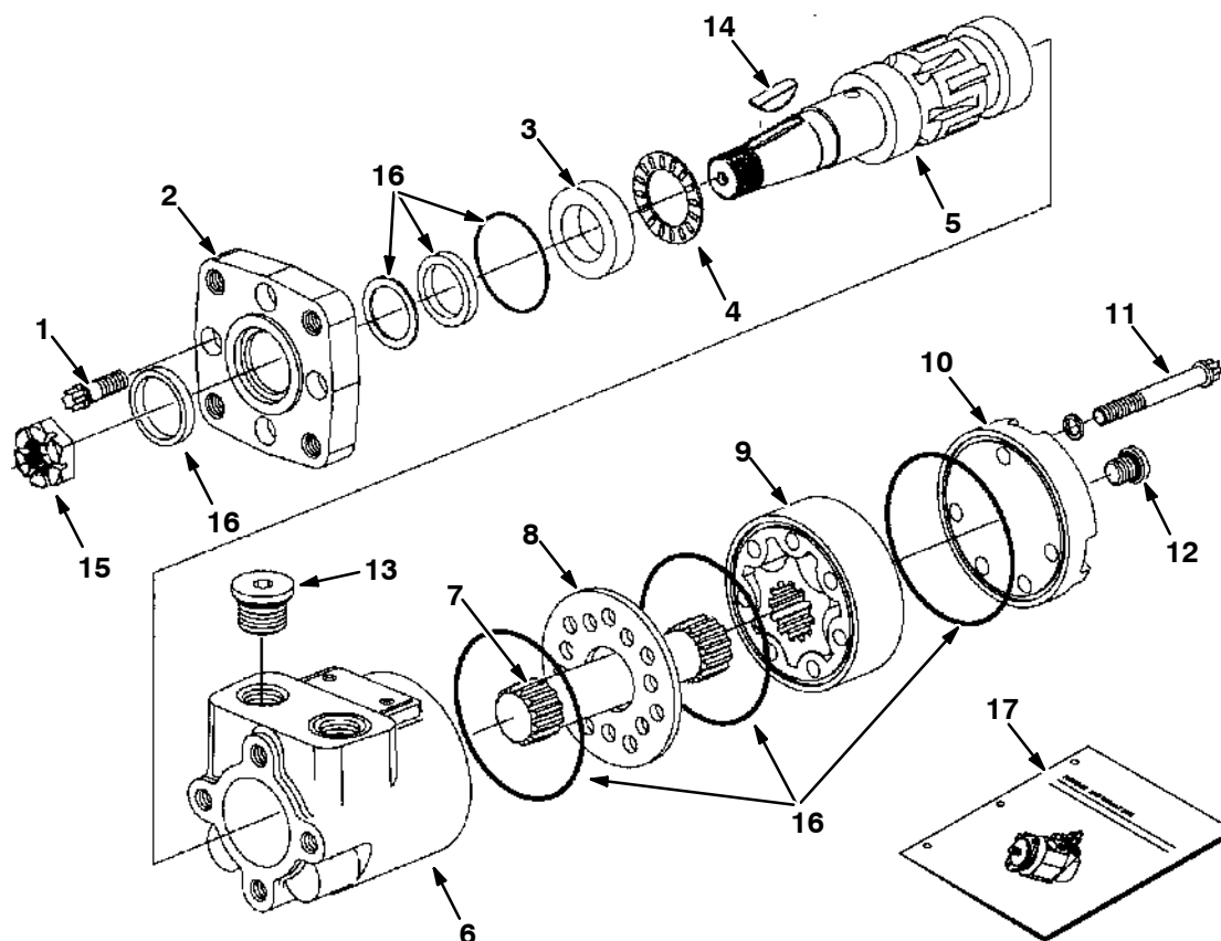
Fig. 5 - Hydraulic Motor Breakdown, 71729 - Hydraulik-Motor-Defekt - Panne de moteur hydraulique, 71729
