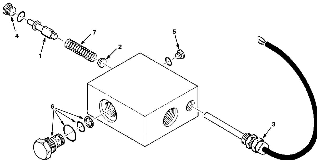
Fig. 21 - Hydraulic Flow Sensor Switch Breakdown, 73430 - Hydraulik-Durchfluß-Sensorschalter-Defekt - Panne d'interrupteur du capteur de débit, 73430
