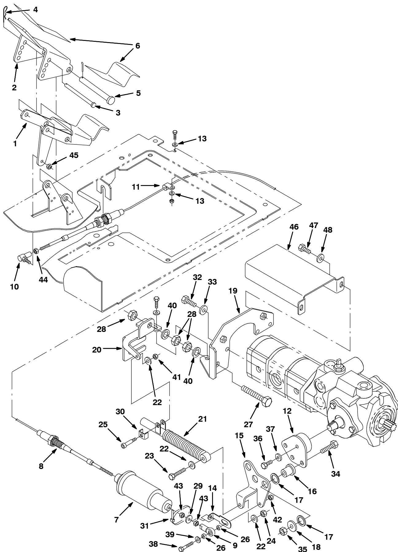
Fig. 25 - Directional Pedal and Linkage Group - Lenkpedal-/Gestängegruppe - Assemblage pédale de direction et timonerie
