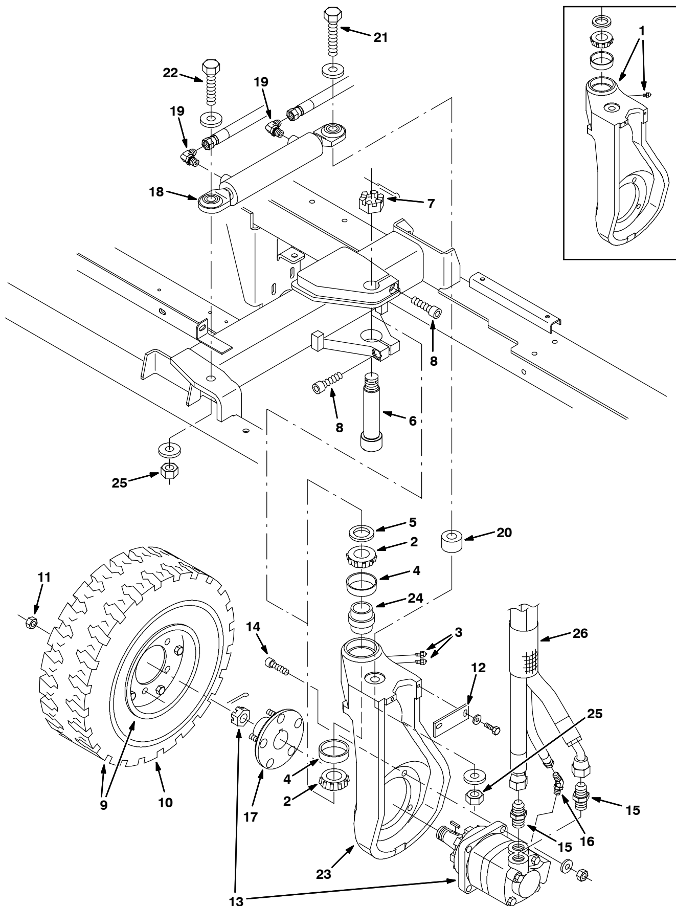
Fig. 22 - Front Drive Wheel Group - Vorderantrieb-Radgruppe - Assemblage roues motrices avant
