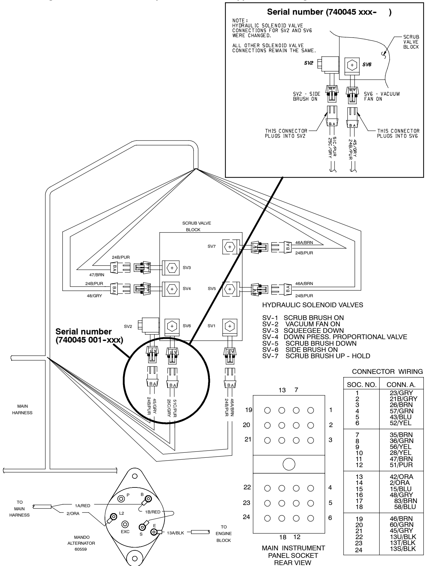
Fig. 42 - Wire Harness Group - Kabelbaum-Gruppe - Assemblage harnais de câbles
