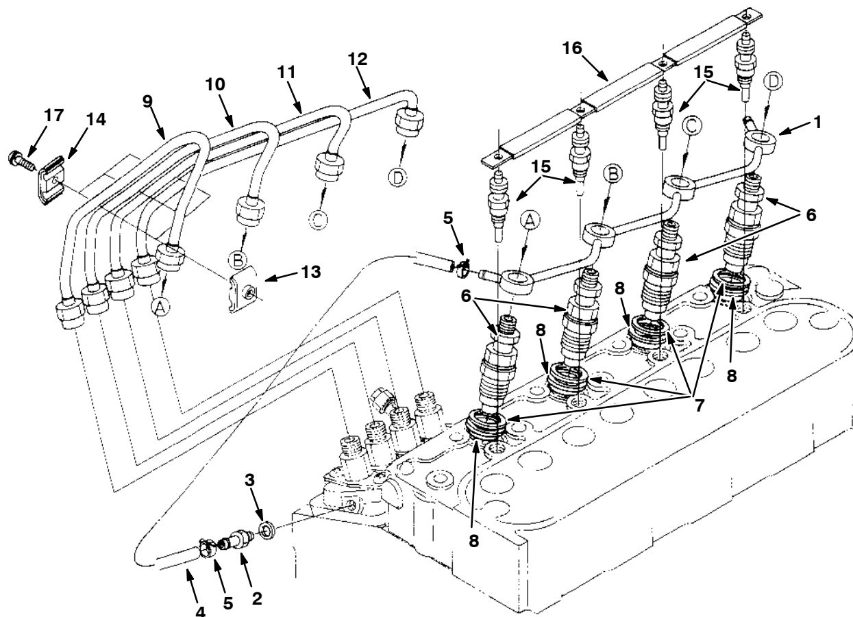
Fig. 14 - Nozzle Holder Group - Düsen-Halter-Gruppe - Assemblage porte-injecteur
