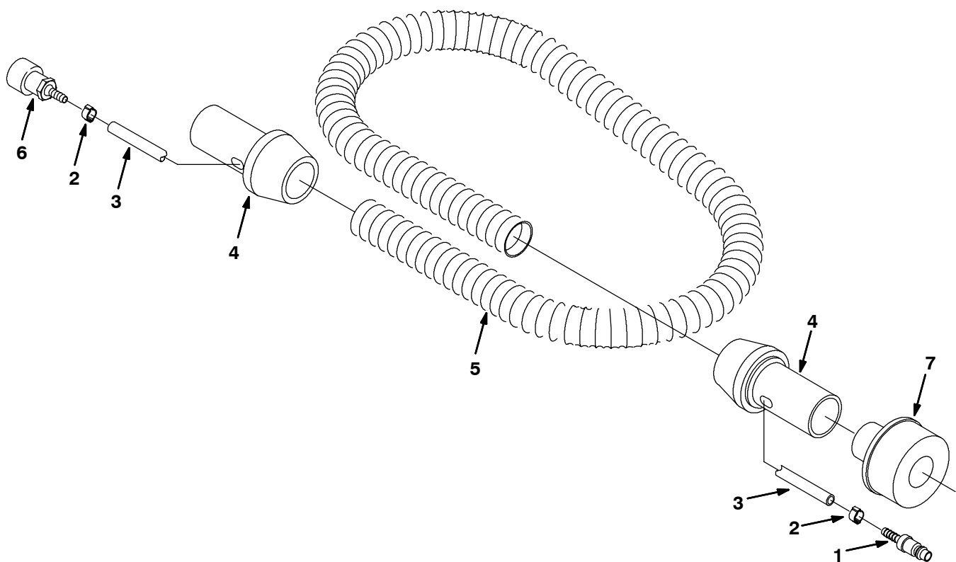
Fig. 18 - Power Wand Hose Assembly - Handschrubbschlauch Gruppe - Groupe Tuyau flexible de la Laveuse à Main
