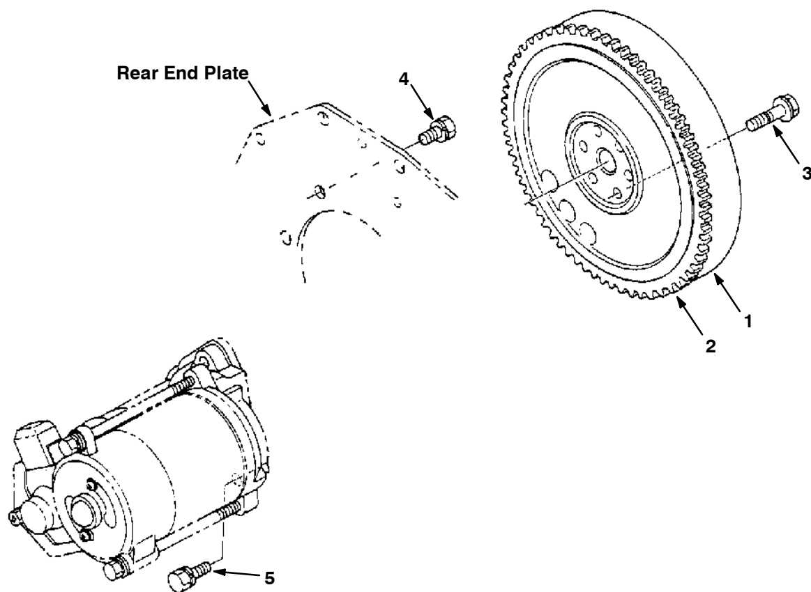
Fig. 12 - Flywheel Group - Schwungrad-Gruppe - Assemblage volant-moteur
