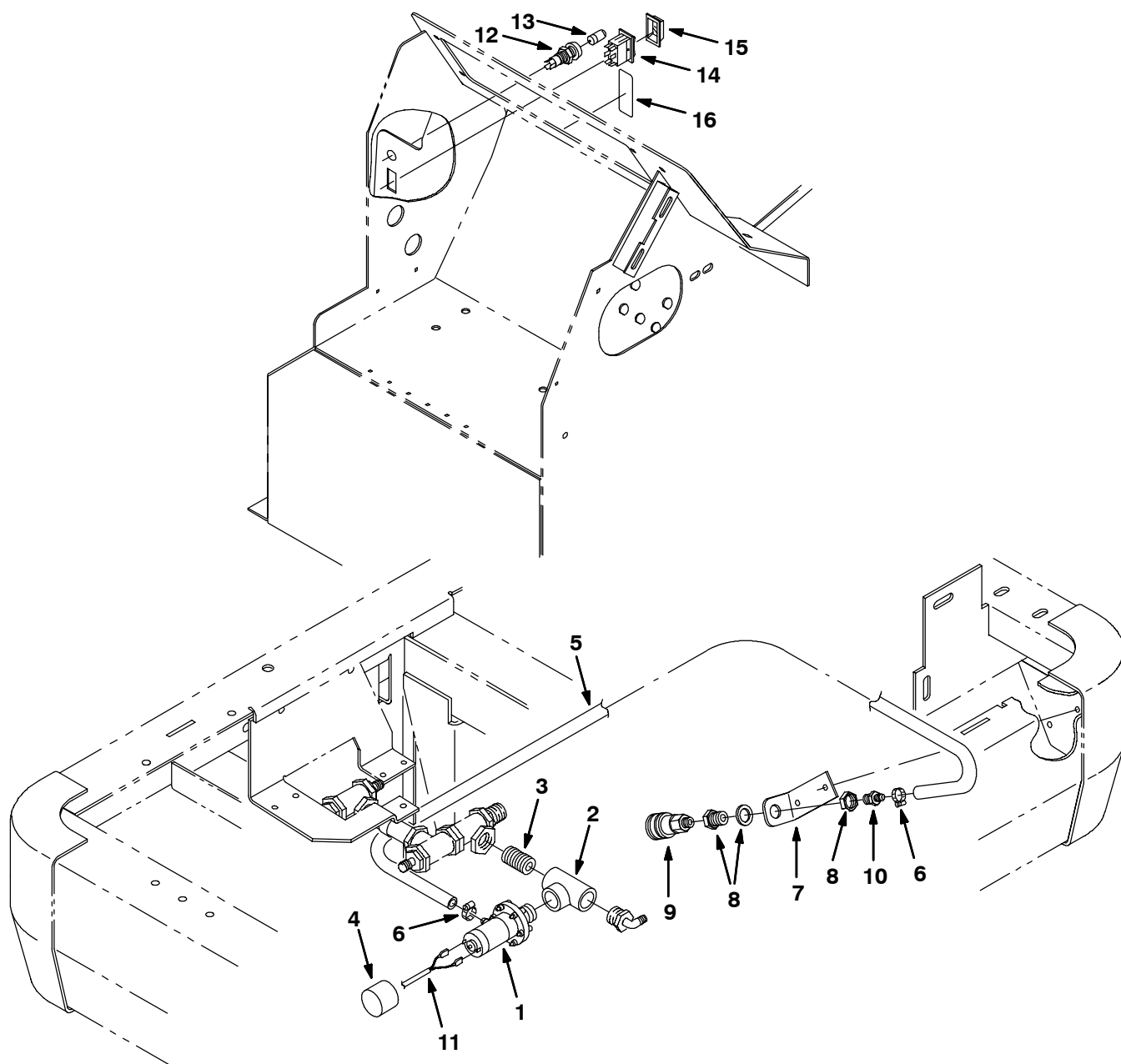
Fig. 16 - Power Wand Pump and Fittings Group - Wasserpumpe und Anschluß Gruppe - Groupe de la Pompe à Eau et des Raccords
