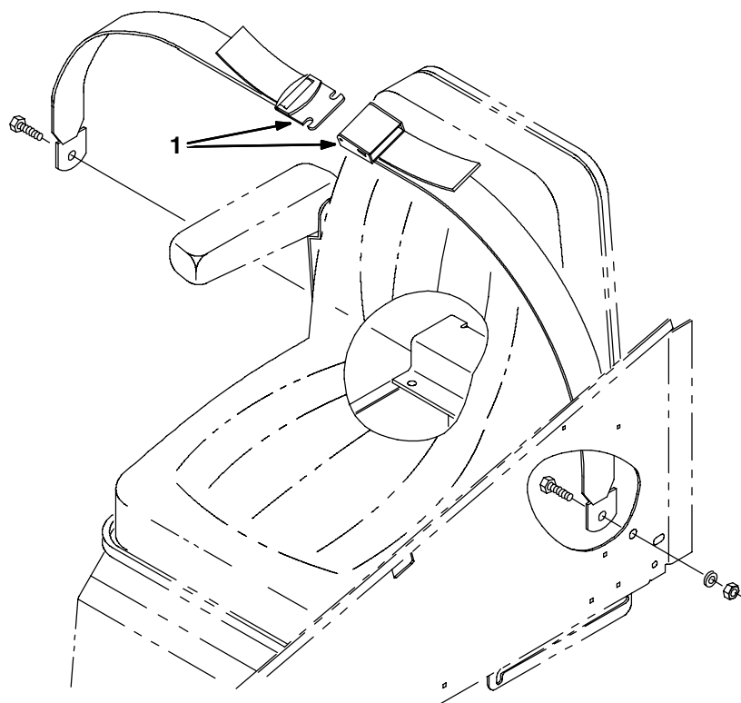
Fig. 8 - Seat Belt Kit - Sitzgurt-Satz - Jeu de pièces ceinture de sécurité
