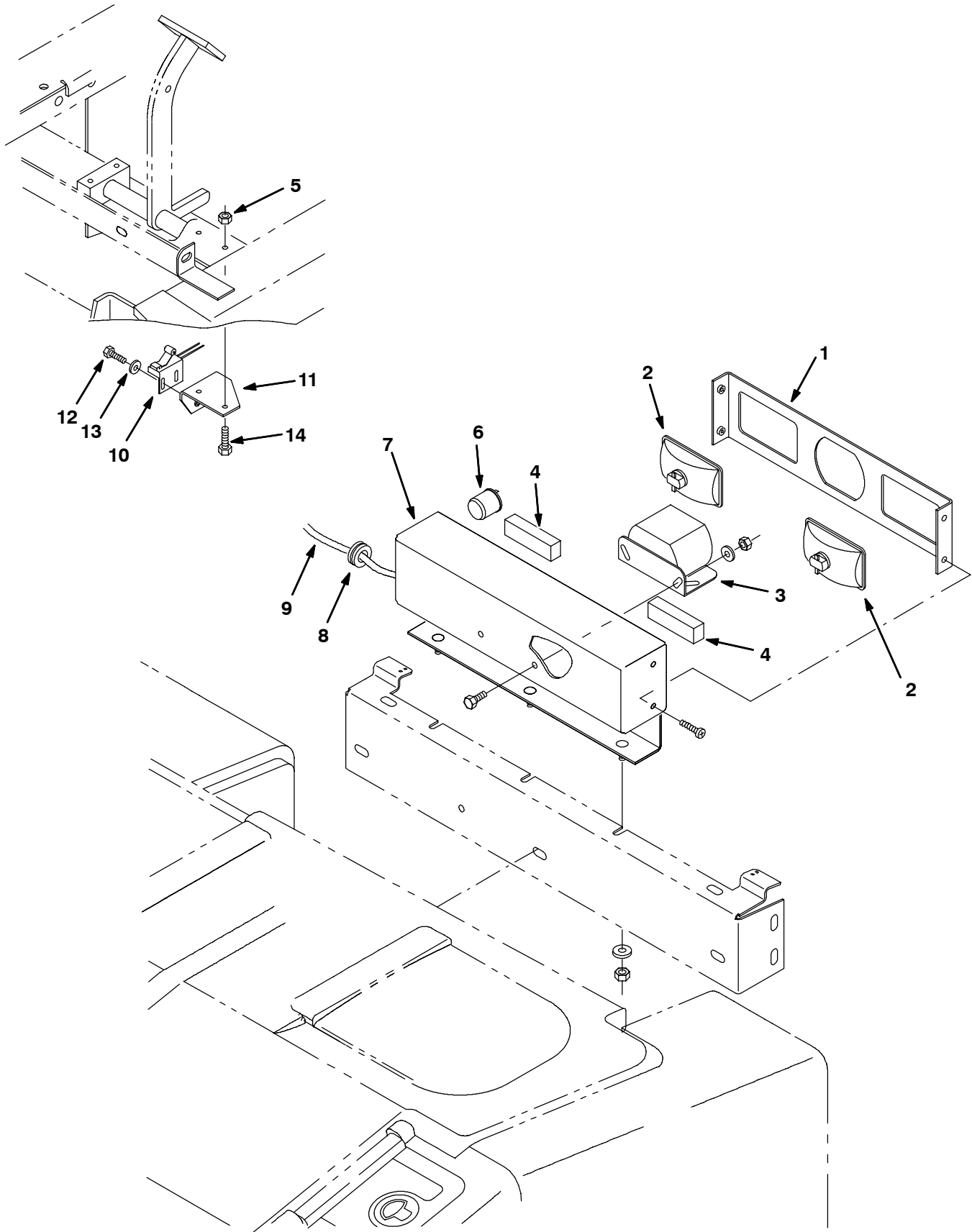
Fig. 5 - Backup Alarm Group - Rückfahr-Alarm-Gruppe - Jeu de pièces alarme de sécurité
