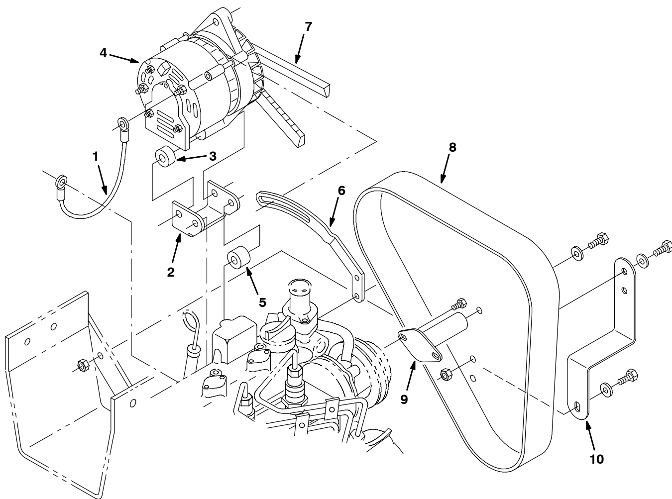
Fig. 16 - Alternator Group - Lichtmaschinen-Gruppe - Assemblage alternateur
