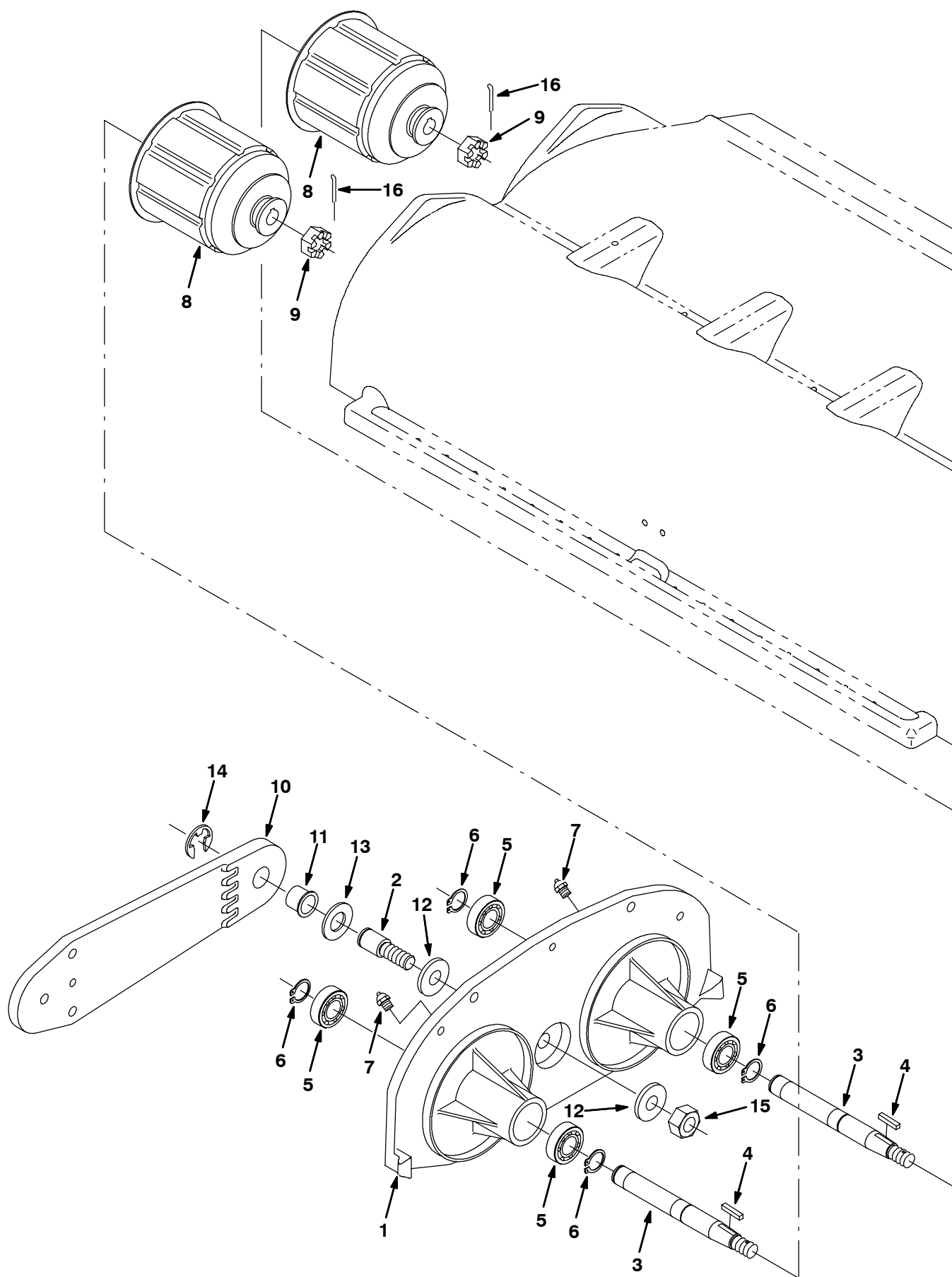
Fig. 47 - Scrub Brush Idler Group - Schrubbbürsten-Spannrollen-Gruppe - Groupe galet-tendeur de brosse dure
