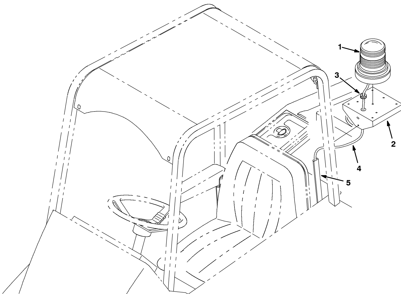
Fig. 1 - Flashing Light Kit, Overhead Guard - Blinklicht-Satz, Überkopf-Schutz - Jeu de pièces gyrophare, protégé-conducteur
