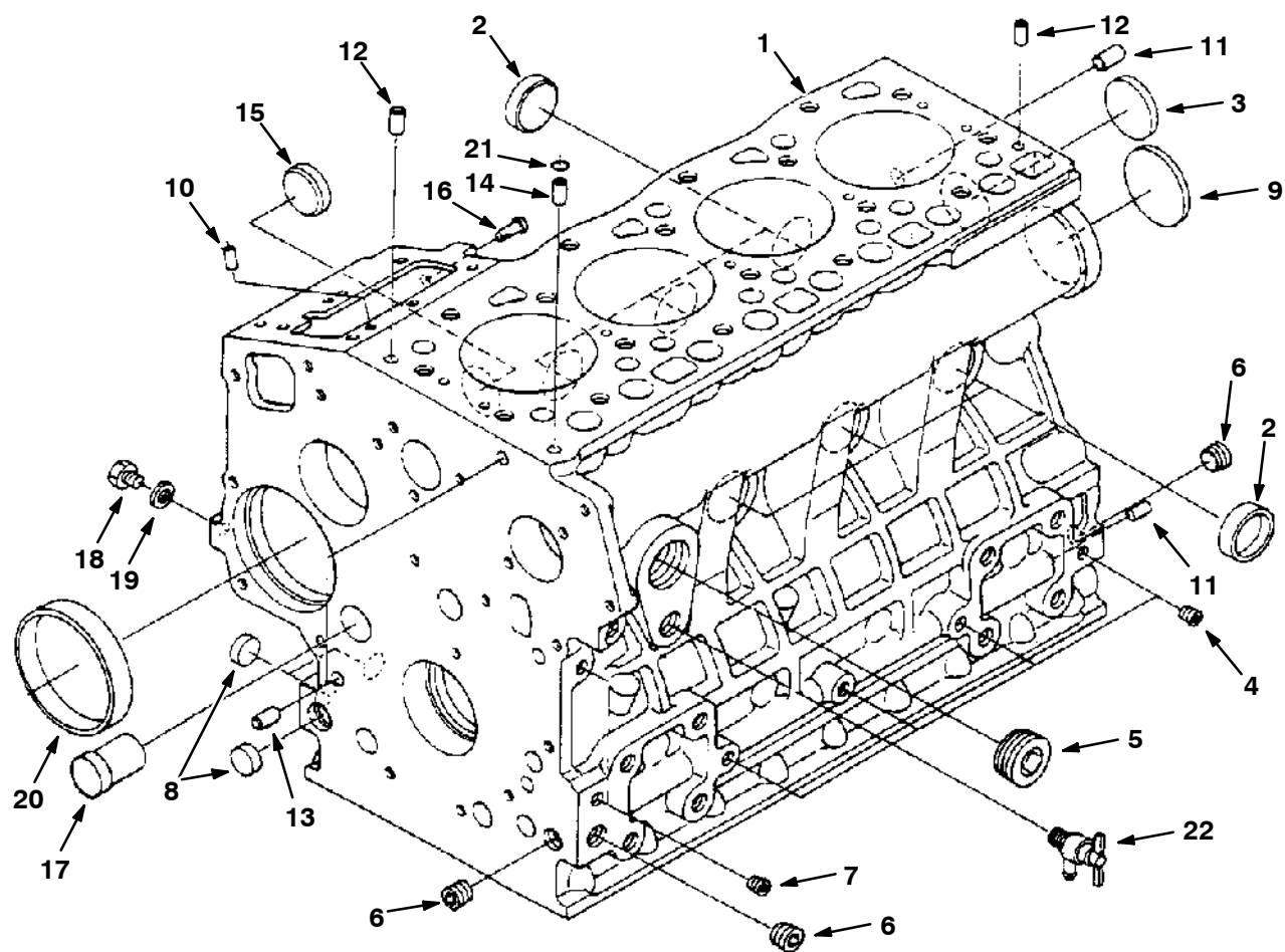
Fig. 1 - Crankcase Group - Kurbelwellen-Gruppe - Assemblage carter de vilebrequin
