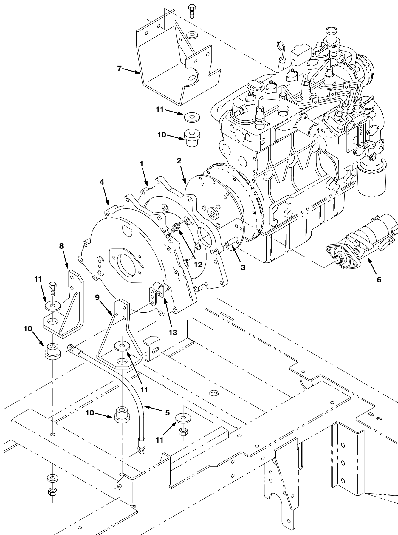
Fig. 14 - Engine Mount Group - Motor-Montage-Gruppe - Assemblage attaches du moteur
