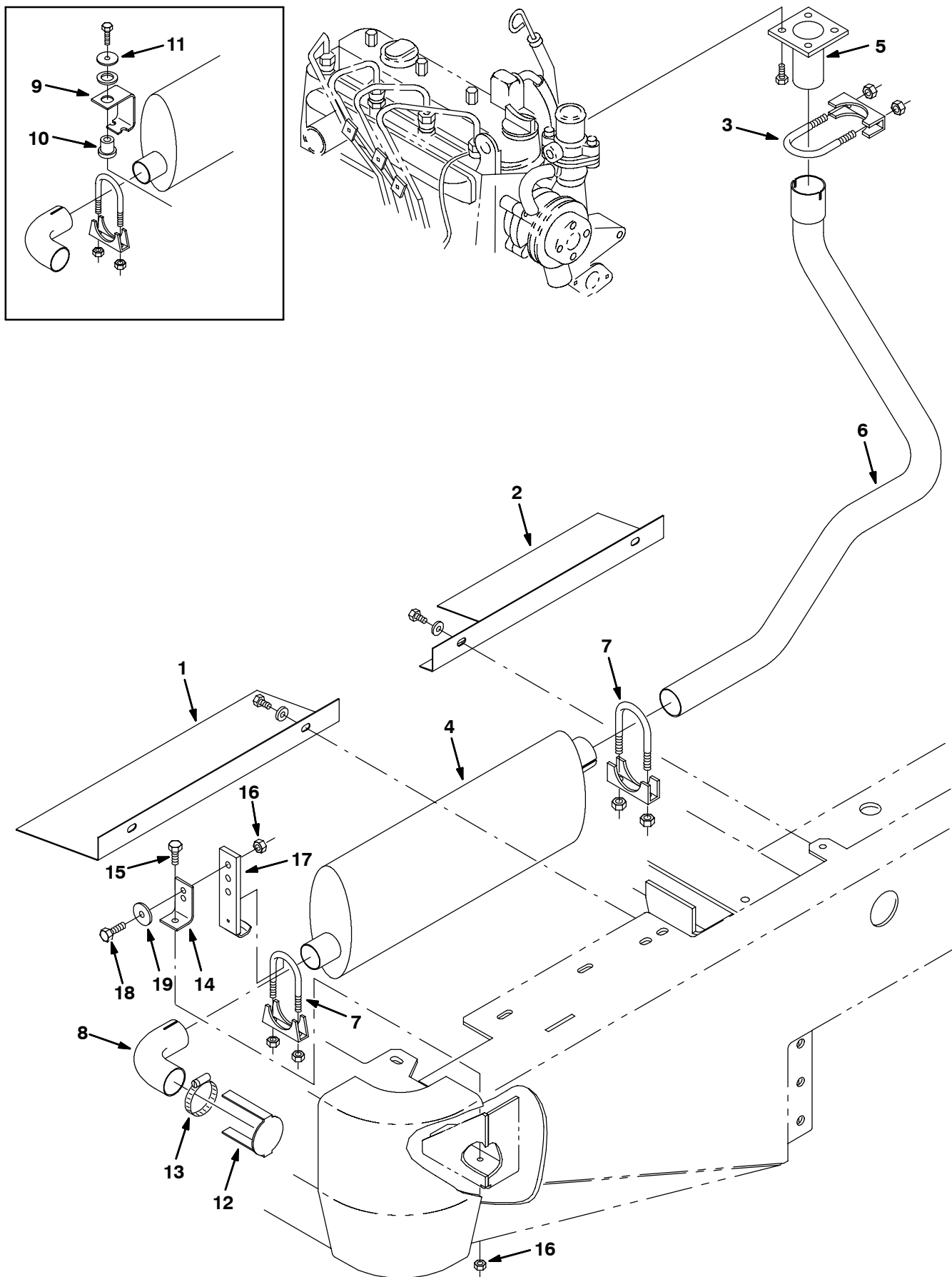
Fig. 17 - Muffler Group - Schalldämpfer-Gruppe - Assemblage silencieux
