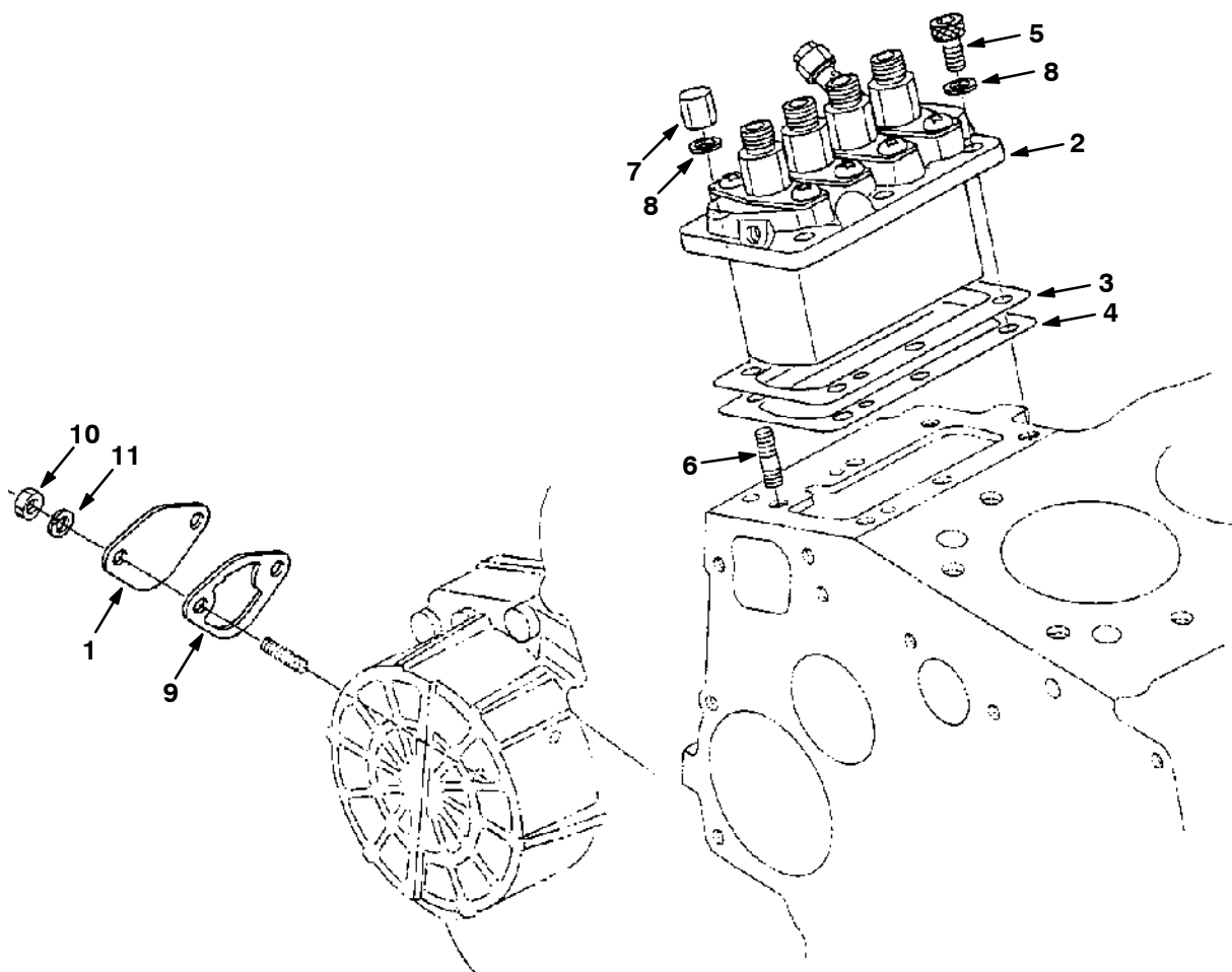
Fig. 15 - Injection Pump Group - Einspritzpumpen-Gruppe - Assemblage pompe à injection
