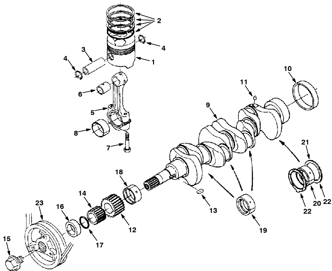
Fig. 11 - Piston and Crankshaft Group - Kolben-/Kurbelwellen-Gruppe - Assemblage pistons et vilebrequin
