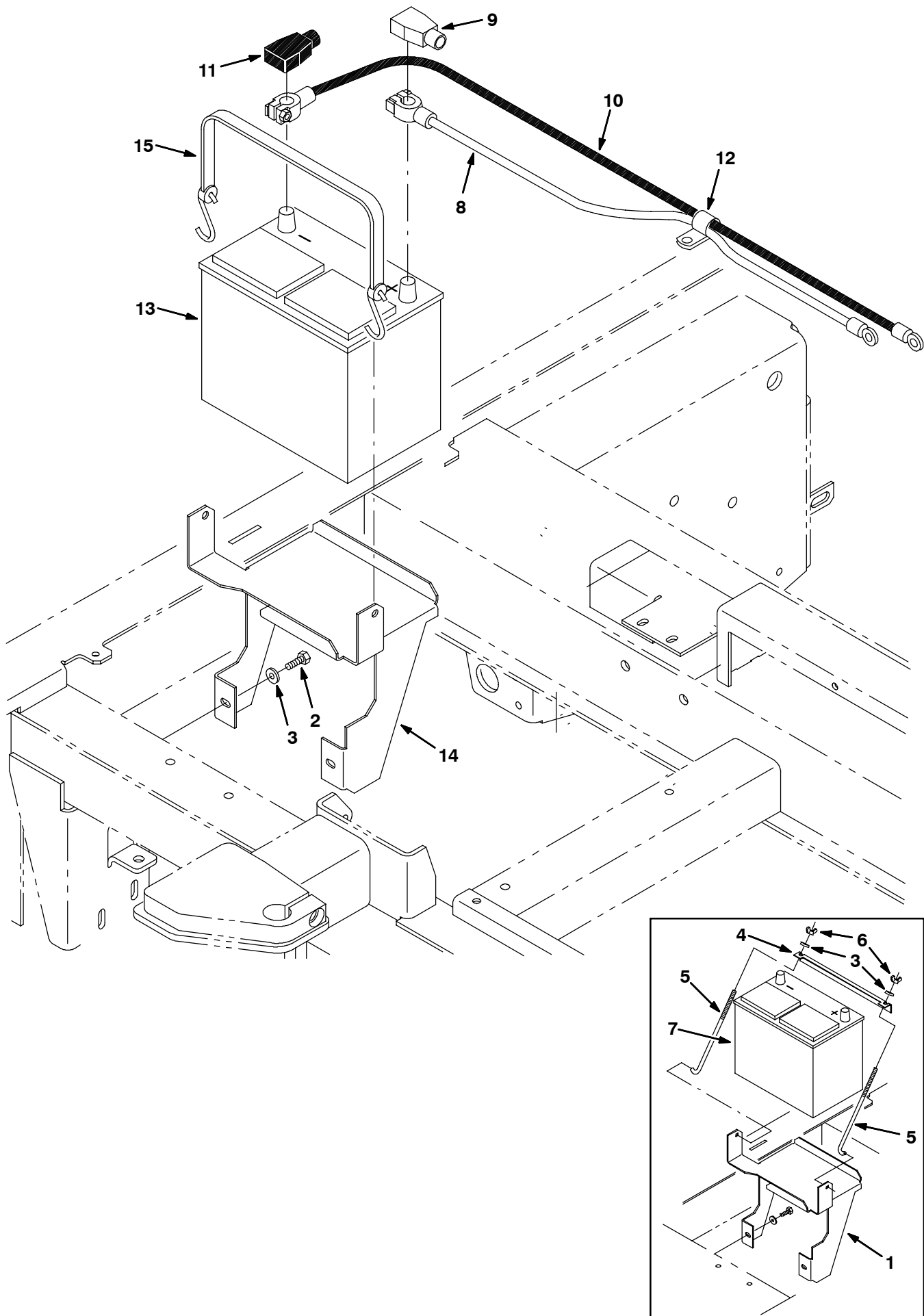
Fig. 21 - Battery Group - Batteriegruppe - Assemblage batterie
