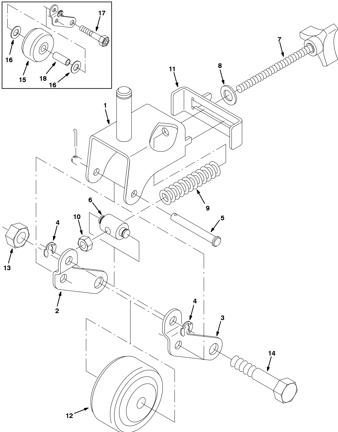
Fig. 54 - Rear Squeegee Caster Assembly - Heck-Abstreifleisten-Rad-Baugruppe - Assemblage roulettes du racloir arrière
