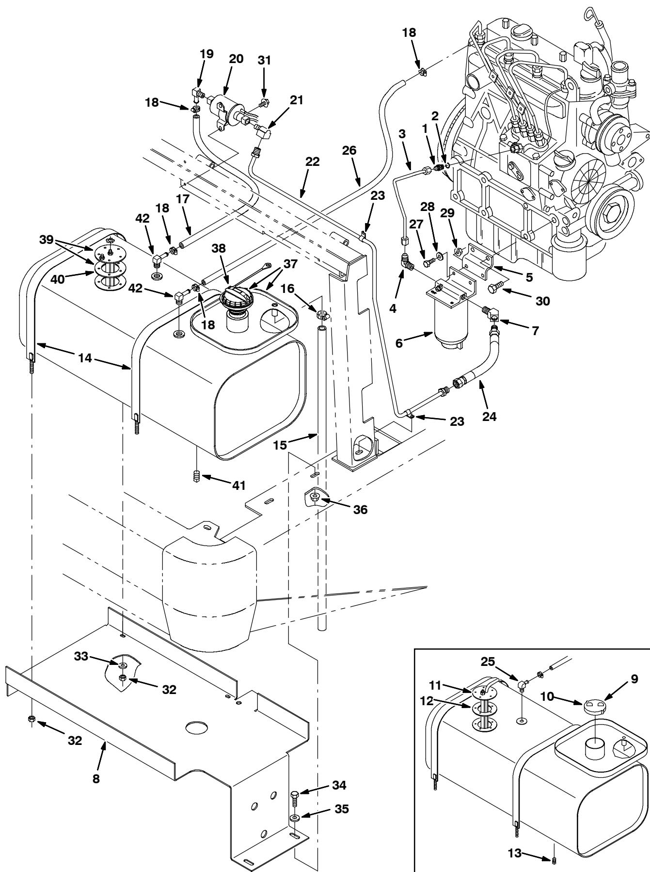
Fig. 18 - Fuel Tank Group - Kraftstofftank Gruppe - Reservoir du carburant
