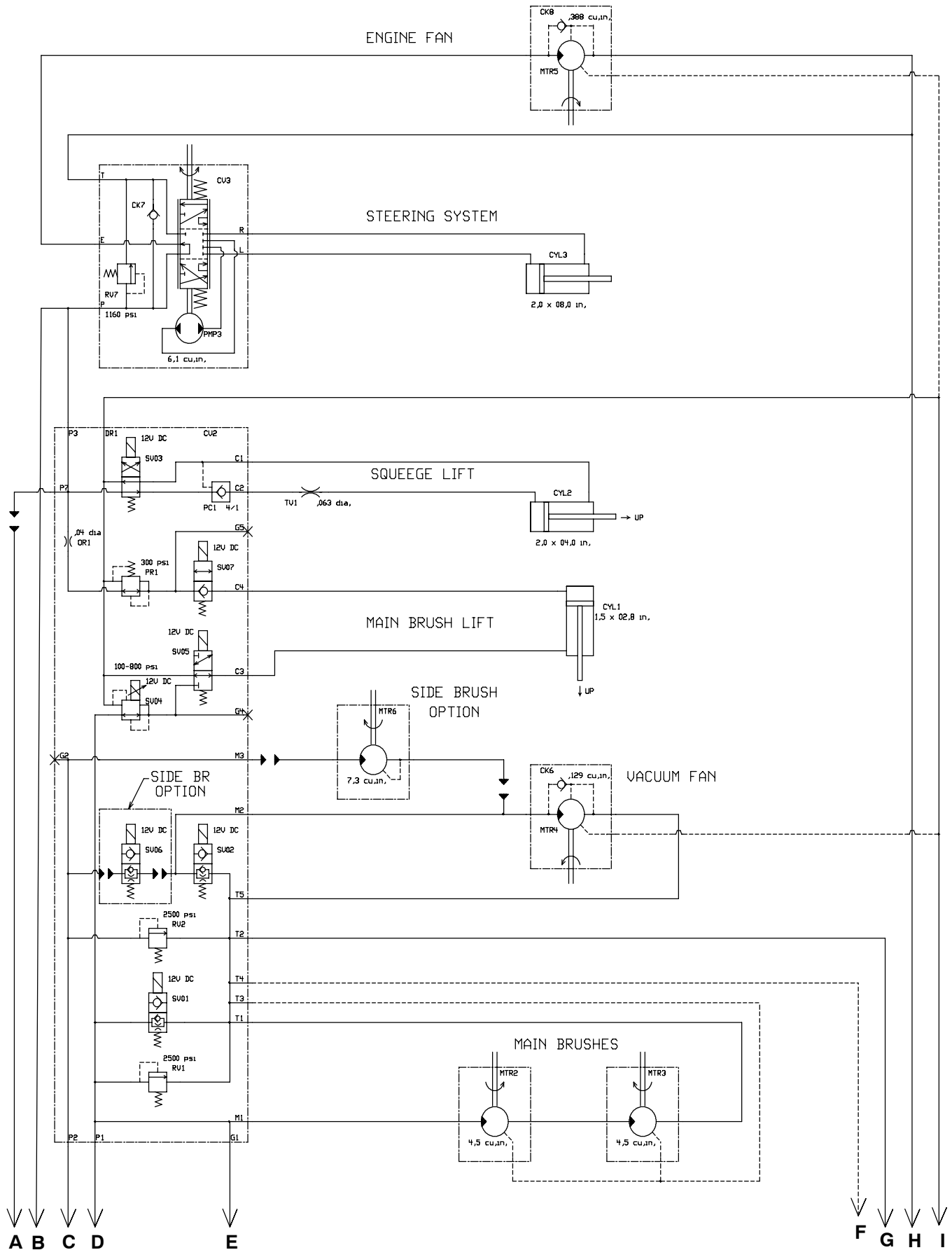
Fig. 33 - Hydraulic Schematic (740045 001-xxx) - Hydraulik-Schema - Schéma du système hydraulique
