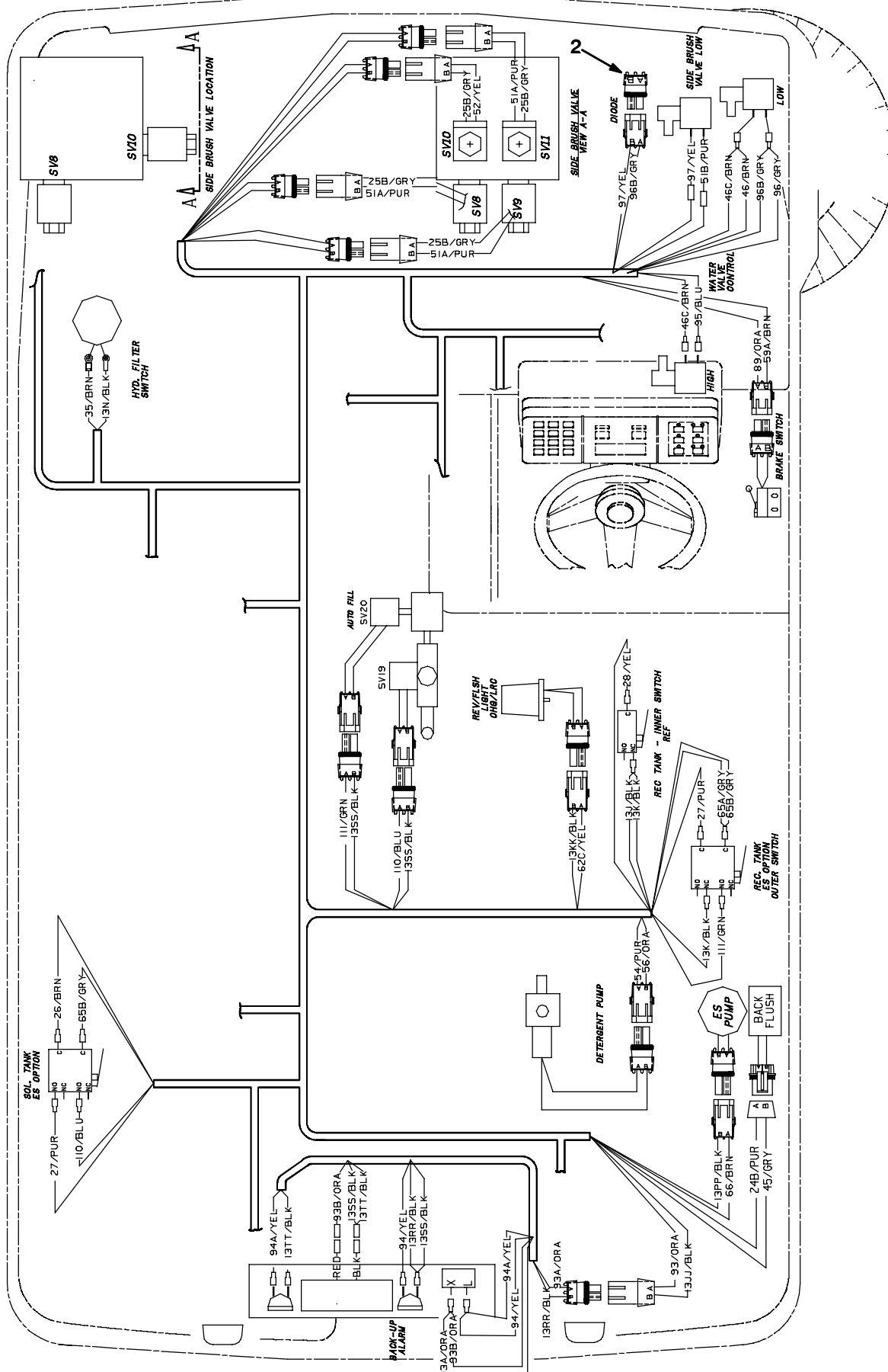
Fig. 42 - Wire Harness Group - Kabelbaum-Gruppe - Assemblage harnais de câbles
