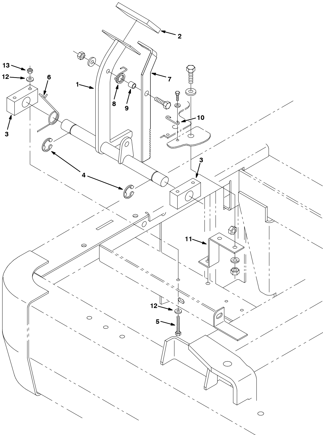
Fig. 24 - Brake Pedal Group - Bremspedal-Gruppe - Assemblage pédale de frein
