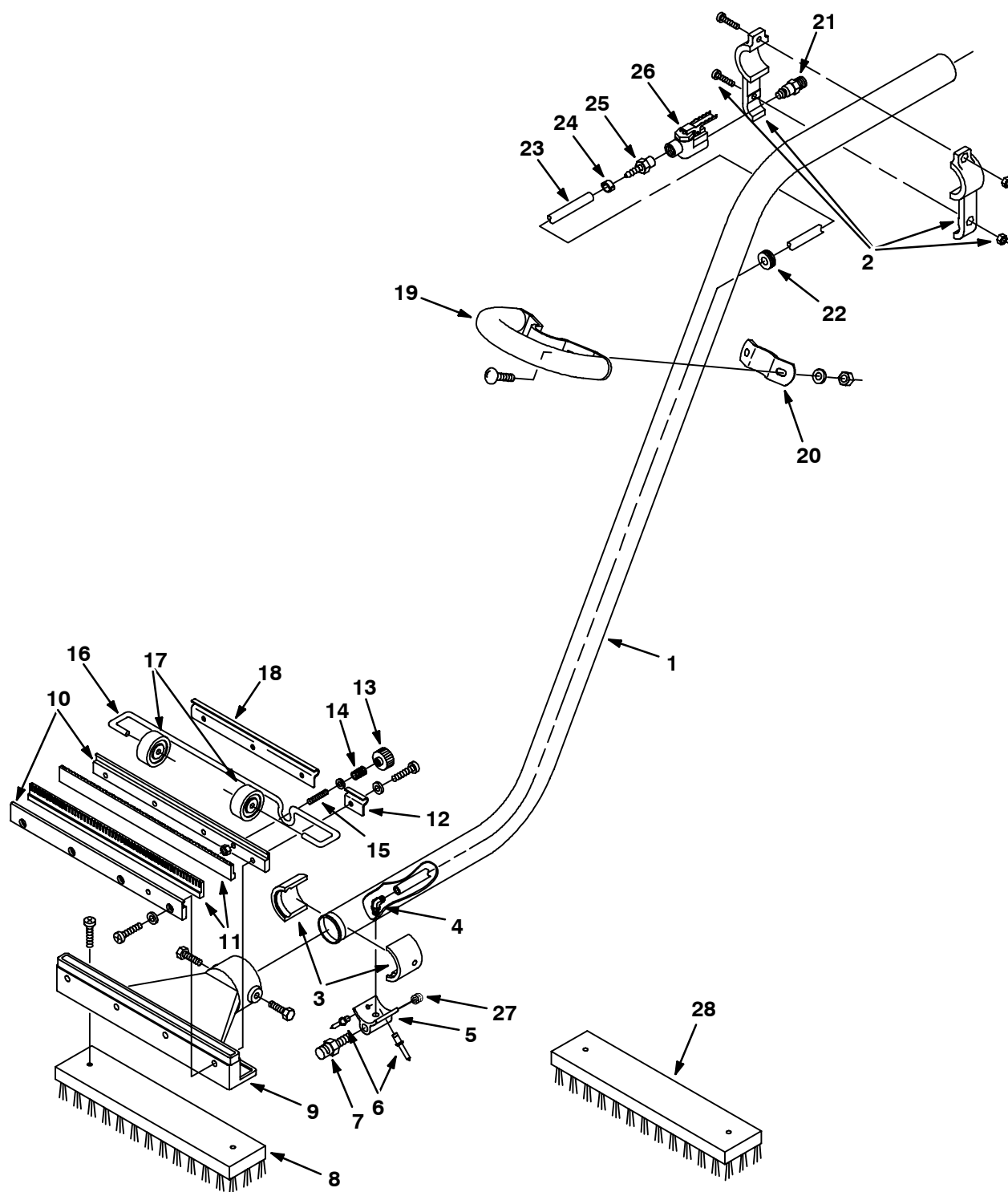
Fig. 19 - Power Wand Assembly - Handschrubber-Baugruppe - Assemblage manche d'aspiration
