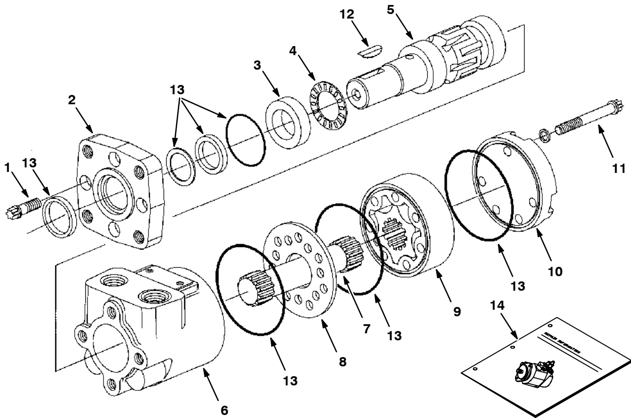
Fig. 8 - Hydraulic Motor Breakdown, 397692 - Hydraulik-Motor-Defekt - Panne de moteur hydraulique, 397692
