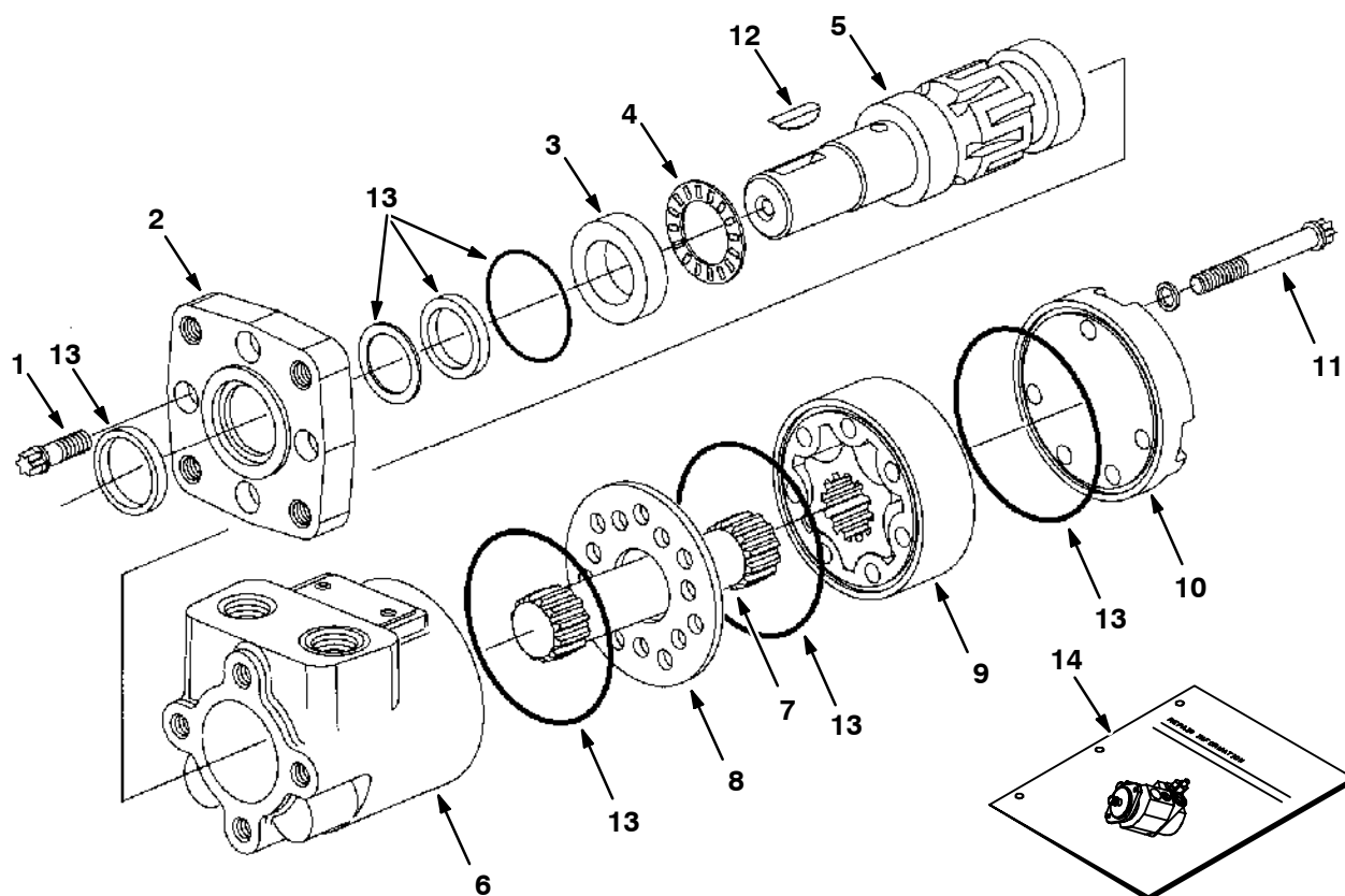
Fig. 6 - Hydraulic Motor Breakdown, 71722 - Hydraulik-Motor-Defekt - Panne de moteur hydraulique, 71722
