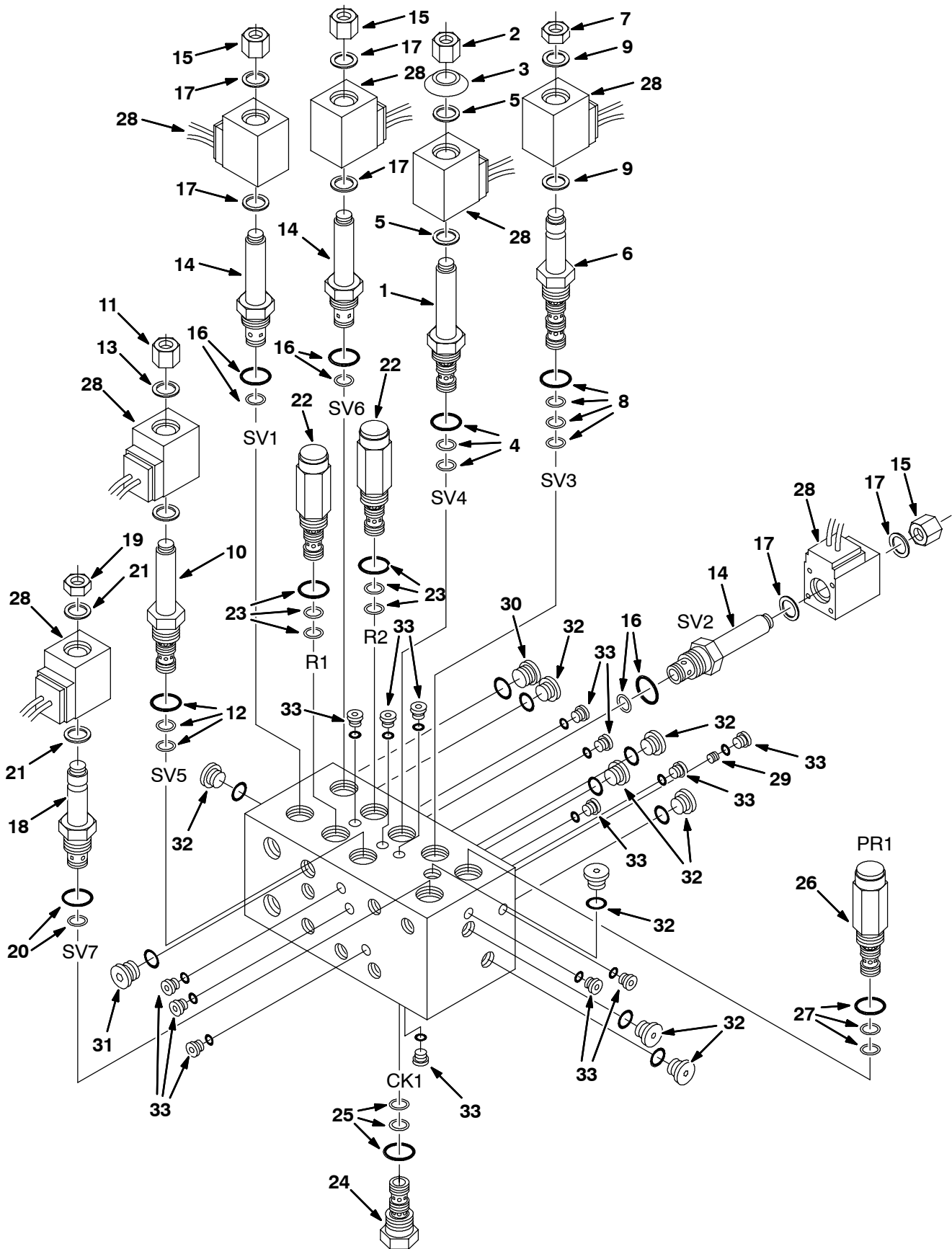
Fig. 13 - Hydraulic Solenoid Valve Breakdown, 71760 - Hydraulik-Magnetventil-Defekt - Panne de soupape magnétique hydraulique, 71760
