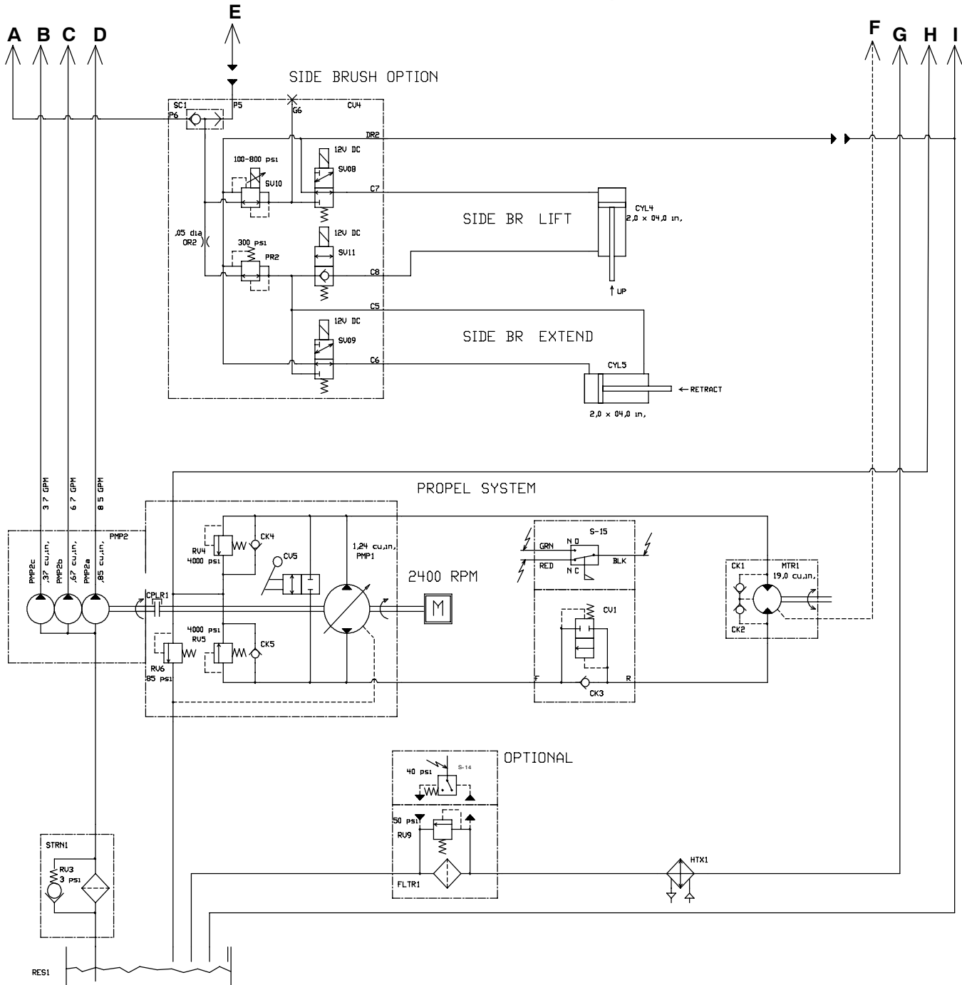
Fig. 33 - Hydraulic Schematic (740045 001-xxx) - Hydraulik-Schema - Schéma du système hydraulique
