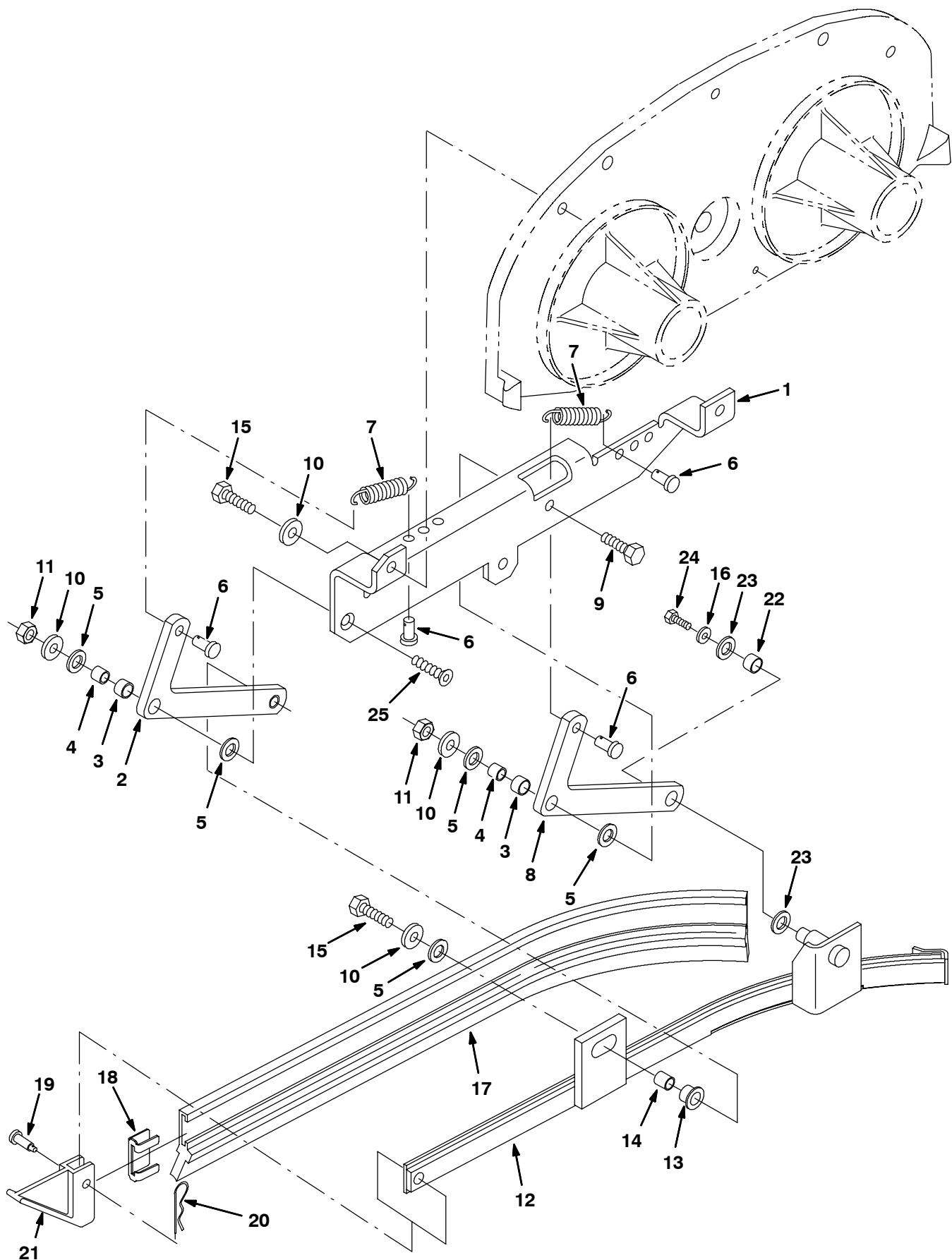
Fig. 48 - Right Side Squeegee Group - Rechte Abstreifleisten-Gruppe - Assemblage racloir droit
