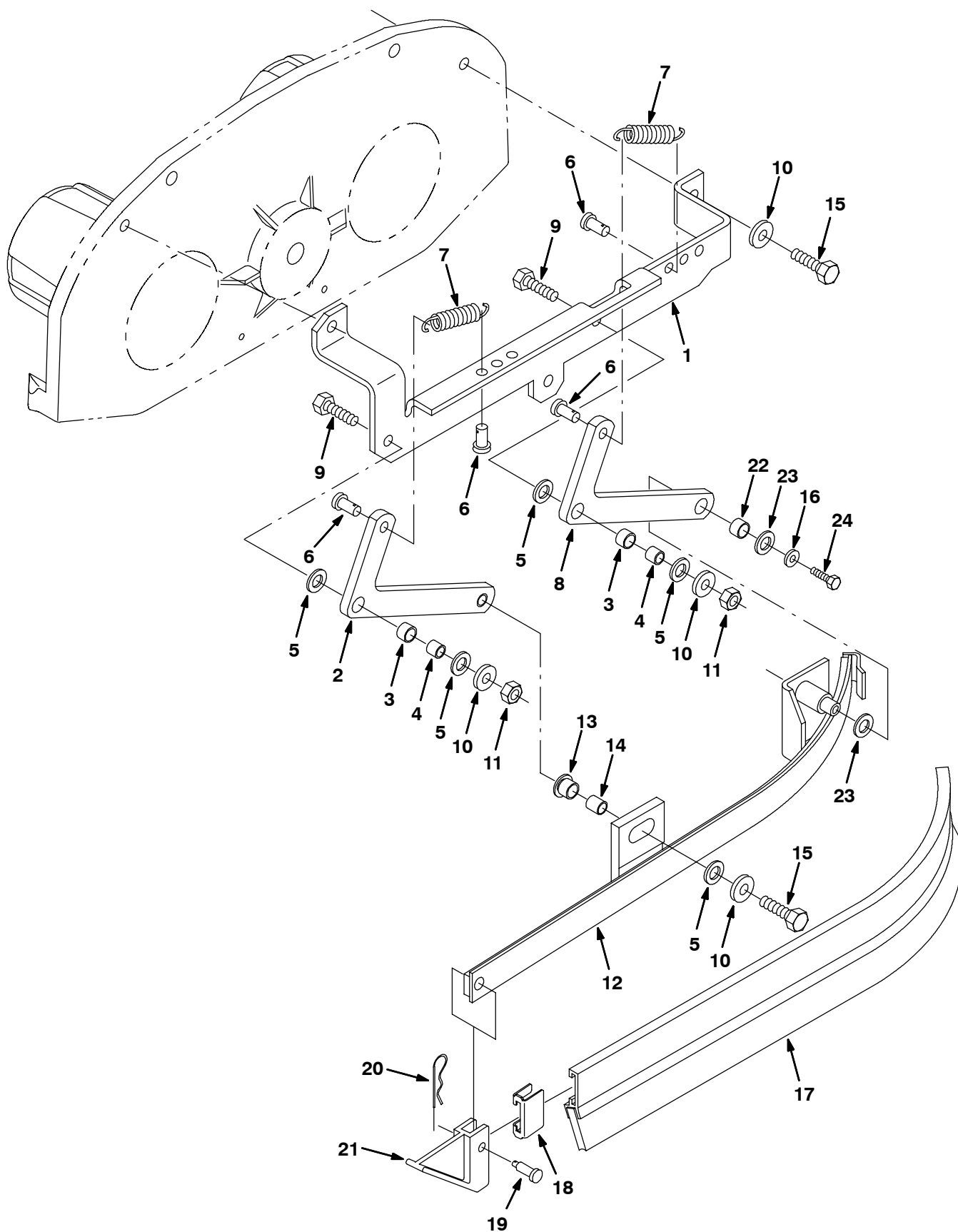
Fig. 46 - Left Side Squeegee Group - Linke Abstreifleisten-Gruppe - Assemblage racloir gauche
