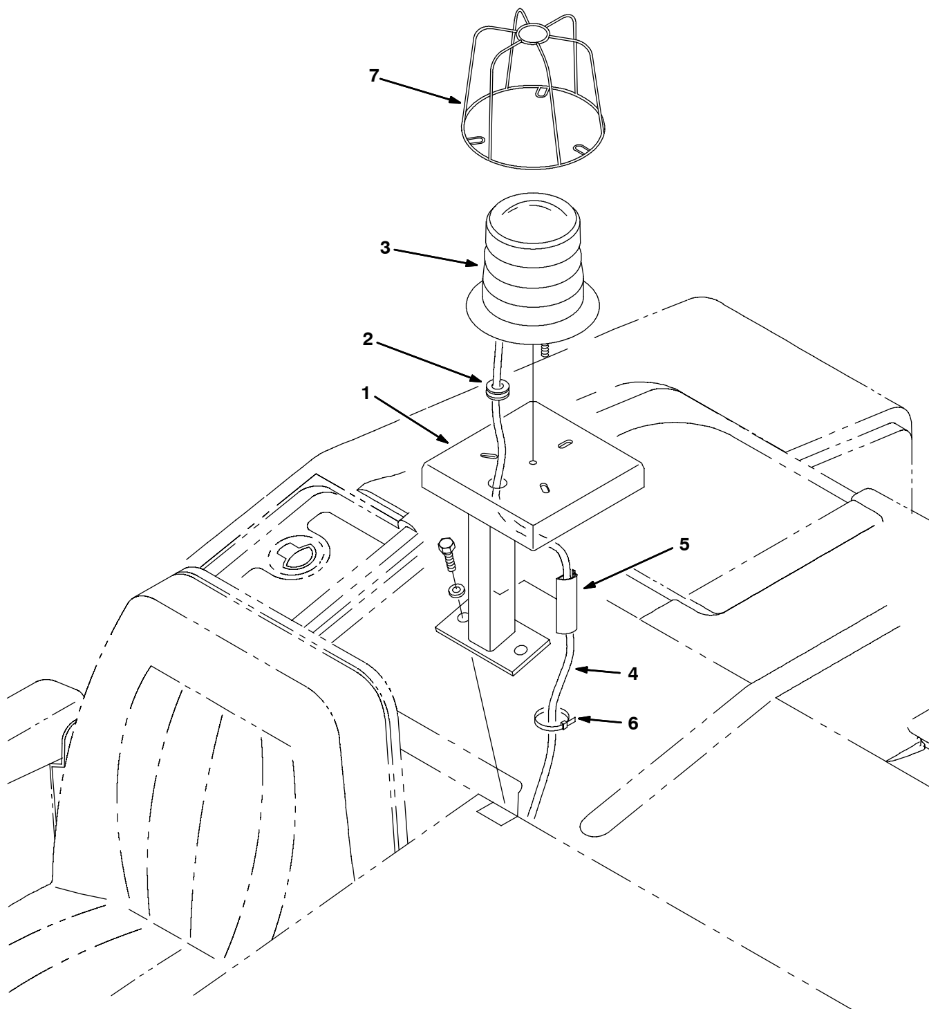
Fig. 3 - Flashing Light Kit, LRC - Blinklicht-Satz LRC - Jeu de pièces gyrophare, côtés droit et gauche
