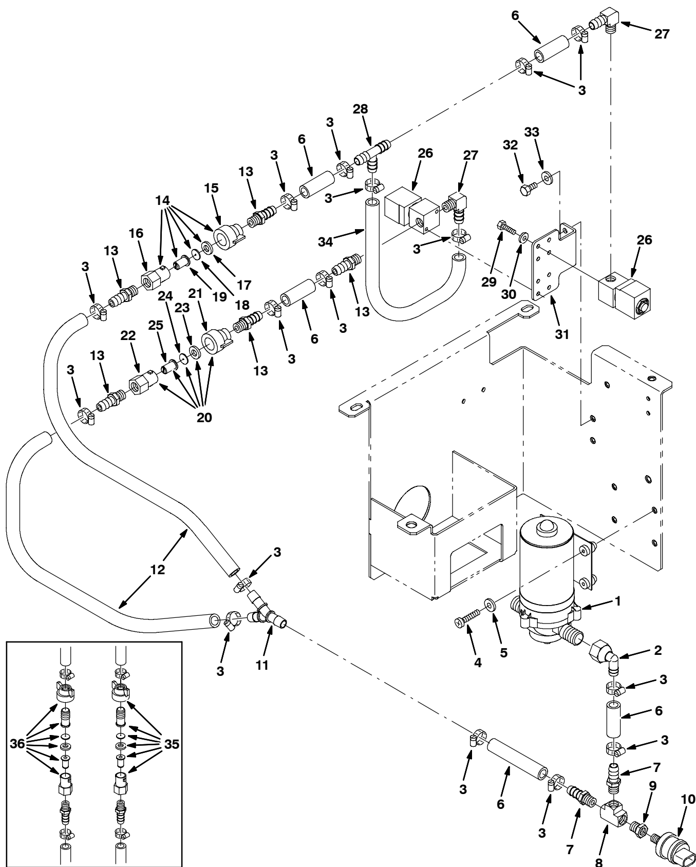
Fig. 68 - FaST Solution Pump Group — FaST Frischwasserpumpen-Gruppe — Groupe pompe à solution FaST
