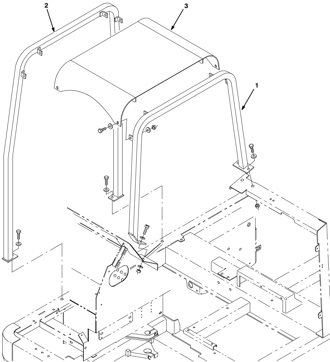
Fig. 6 - Overhead Guard Kit - Überkopf-Schutz-Satz - Jeu de pièces protège-conducteur
