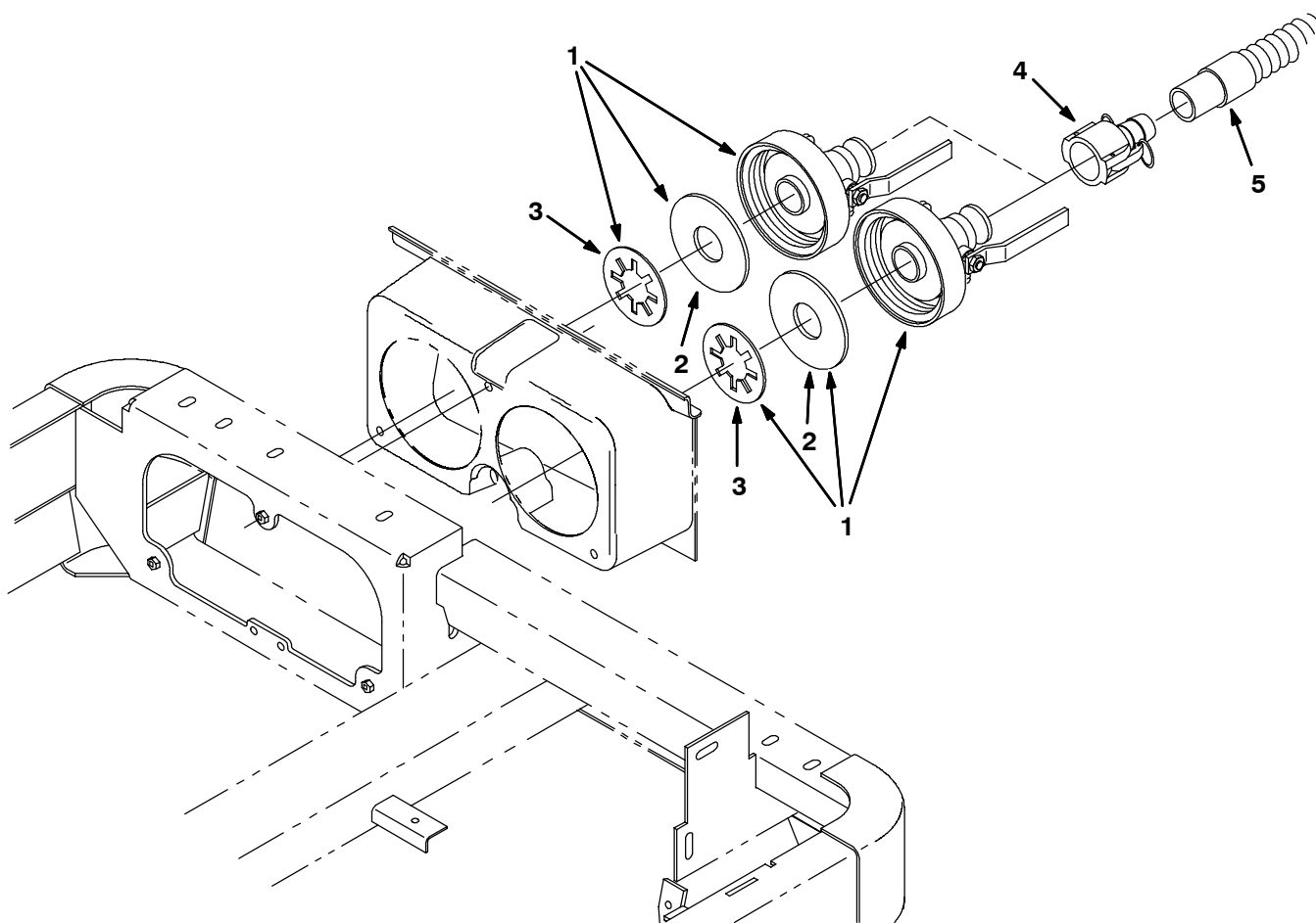
Fig. 20 - Positive Solution Control Drain Kit, ES - Satz Kontrollierte Frischwassertankentleerung/ES - Jeu de pièces système de vidange à système de contrôle de la solution, ES
