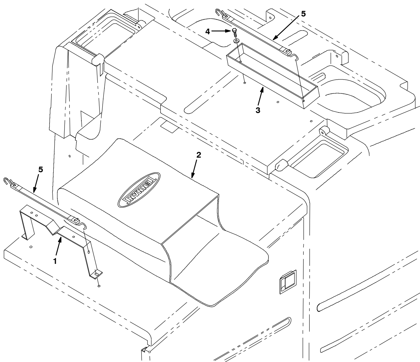
Fig. 17 - Power Wand Mount Group - Handschrubbarm Montage Gruppe - Groupe Montage de la Laveuse à Main
