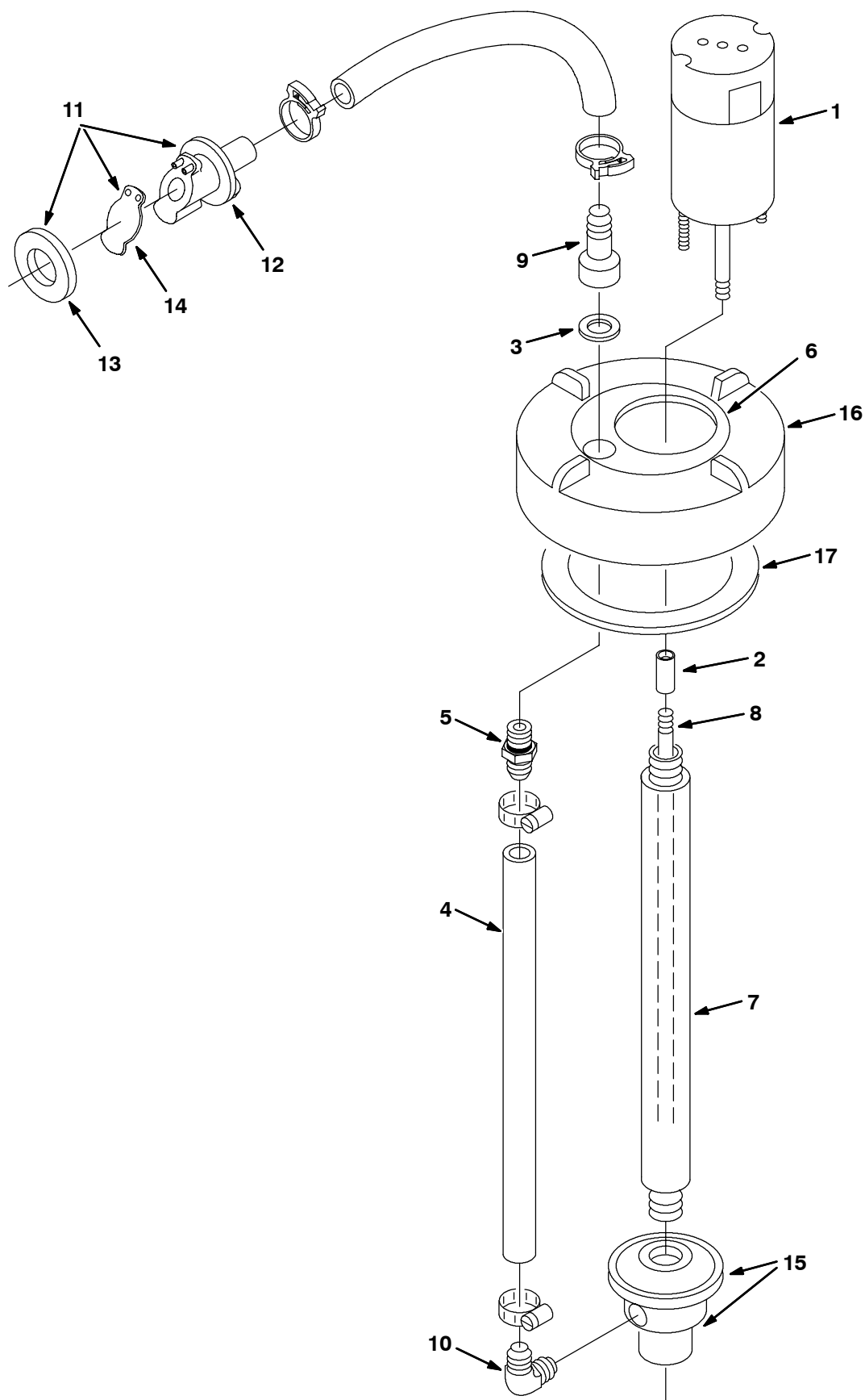
Fig. 18 - Extended Scrub Pump Breakdown, 379005 - Defekt Verlängerter Schrubbetrieb-Pumpe - Panne de pompe du système de nettoyage prolongé, 370005
