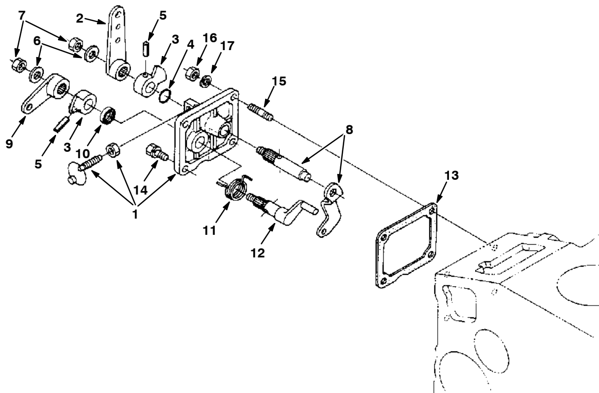
Fig. 19 - Speed Control Plate Group - Drehzahlsteuerungs-Gruppe - Assemblage plaque de régulation de vitesse
