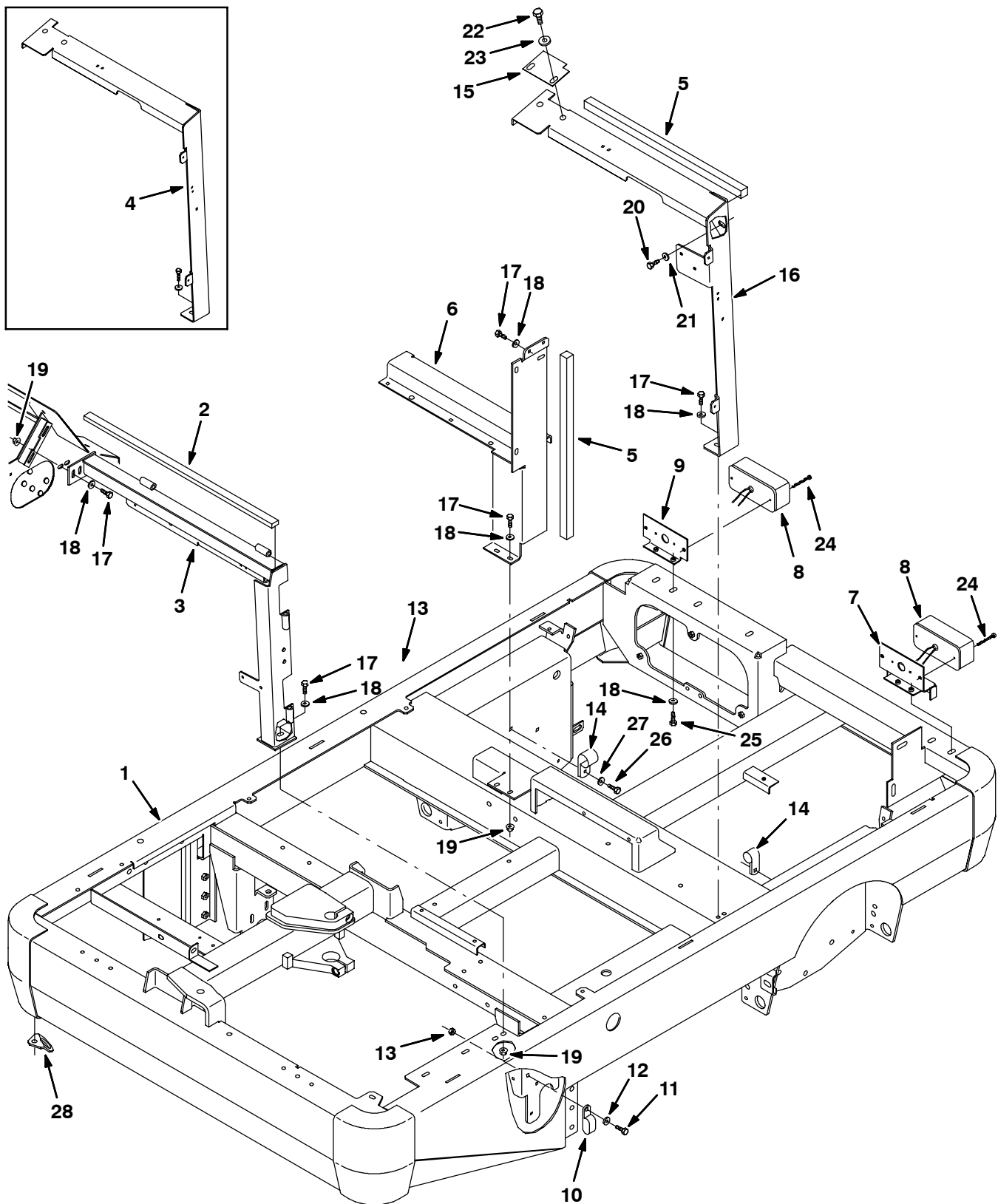
Fig. 3 - Mainframe Group - Hauptfahrgestell-Gruppe - Assemblage châssis
