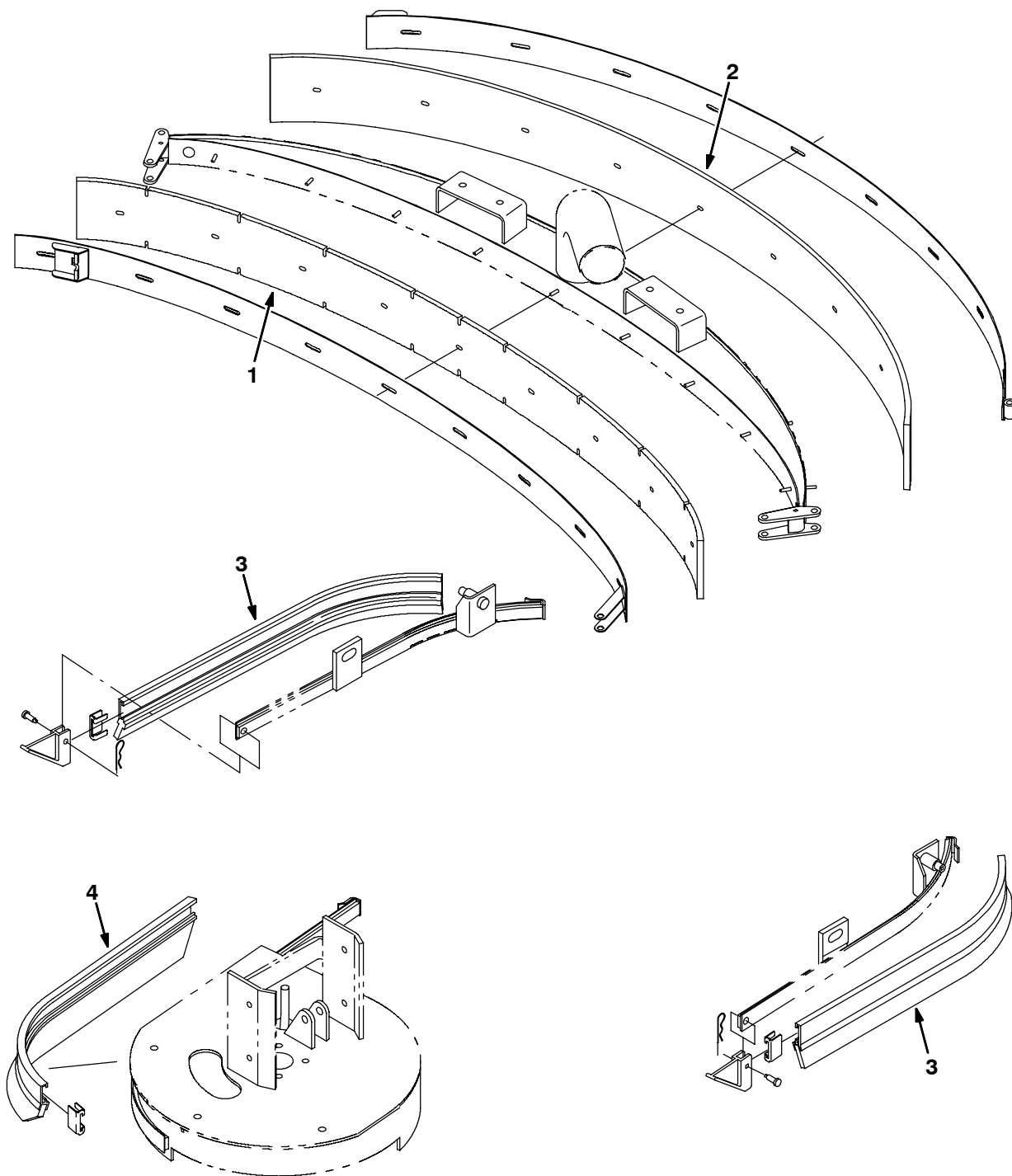
Fig. 14 - Urethane Squeegee Blade Kit - Urethan-Abstreifleisten-Wischgummi-Satz - Jeu de pièces lame de racloir en uréthane
