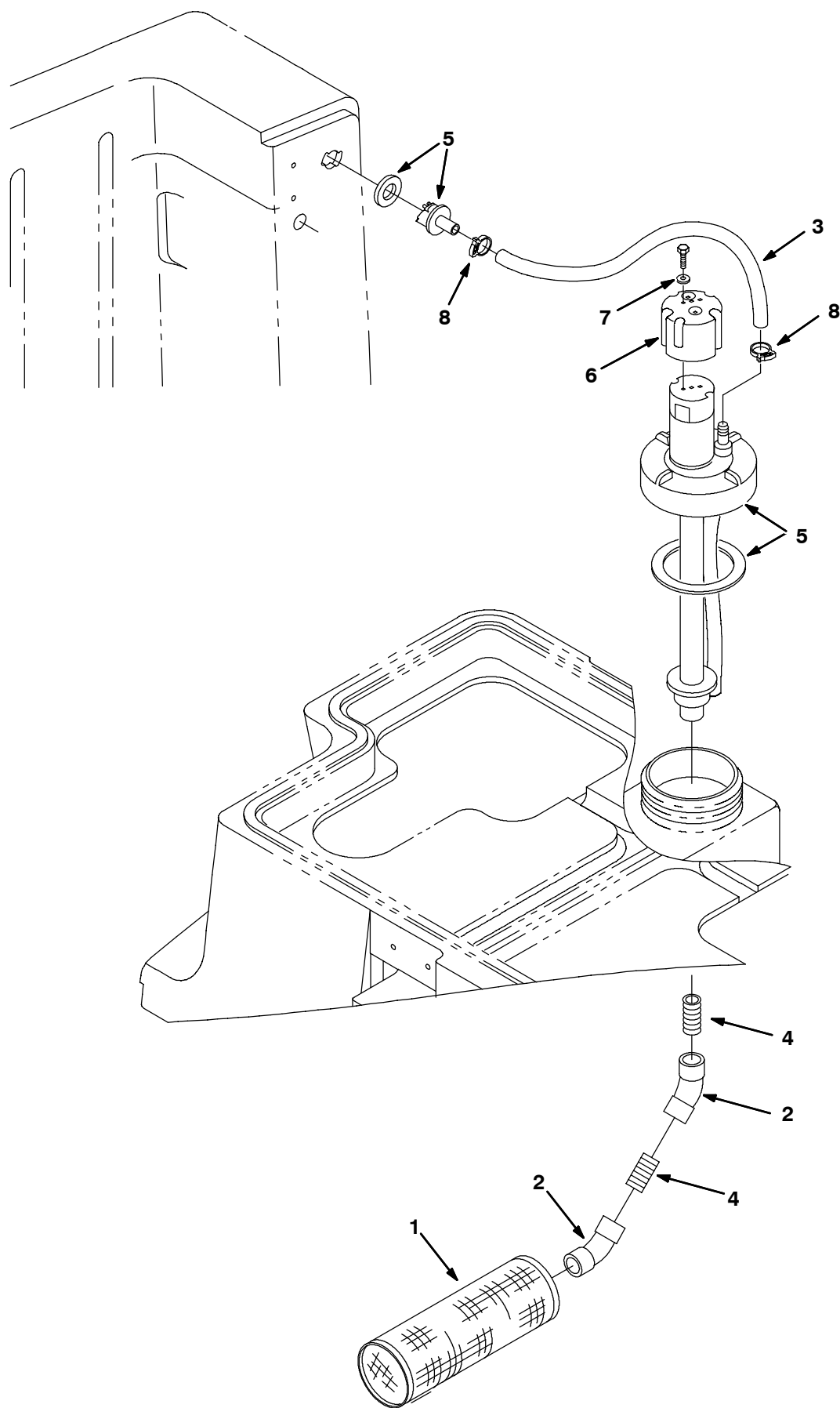
Fig. 56 - ES Pump Column Group (740045 001-074) - ES-Pumpensäulen-Gruppe - Assemblage colonne de pompage ES
