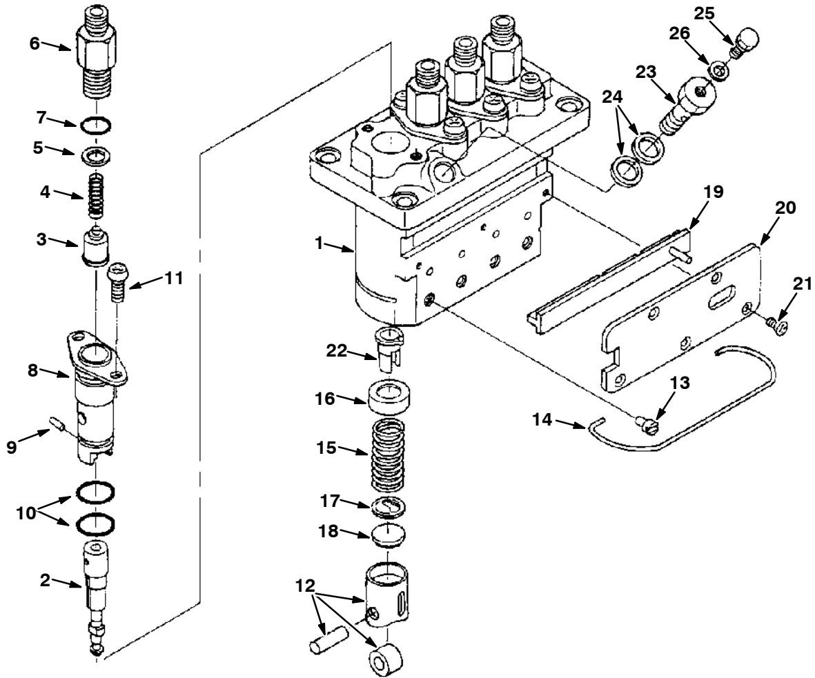
Fig. 16 - Injection Pump Breakdown - Einspritzpumpen-Defekt - Panne pompe à injection
