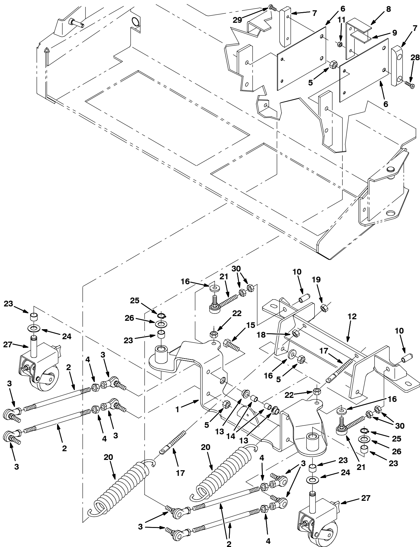
Fig. 52 - Rear Squeegee Linkage Group - Heck-Abstreifleisten-Gestänge-Gruppe - Assemblage timonerie du racloir arrière
