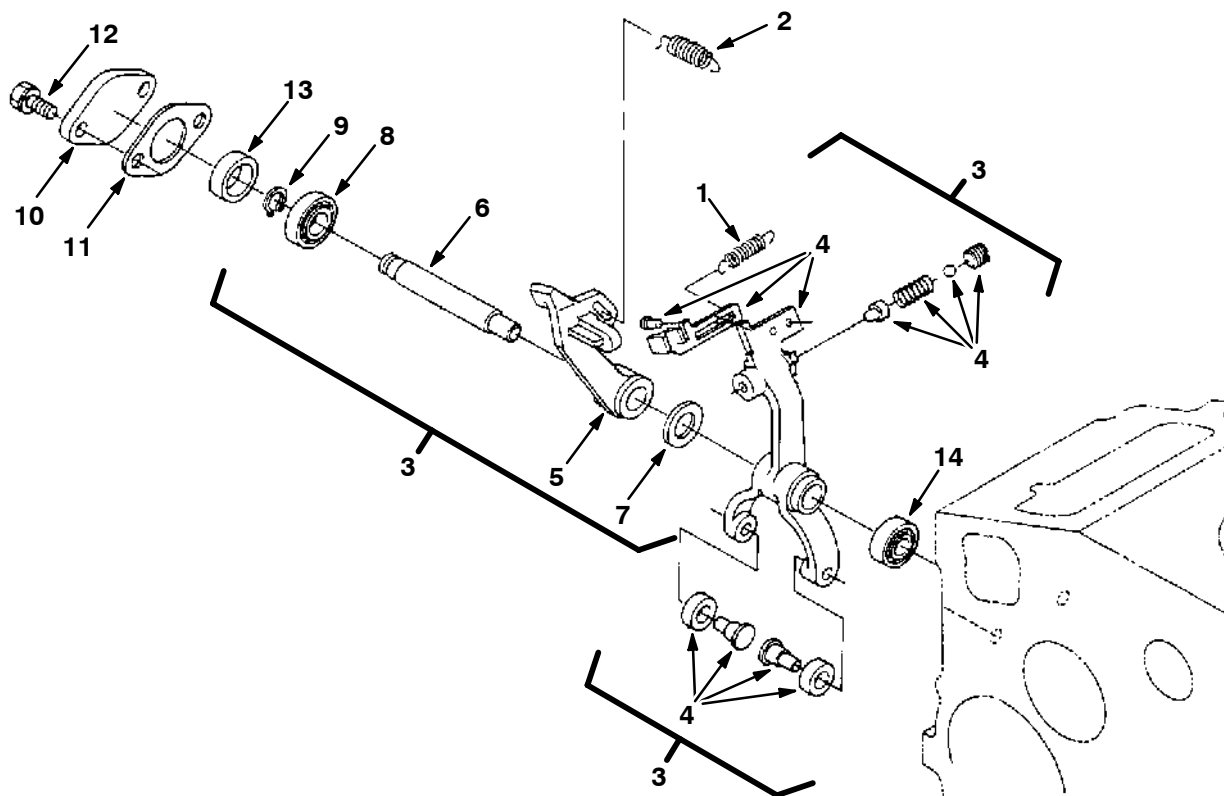
Fig. 20 - Governor Group - Regler-Gruppe - Assemblage régulateur
