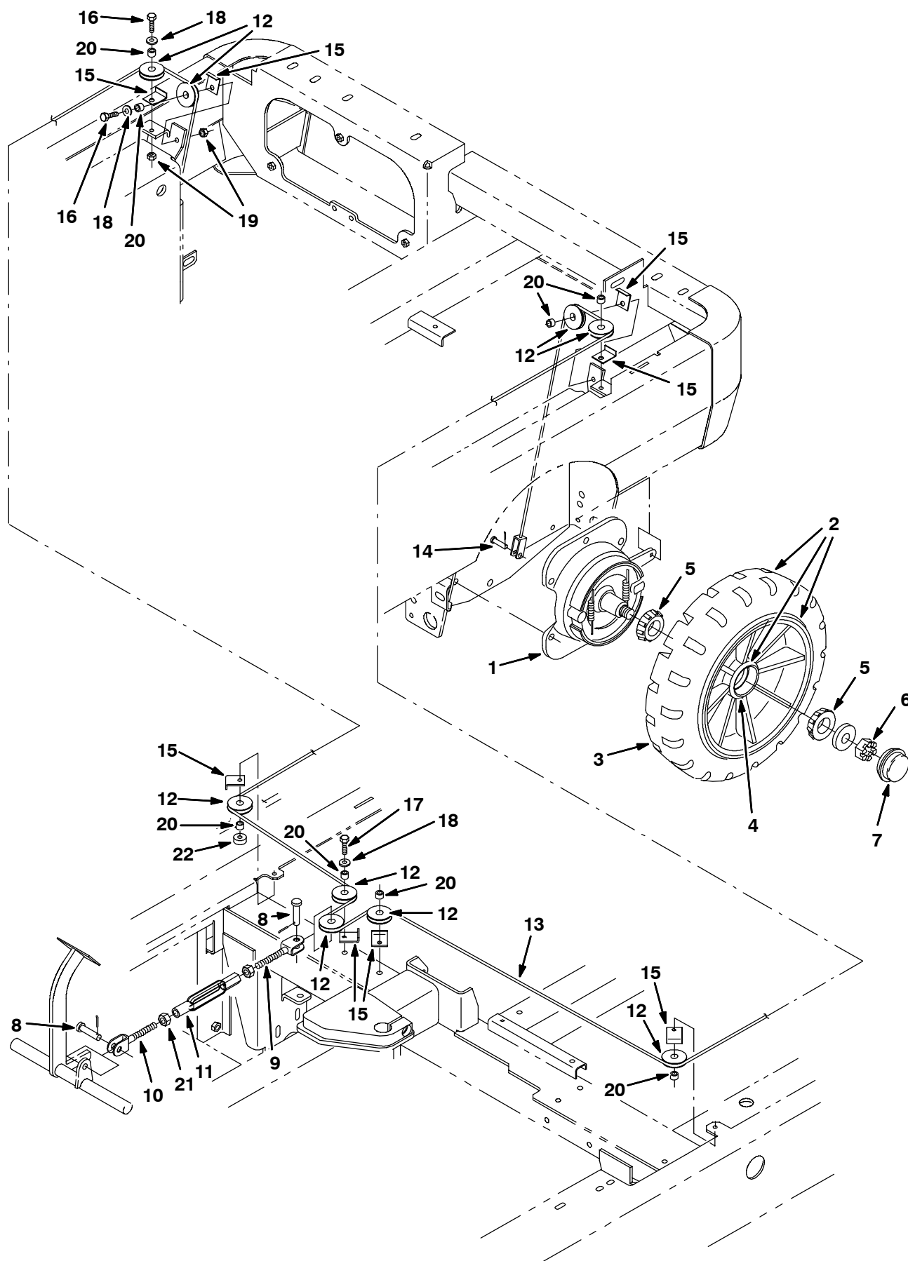
Fig. 23 - Rear Wheels and Brakes Group - Heck-Räder-/Bremsen-Gruppe - Assemblage freins et roues arrière
