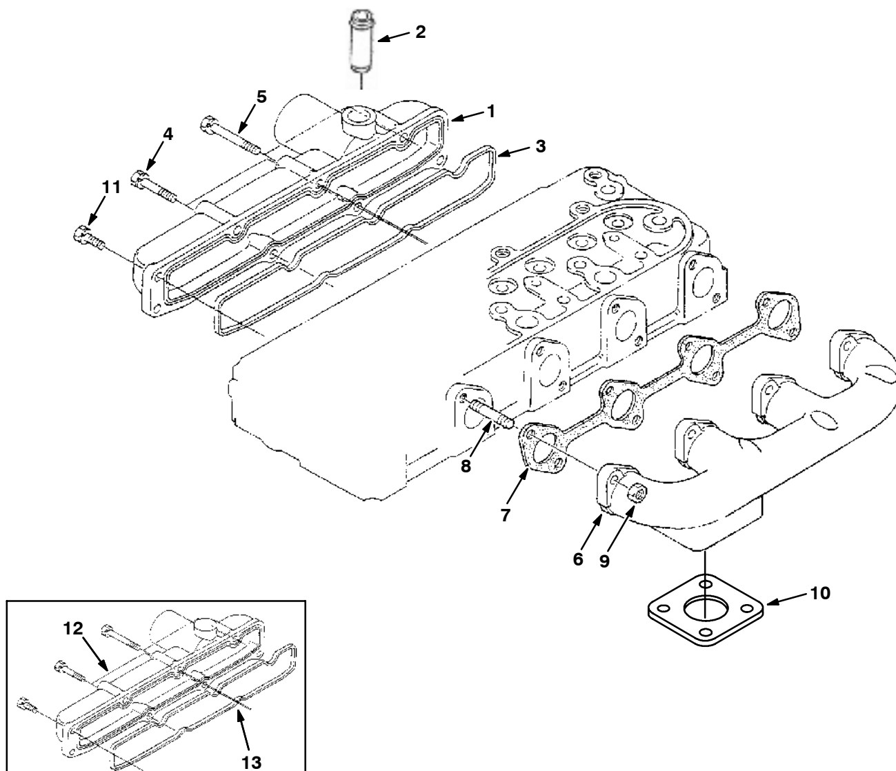
Fig. 8 - Manifold Group - Krümmergruppe - Assemblage collecteur
