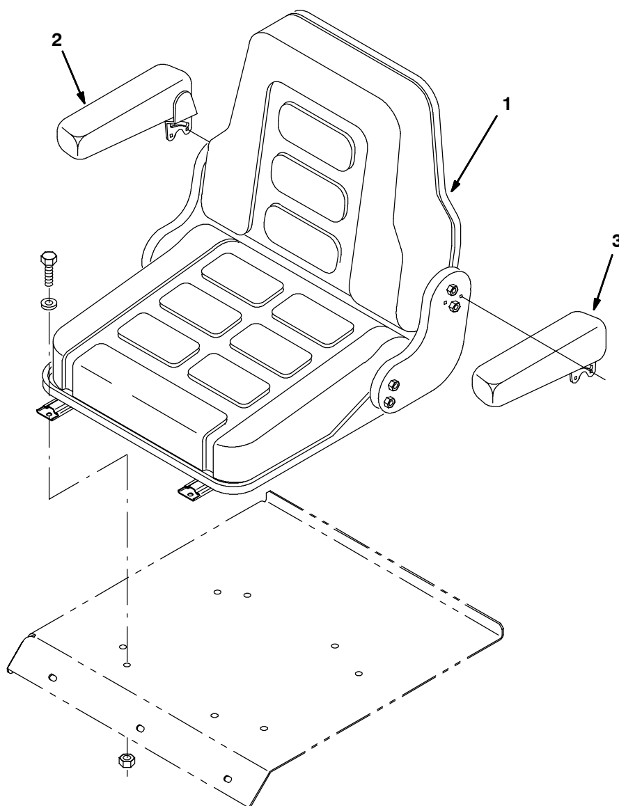
Fig. 9 - Driver Seat Kit - Fahrersitz-Satz - Jeu de pièces siège du conducteur
