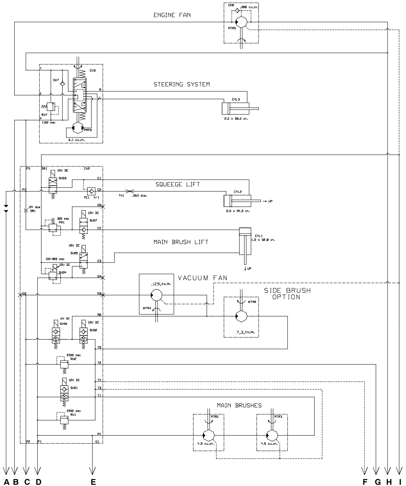
Fig. 34 - Hydraulic Schematic (740045 xxx- ) - Hydraulik-Schema - Schéma du système hydraulique
