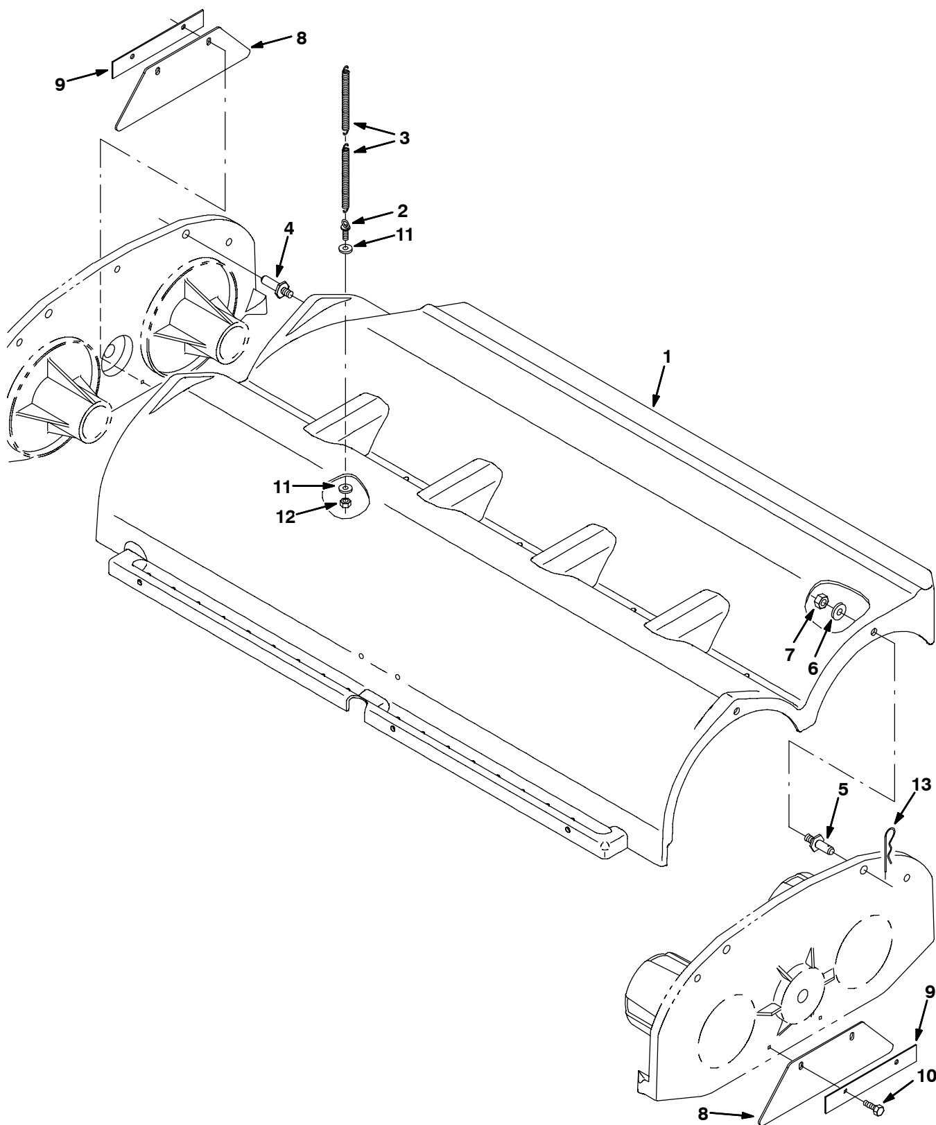
Fig. 44 - Scrub Brush Housing Group - Schrubbürsten-Gehäuse-Gruppe - Groupe boîtier de brosse
