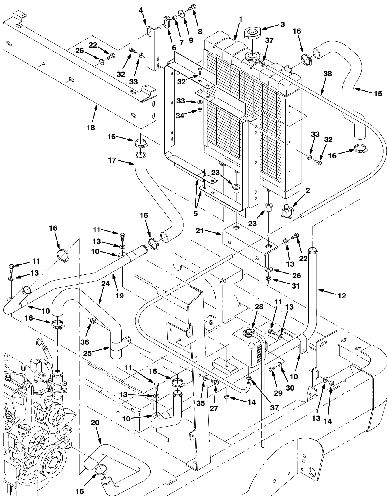
Fig. 19 - Radiator Group - Kühlergruppe - Assemblage radiateur
