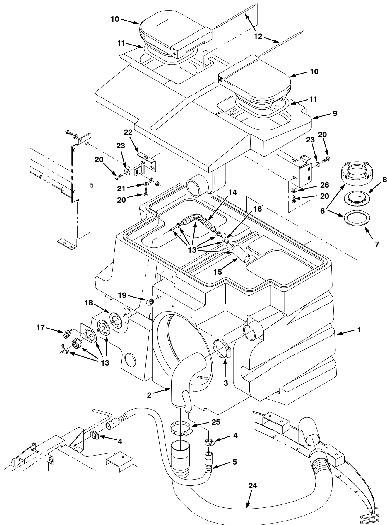
Fig. 30 - Recovery Tank Group - Schmutzwasser-Tankgruppe - Assemblage réservoir de récupération
