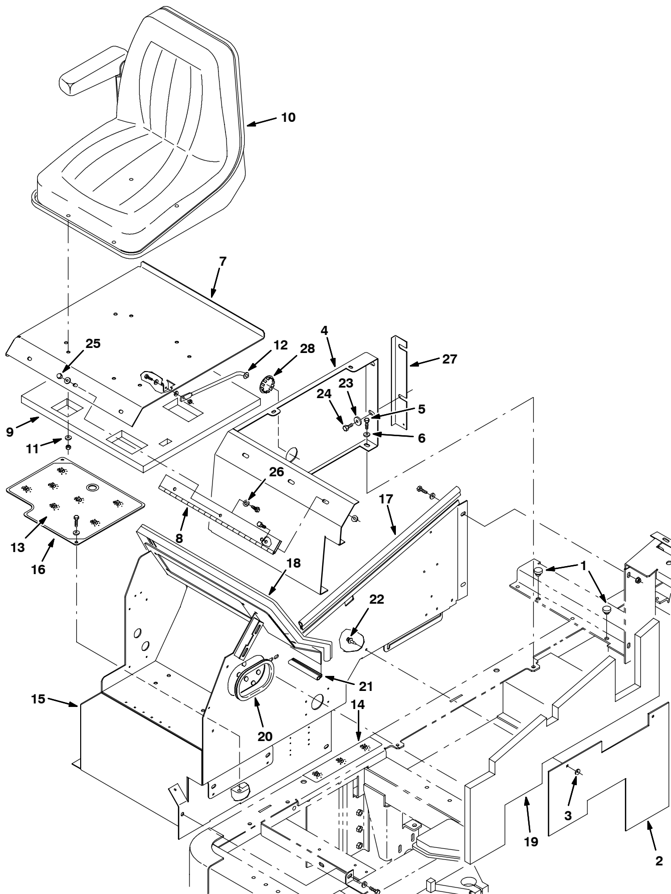
Fig. 5 - Seat and Shroud Group - Sitz- und Abschirmblech-Gruppe - Assemblage siège et protection
