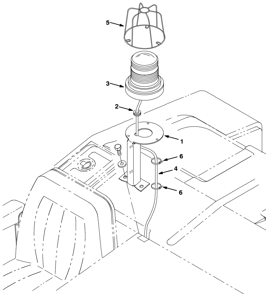
Fig. 70 - Flashing Light and Backup Alarm Group, LRC — Blinklicht - und Rückfahr-Alarm-Gruppe, LRC — Jeu de pièces alarme de sécurité et gyrophare, côtés droit et gauche
