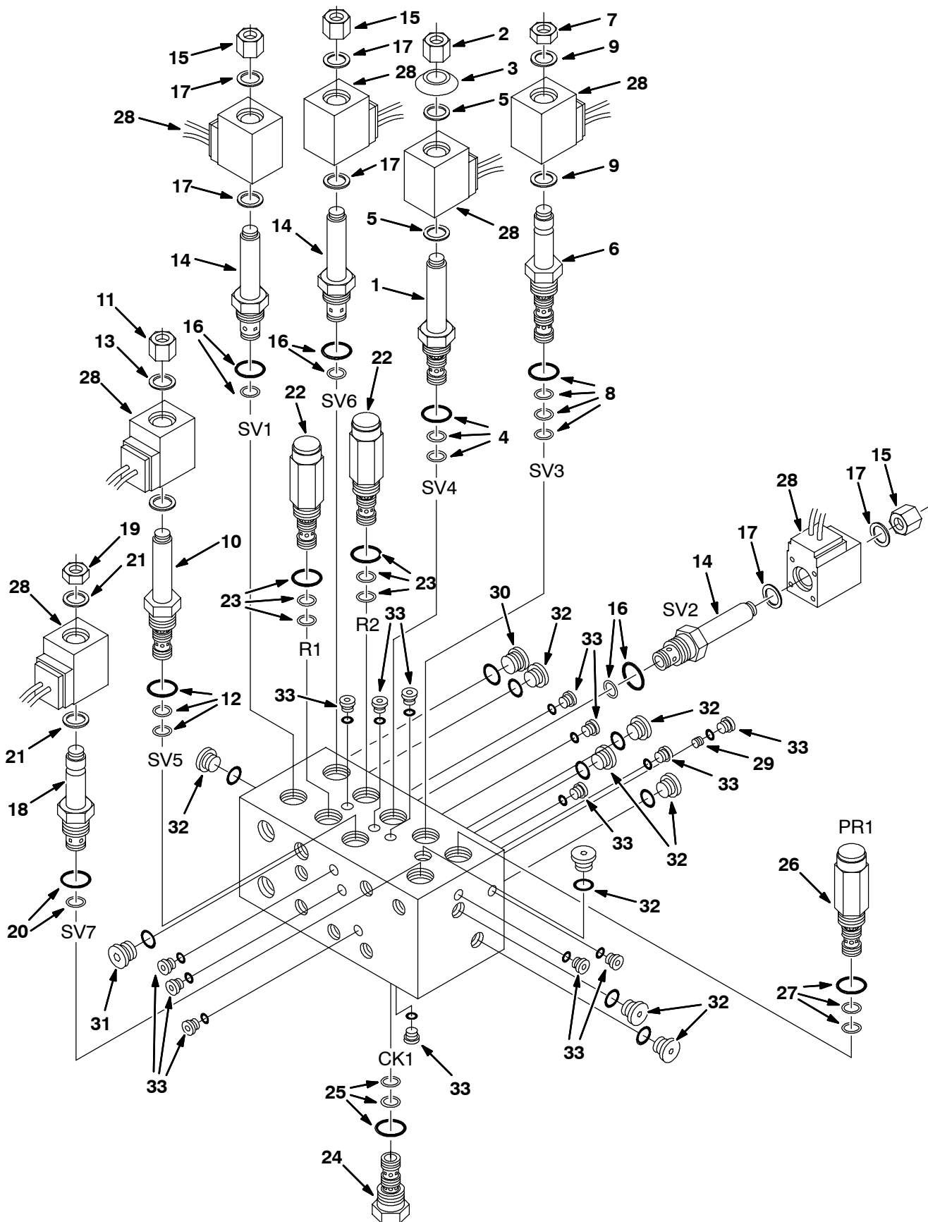
Fig. 15 - Hydraulic Solenoid Valve Breakdown, Side Brush and Nylon Brush, 71762 - Hydraulik-Magnetventil-Defekt, Seitenbürste und Nylon-Bürste - Panne de soupape magnétique hydraulique, brosse latérale et brosse en nylon, 71762
