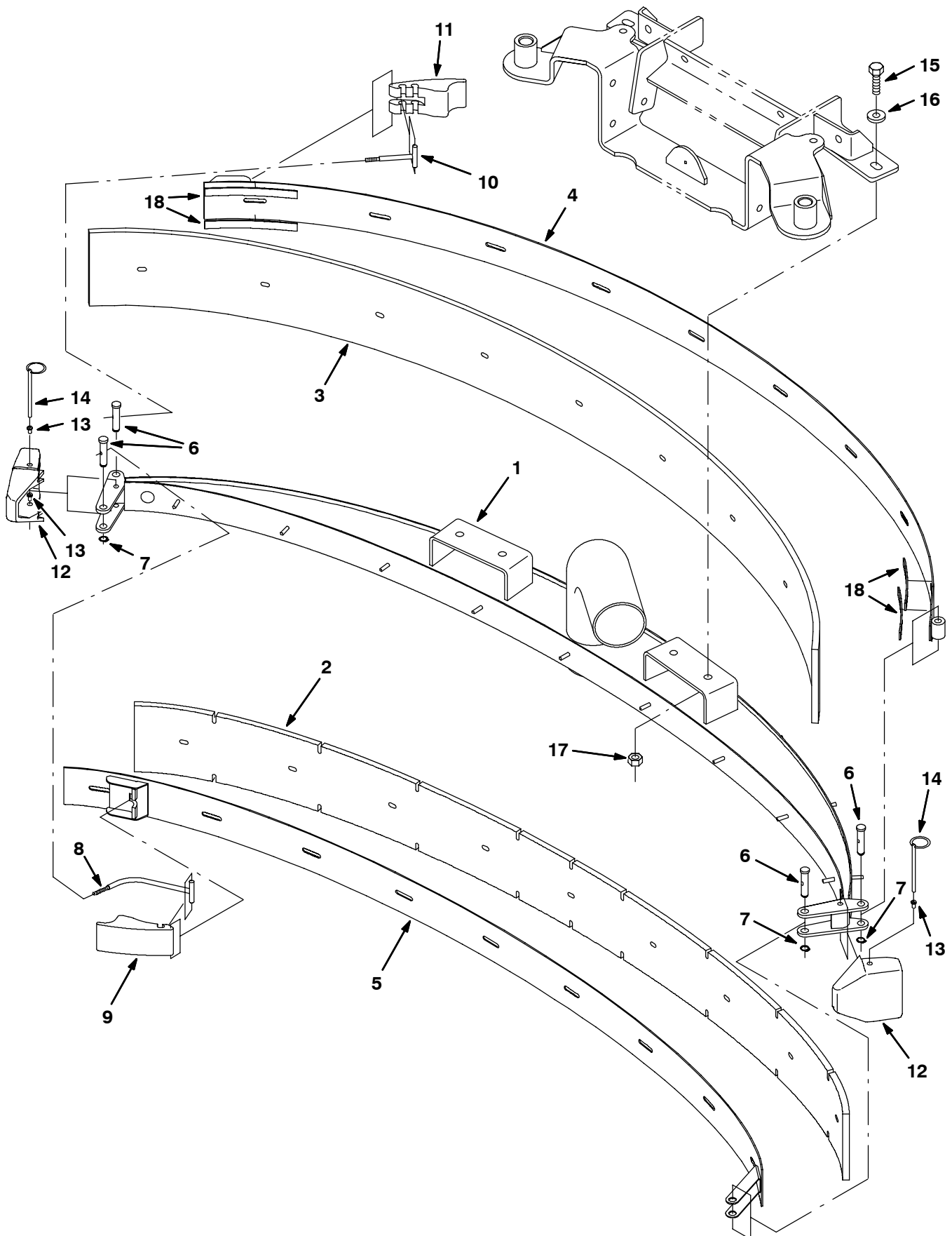
Fig. 53 - Rear Squeegee Assembly - Heck-Abstreifleisten-Baugruppe - Assemblage racloir arrière
