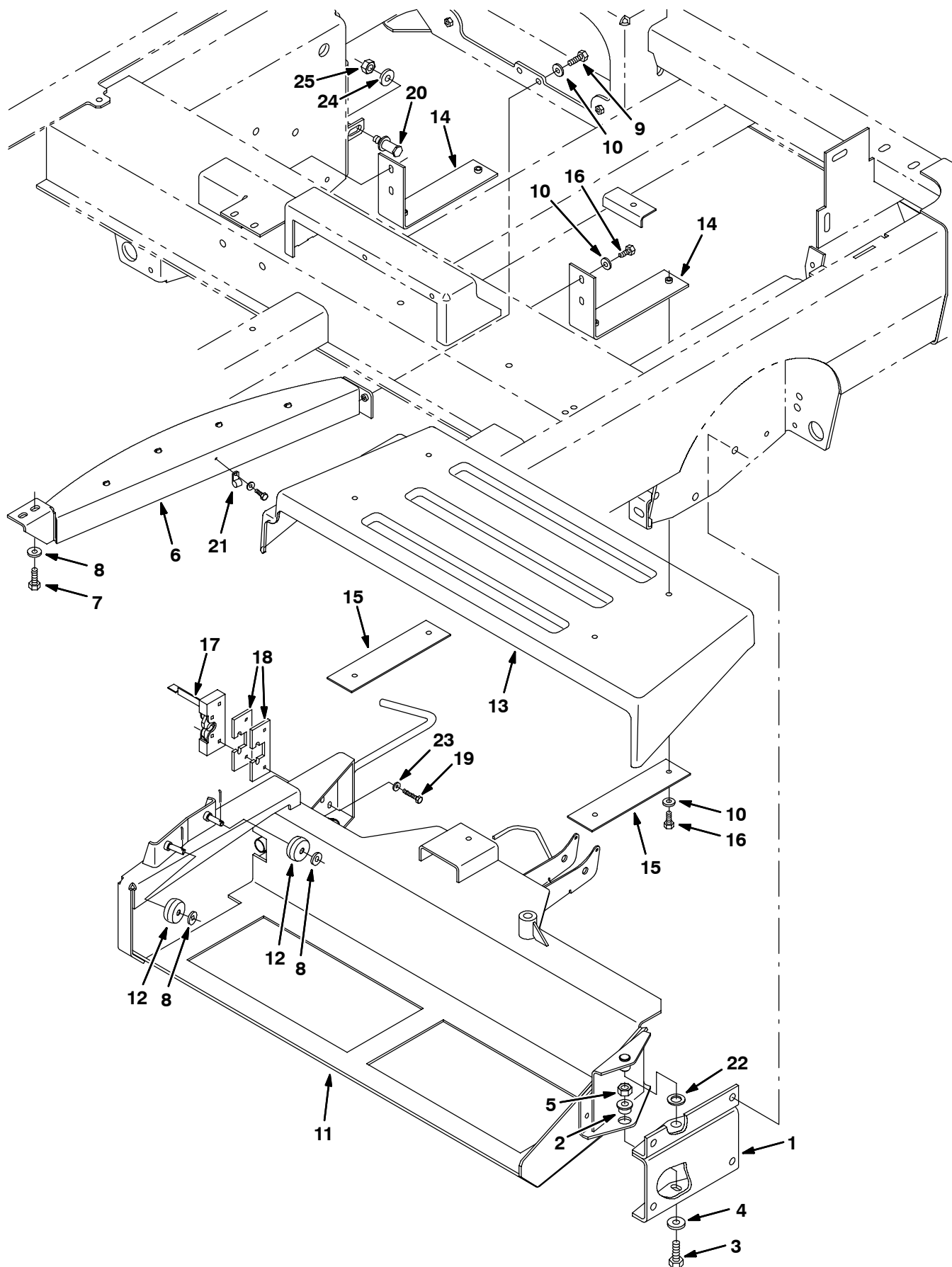
Fig. 49 - Debris Tray Frame Group - Schmutzkassette-Rahmen-Gruppe - Assemblage cadre du plateau à détrit
