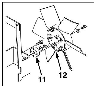
Fig. 20 - Cooling Fan and Housing Group - Kühlgebläse-/Gehäuse-Gruppe - Assemblage ventilateur et logement
