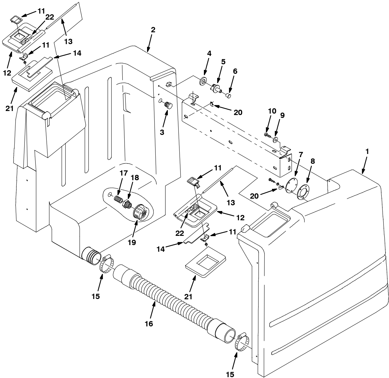
Fig. 29 - FaST Solution Tank Group - FaST-Frischwasser-Tankgruppe - Assemblage réservoir de solution FaST
