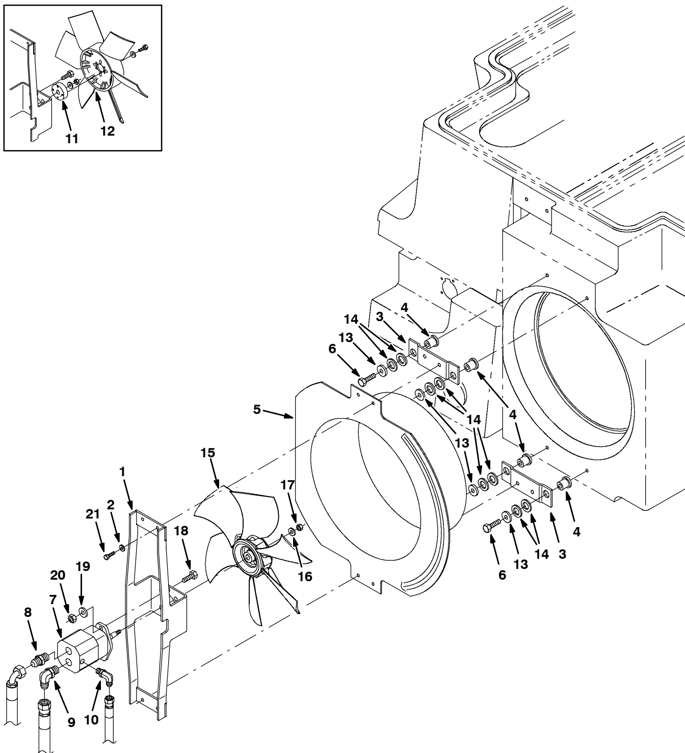
Fig. 20 - Cooling Fan and Housing Group - Kühlgebläse-/Gehäuse-Gruppe - Assemblage ventilateur et logement
