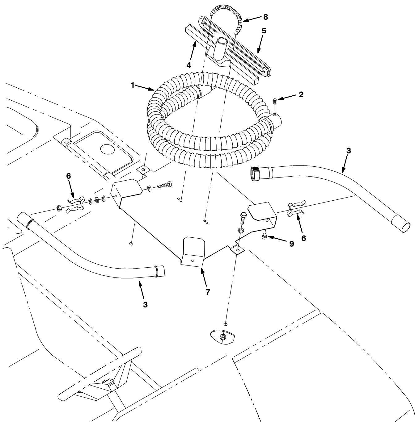
Fig. 15 - Squeegee Wand Kit - Hand-Abstreifleisten-Satz - Jeu de pièces manche à racloir
