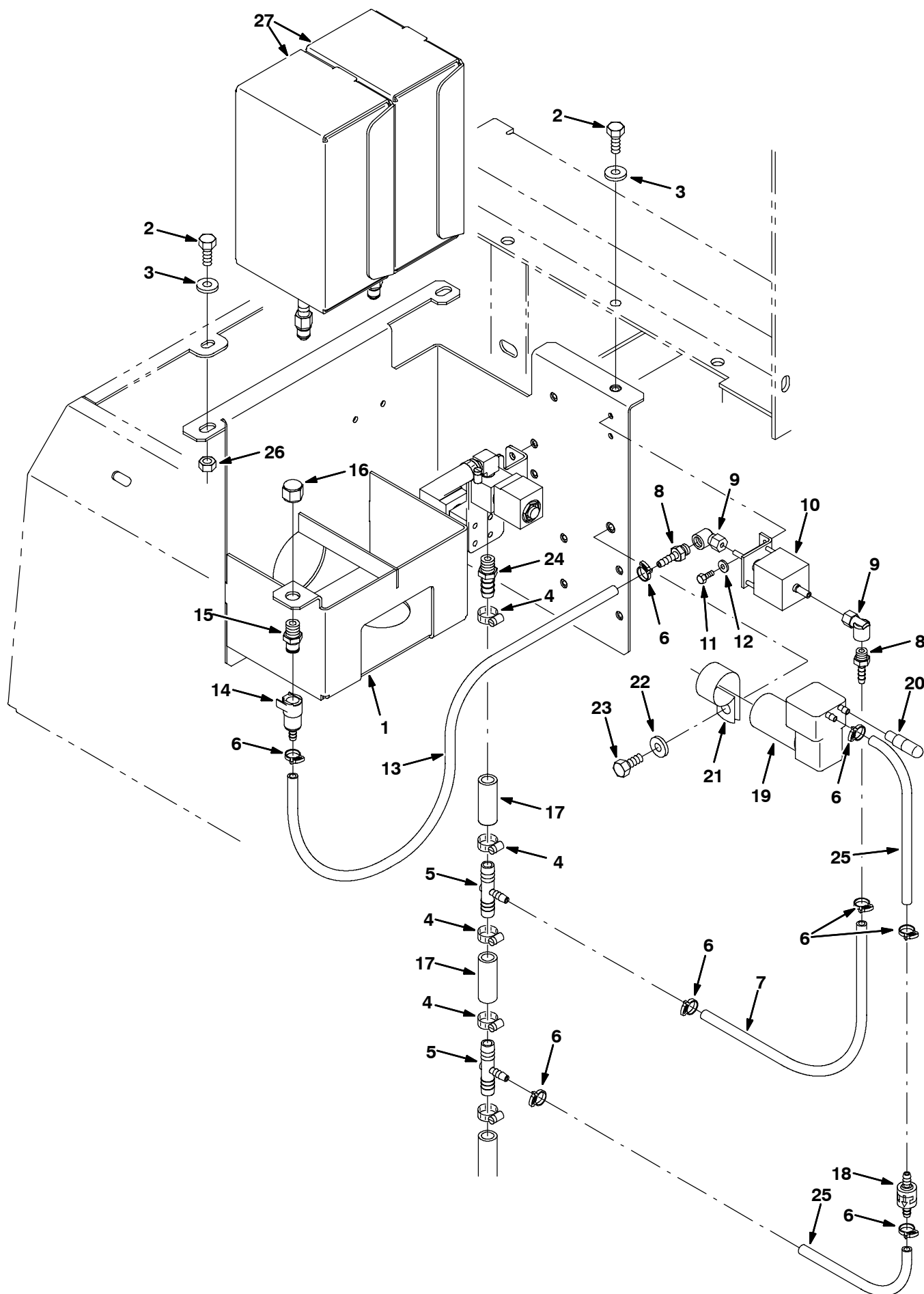
Fig. 66 - FaST Air Pump and Detergent Group — FaST Luftfilter - und Reinigungsmittel-Einheit — Groupe détergent et pompe à air FaST
