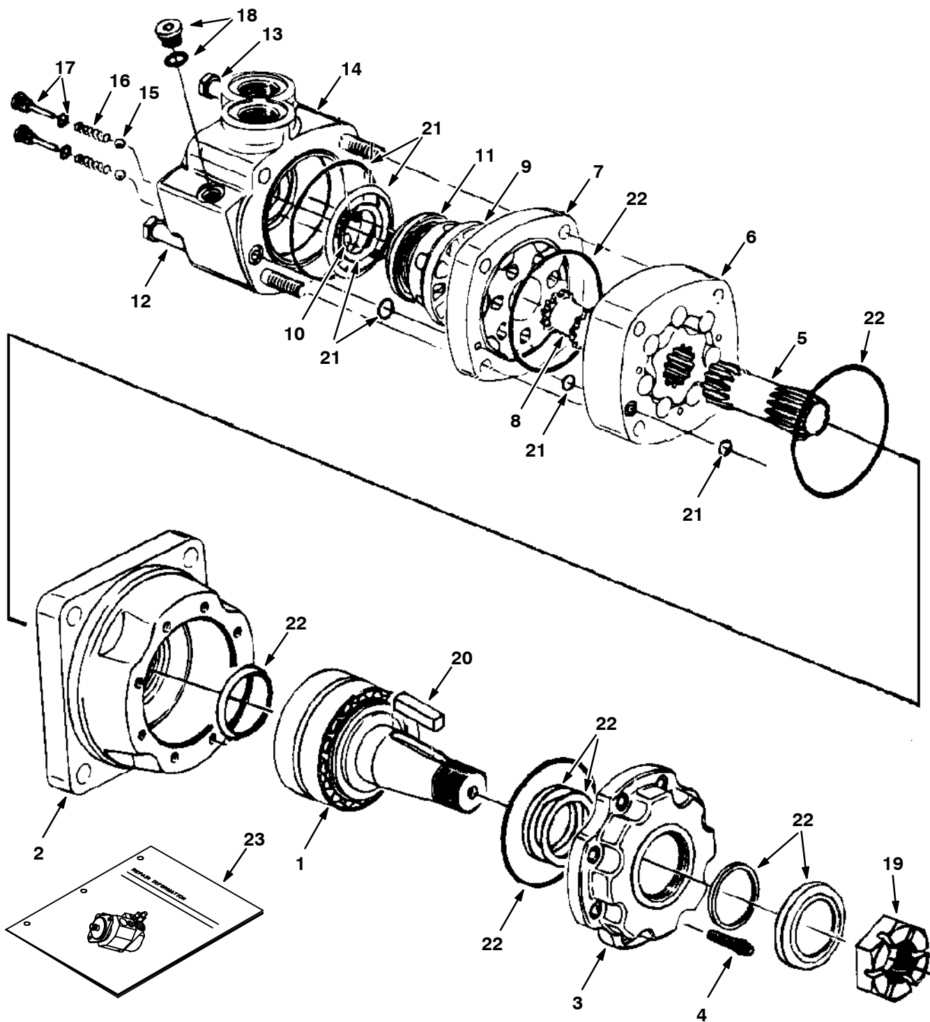
Fig. 4 - Hydraulic Motor Breakdown, 22604 - Hydraulik-Motor-Defekt - Panne de moteur hydraulique, 22604
