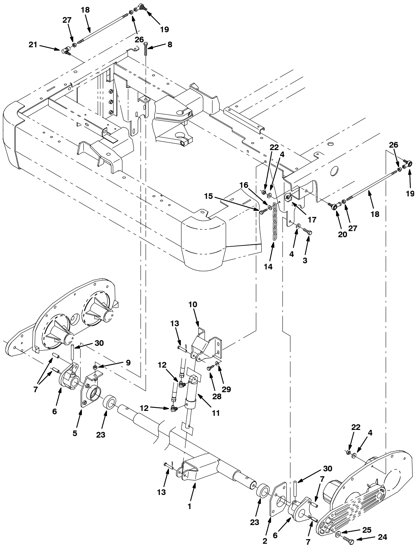
Fig. 43 - Scrub Head Lift Group - Schrubbkopf-Hebe-Gruppe - Assemblage système de levage de la tête de nettoyage
