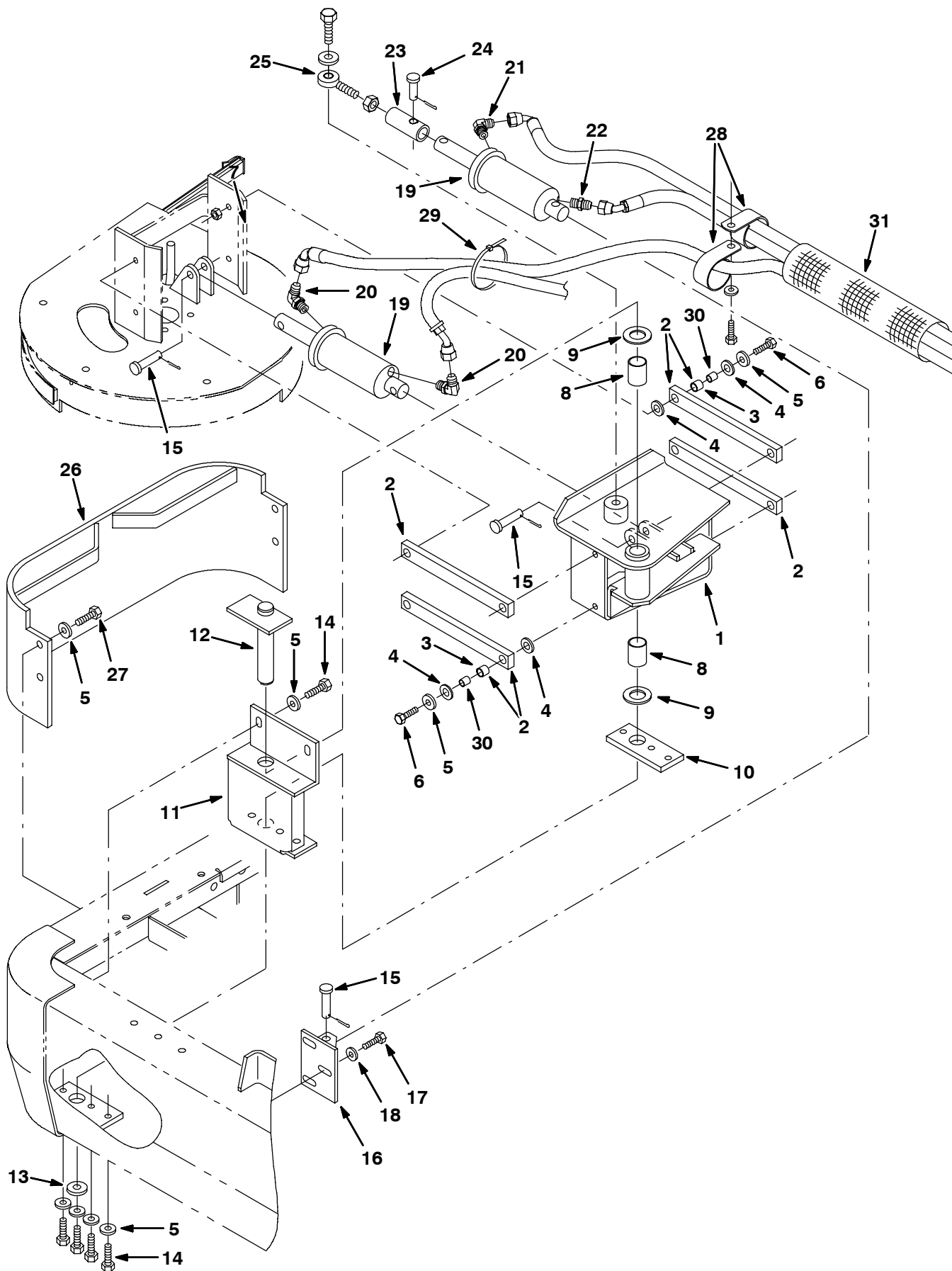
Fig. 59 - Side Brush Mount Group - Seitenbürsten-Montagegruppe - Assemblage attaches de la brosse latérale
