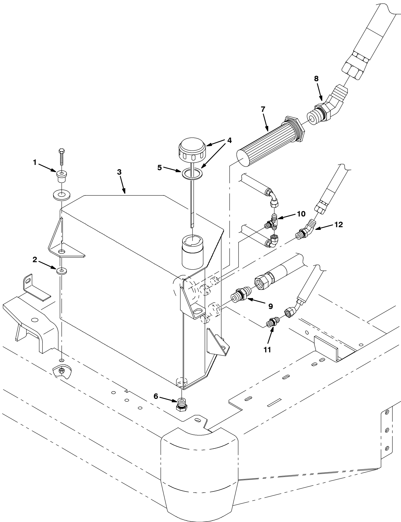
Fig. 38 - Hydraulic Reservoir Group - Hydraulik-Behältergruppe - Assemblage réservoir hydraulique
