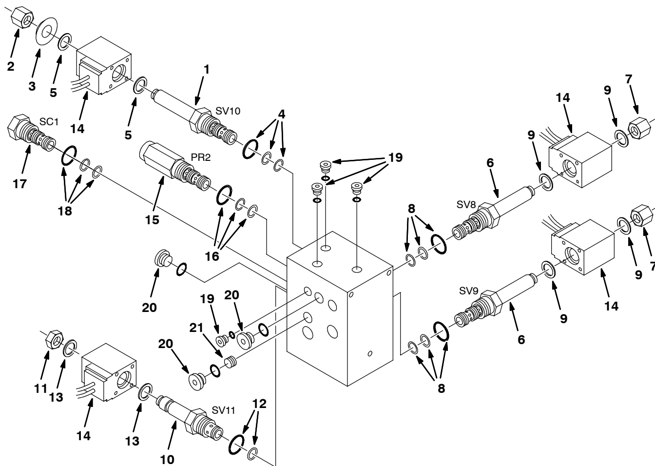
Fig. 16 - Hydraulic Solenoid Valve Breakdown, 71708 - Hydraulik-Magnetventil-Defekt - Panne de soupape magnétique hydraulique, 71708
