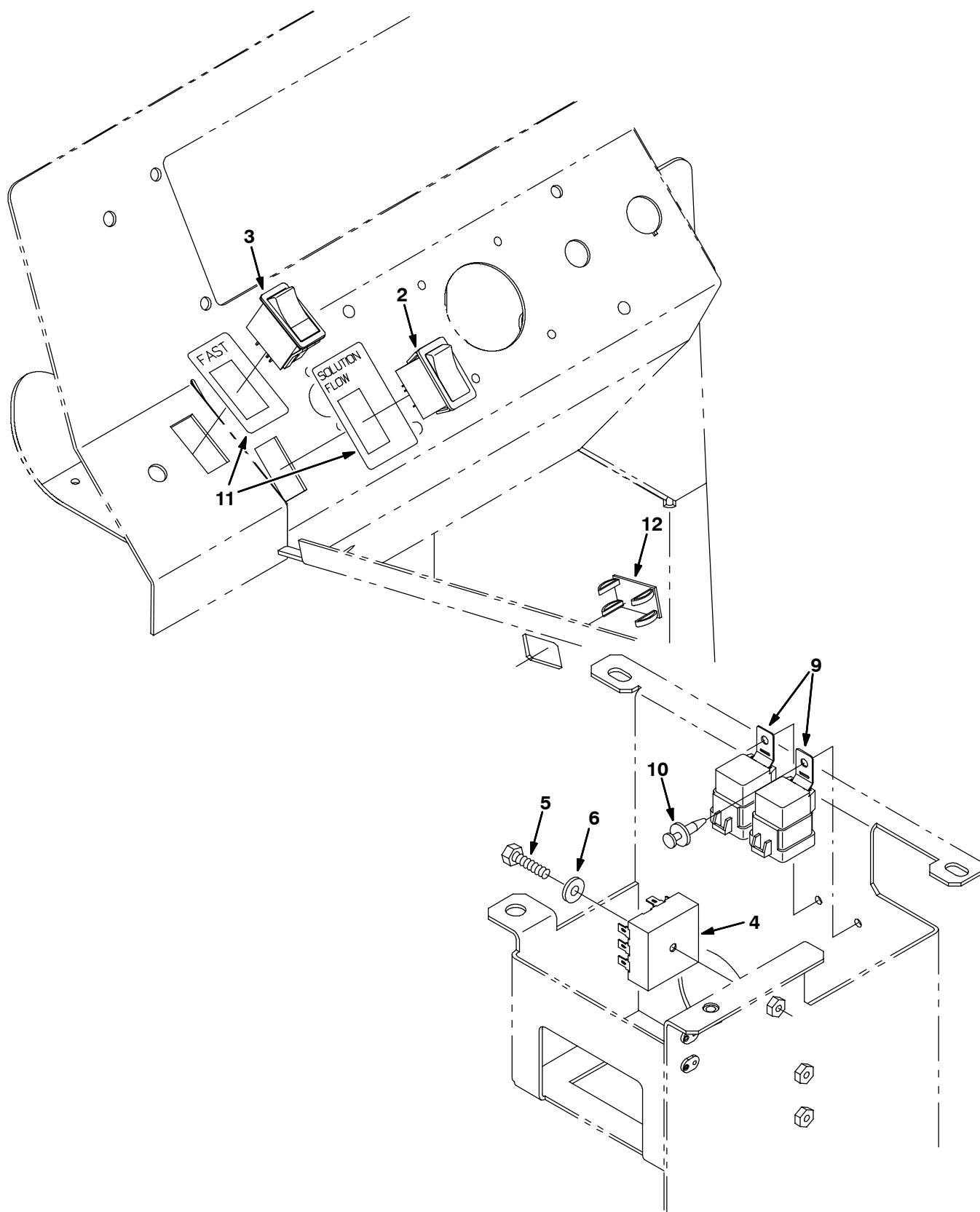
Fig. 69 - FaST Electrical Group — FaST Elektriksatz — Groupe électrique FaST
