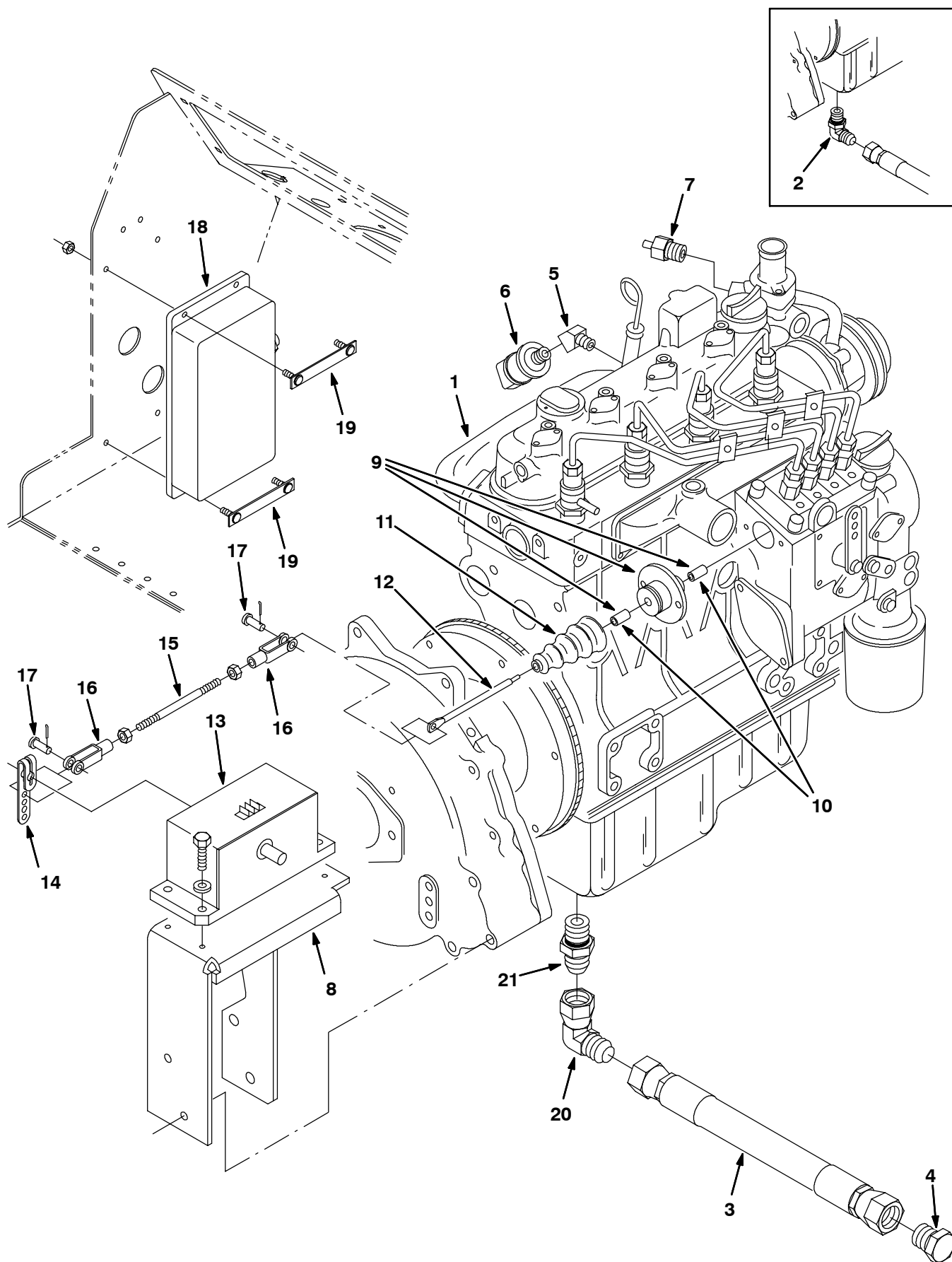
Fig. 12 - Engine and Governor Group (7400 001-7400 0500) - DieselMotor und Regler Gruppe - Groupe du moteur et régulateur
